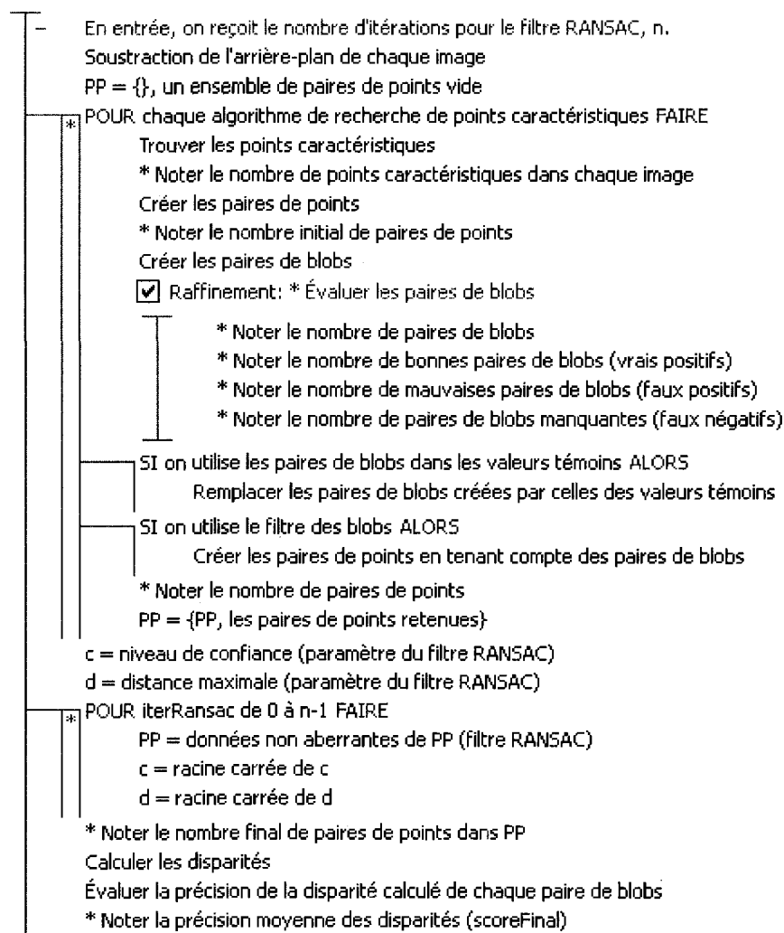
Figure 3.4 Pseudo-code schématique du calcul et des tests effectués. Les mesures sont identifiées par une étoile (*) au début de la ligne de description
