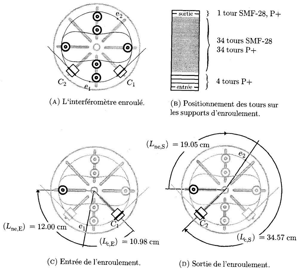
FIG. 2.9 – Détails de l'enroulement pour l'interféromètre de 100 Mbit/sec.
