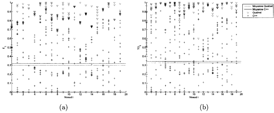
FIGURE 4.11 Impact du trafic à 5 paquets/s, sur Pr(E_{ij}) , (a), et Pr(TO_{ij}) , (b).
