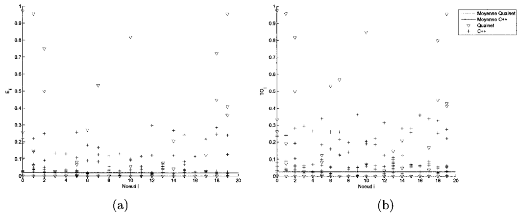
FIGURE 4.13 Impact de la distance, terrain carré de 0,16km^2 , sur \Pr(E_{ij}) , (a), et \Pr(TO_{ij}) , (b).
