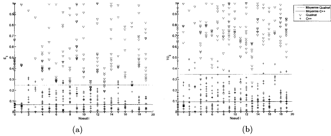
FIGURE 4.10 Impact du trafic à 0,5 paquet/s sur \Pr(E_{ij}) , (a) et \Pr(TO_{ij}) , (b).
