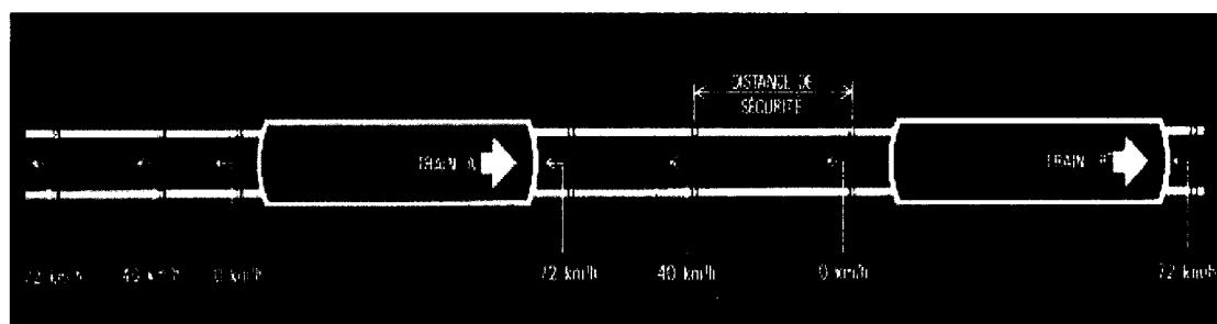
Figure 2-8 : Consignes de vitesse des cantons selon la position des trains. Source : (Communauté urbaine de Montréal et al. , 1983)
