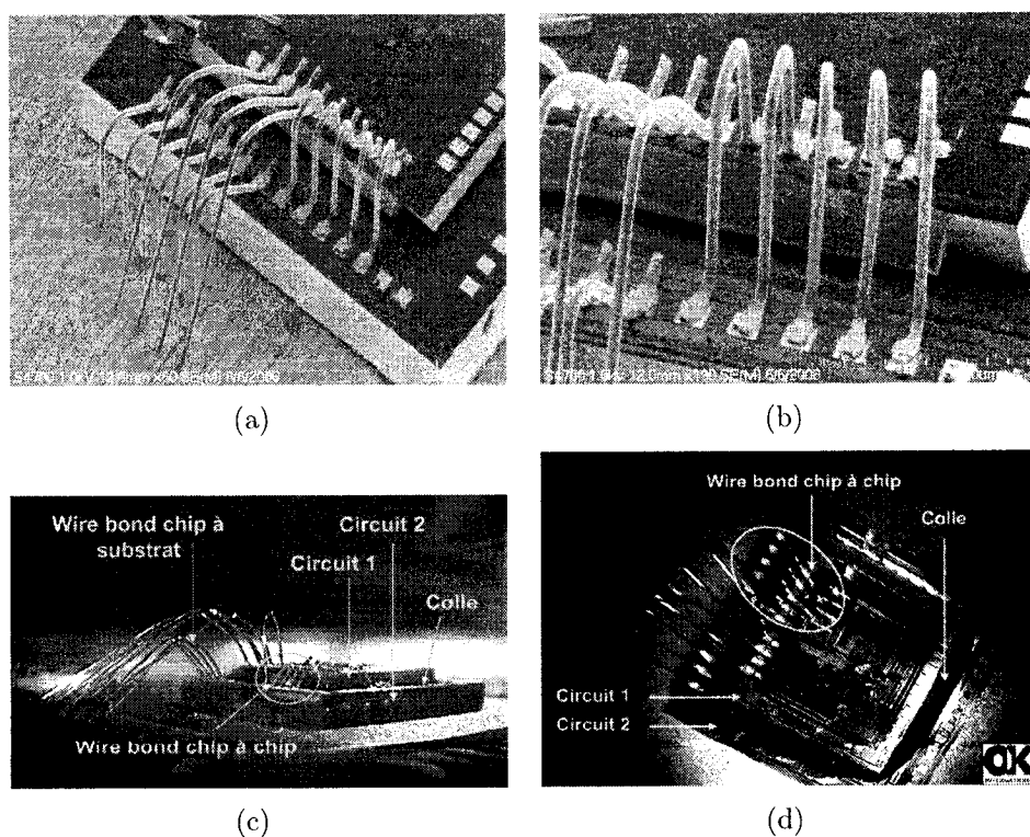
FIG. 4.25: Démonstration de connexions entre deux circuits disposés verticalement : a) Vue de côté, b) Agrandissement des connexions, c) Vue latérale avec identifications, d) Vue de haut avec identifications
