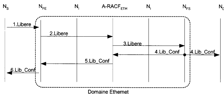
Figure 3.7 Libération bidirectionnelle de ressources dans un réseau Ethernet
