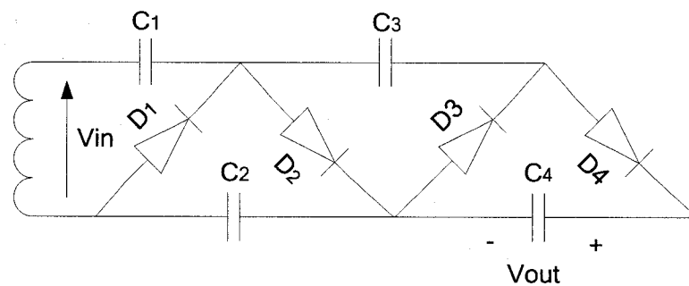
Figure 2.6. Schématique du multiplicateur de tension à demi onde (half wave multiplier).
