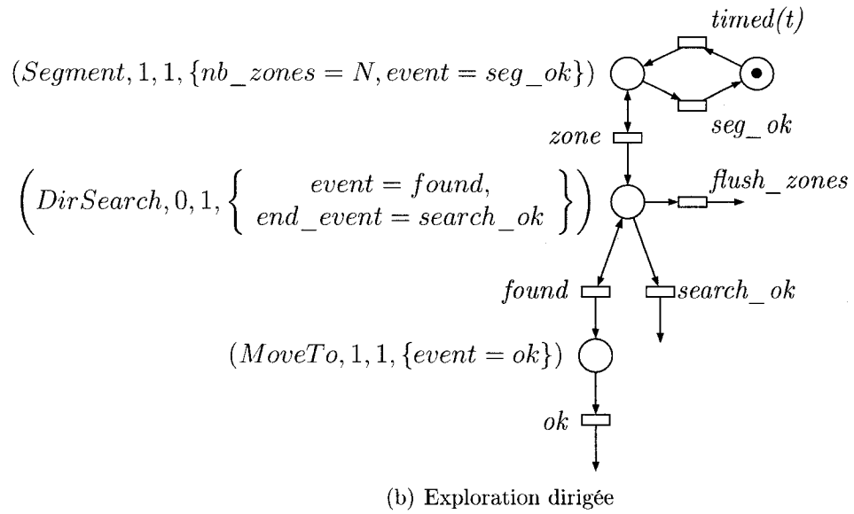
FIG. 4.2 – Réseaux de Pétri associés à la mission de Search-and-Rescue
