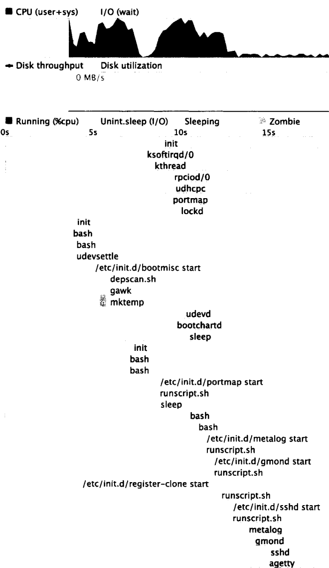
Figure 4.9 Profilage du démarrage d'un clone sans mémoire d'état
