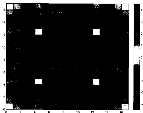
Figure 3.41 Écarts des taux d'absorption rapide en début de cycle (%)
