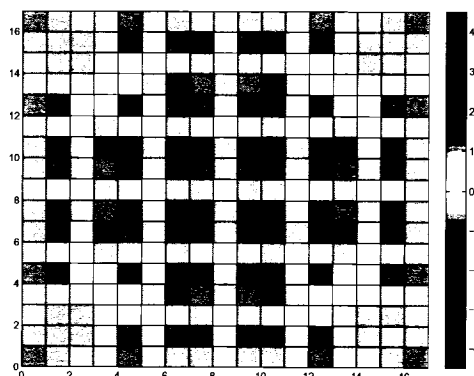
Figure 3.40 Écarts des taux de production thermique en fin de cycle (%)
