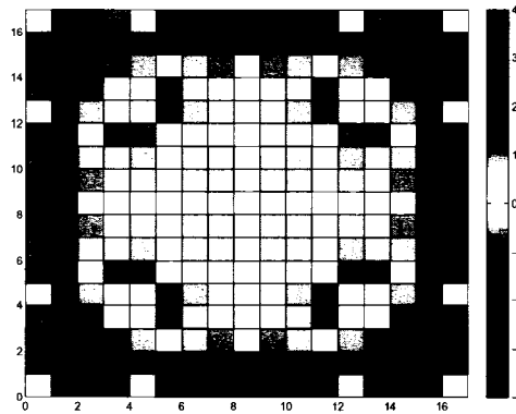
Figure 3.17 Carte des écarts relatifs des taux de fission entre le regroupement 3 et la référence (%)
