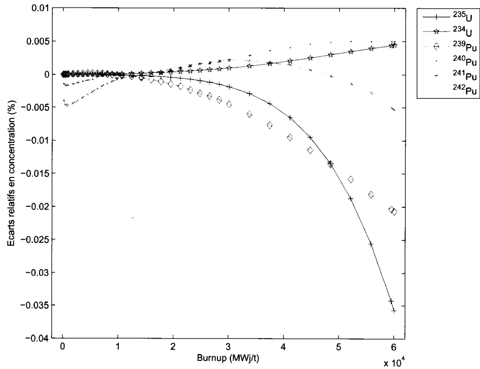
Figure 3.11 Écarts relatifs des concentrations entre le regroupement 3 et la référence
