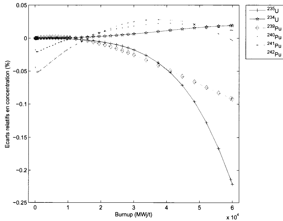
Figure 3.10 Écarts relatifs des concentrations entre le regroupement 1 et la référence
