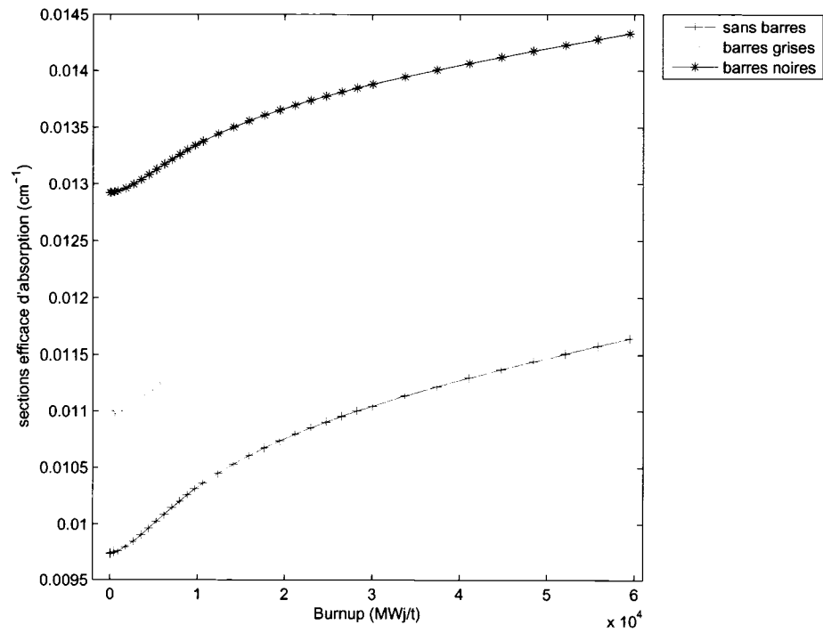
Figure 4.6 \Sigma_a groupe rapide
