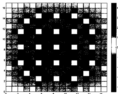
Figure 3.37 Écarts des taux de production rapide en début de cycle (%)
