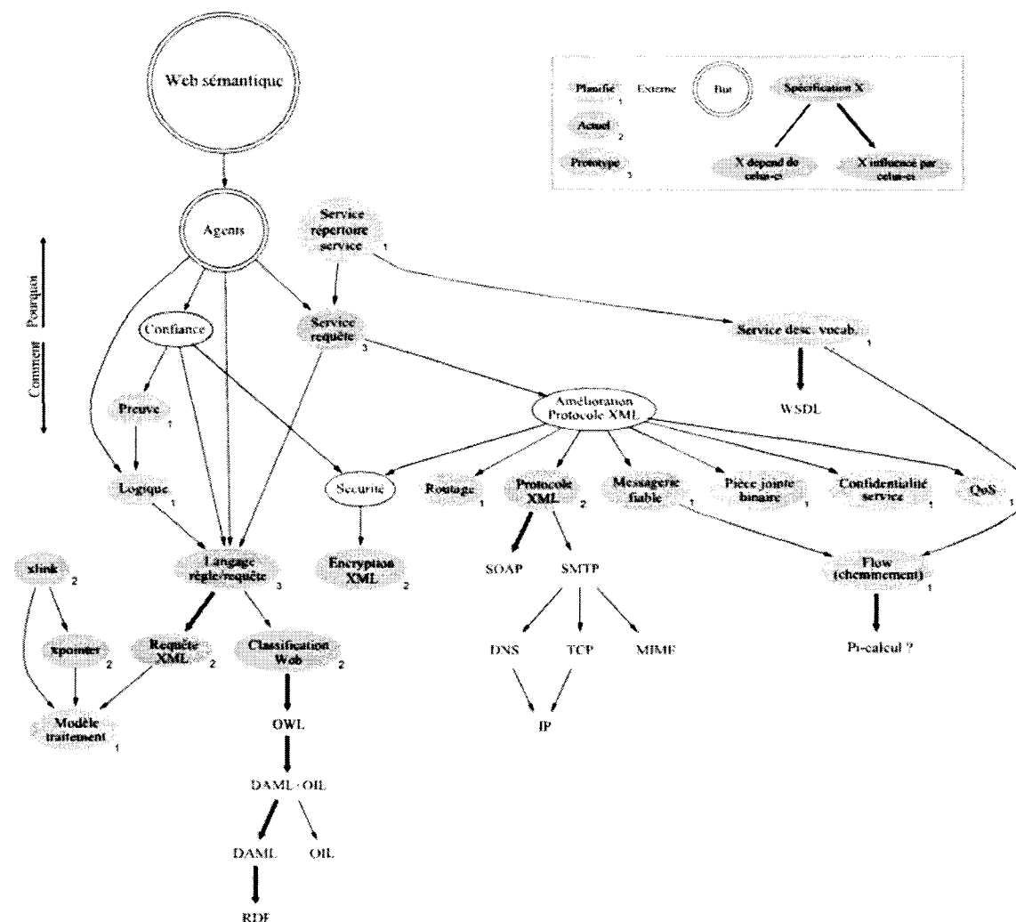
Figure 5-7 : Calendrier de lancement technologique du Web sémantique adapté à partir du calendrier officiel ( http://www.w3.org/2001/sw ).
