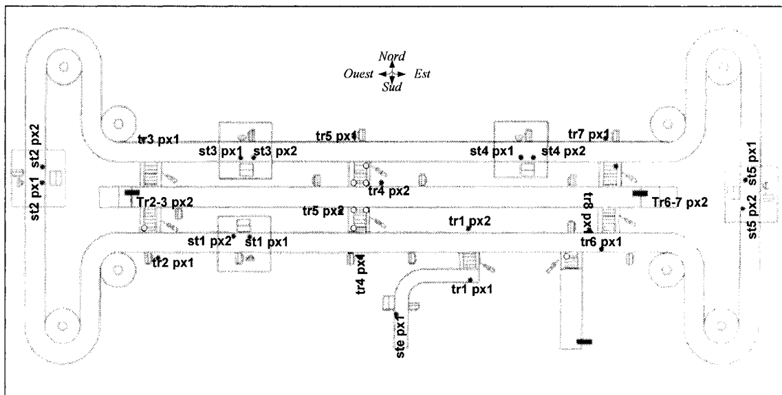
Figure 4. 2. Capteurs utilisés par le ST
