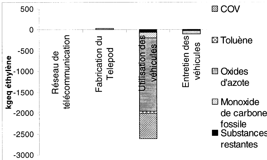
Figure 5.15 : Contribution des divers polluants à l'indicateur de catégorie formation d'ozone photochimique pour les différents processus impliqués dans l'ACV du Telepod.
