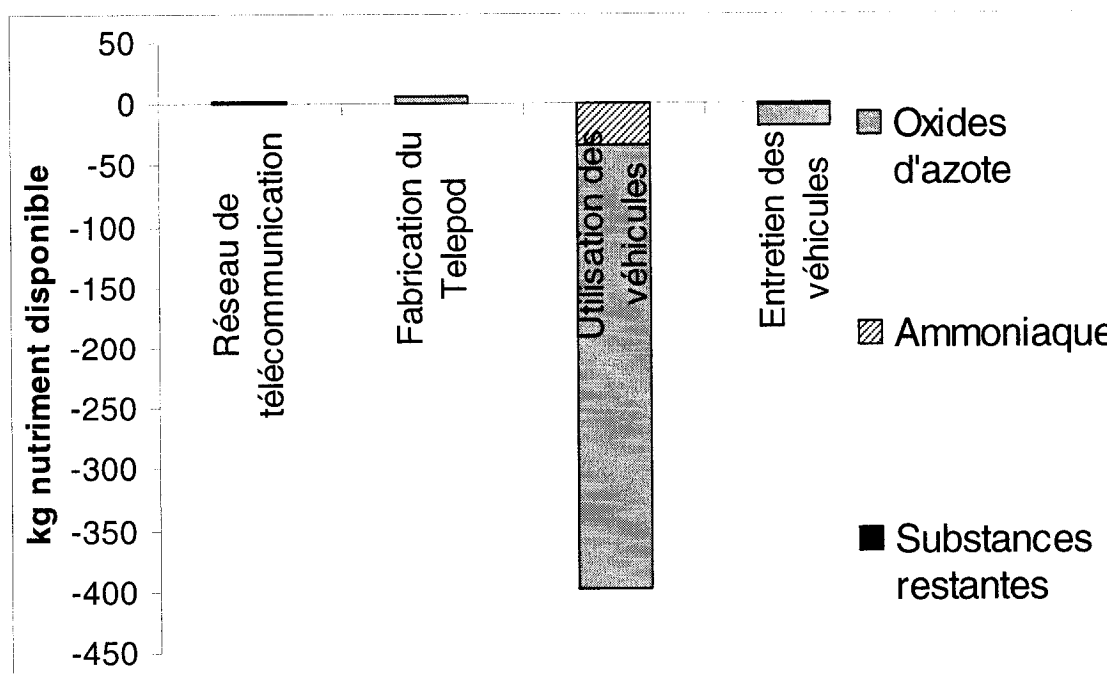
Figure 5.11 : Contribution des divers polluants à l'indicateur de catégorie de l'eutrophisation terrestre pour les différents processus impliqués dans l'ACV du Telepod.
