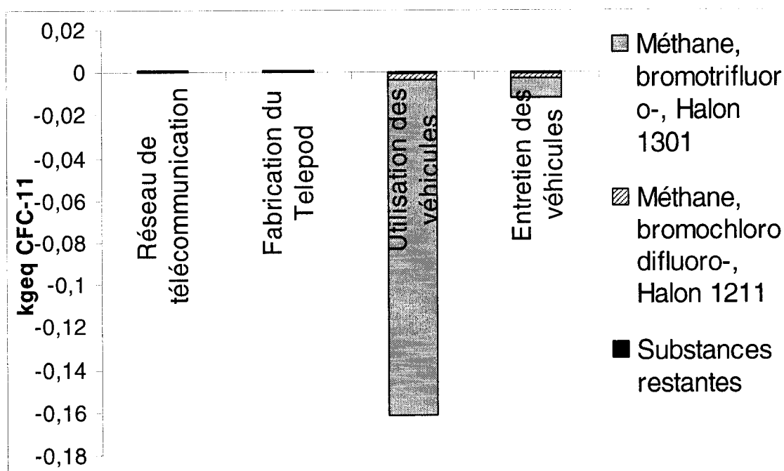
Figure 5.13 : Contribution des divers polluants à l'indicateur de catégorie de la déplétion de la couche d'ozone pour les différents processus impliqués dans l'ACV du Telepod.
