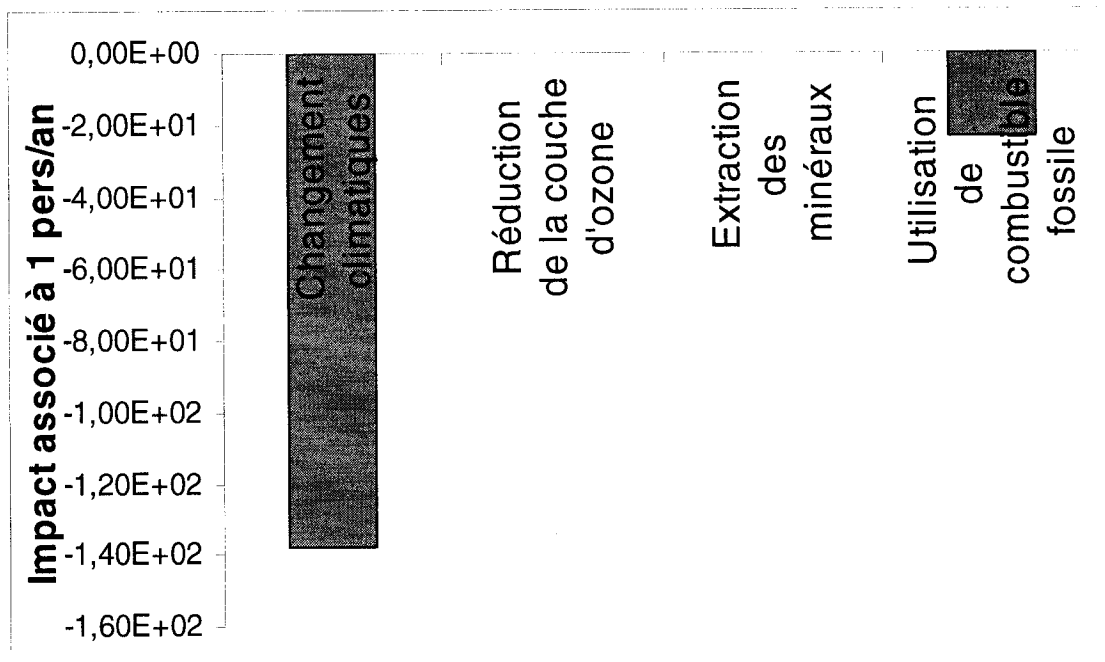
Figure 5.2 : Impacts totaux globaux normalisés associés à l'ACV Telepod.
