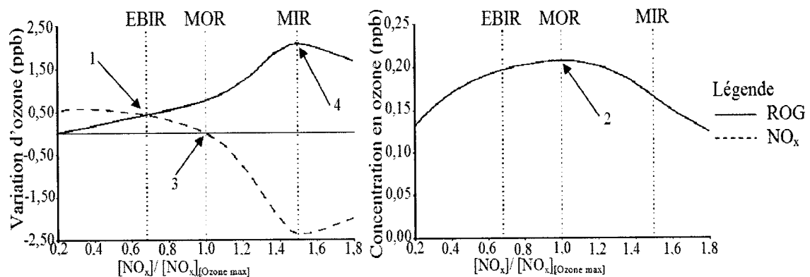
Figure 2.4 : Quantification de la dépendance du maximum d'ozone et du changement relatif en ozone causé par une augmentation de 1% du total de ROG et de NO x pour le scénario des conditions moyennes (Carter 1994).
