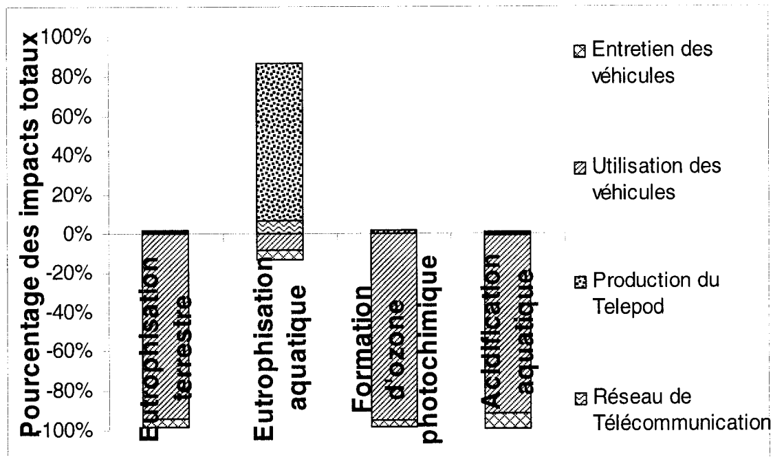
Figure 5.4 : Pourcentages des impacts totaux locaux associés à l'ACV Telepod normalisés sur une échelle de 100%.
