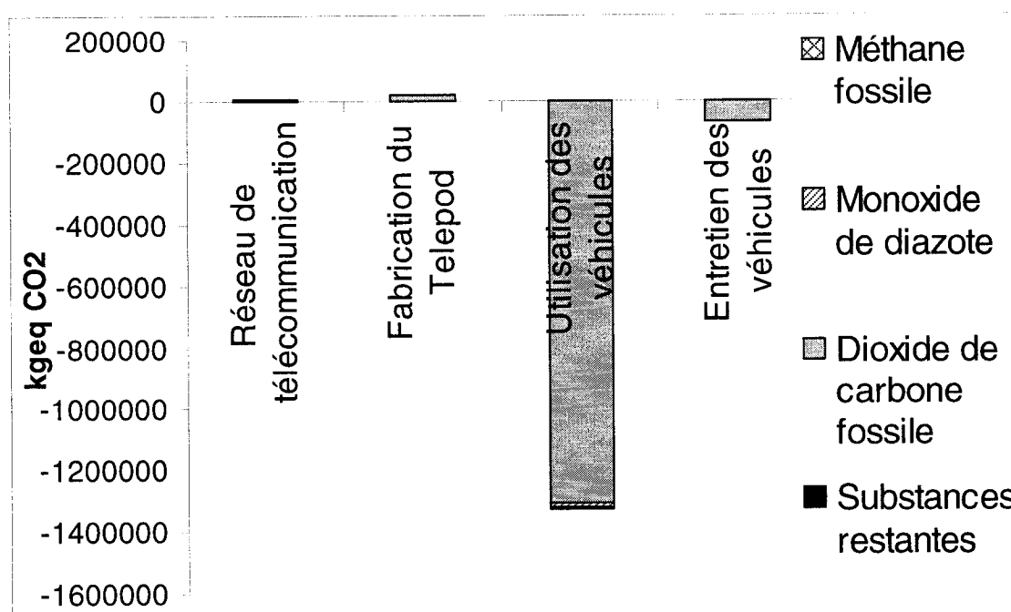
Figure 5.14 : Contribution des divers polluants à l'indicateur de catégorie du réchauffement climatique pour les différents processus impliqués dans l'ACV du Telepod.
