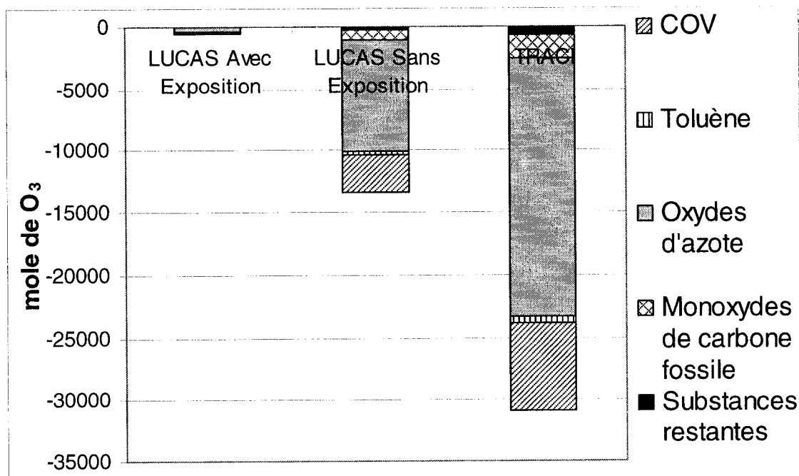
Figure 5.19 : Comparaison des indicateurs de catégories (étude de cas du Telepod) calculés avec les méthodes de LUCAS avec l'utilisation de l'exposition humaine, de LUCAS sans l'utilisation de l'exposition humaine et de TRACI pour la catégorie d'impact de la formation d'ozone photochimique.
