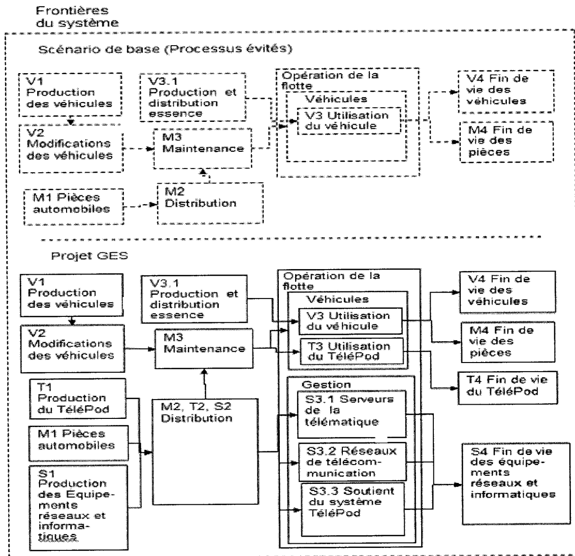
Figure 3.1 : Frontières initiales du système de produits pour le projet Telepod sur les GES (Charron-Doucet 2006).
