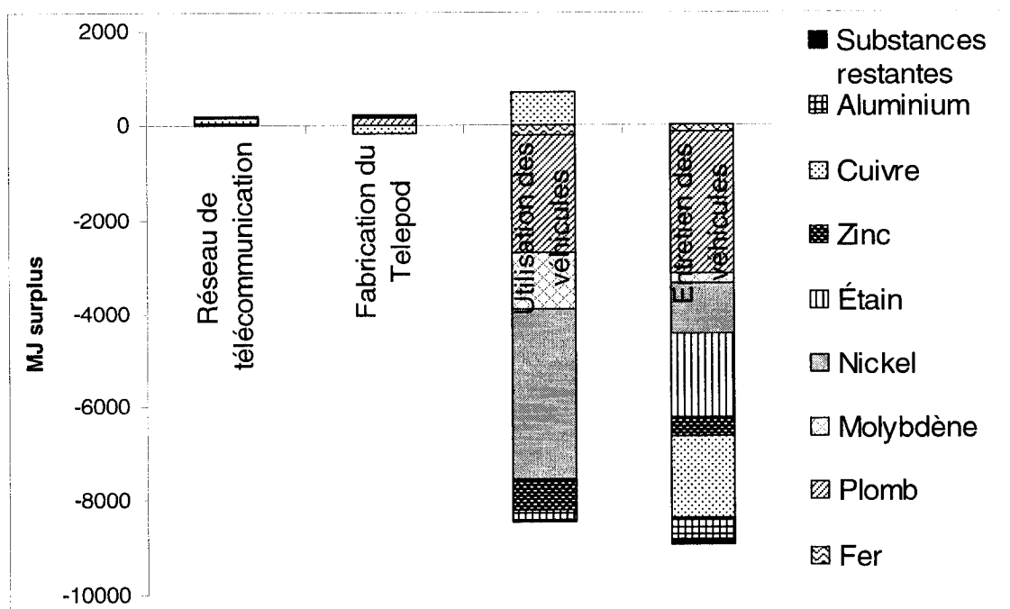
Figure 5.12 : Contribution des divers minéraux extraits à l'indicateur de catégorie de l'eutrophisation terrestre pour les différents processus impliqués dans l'ACV du Telepod.
