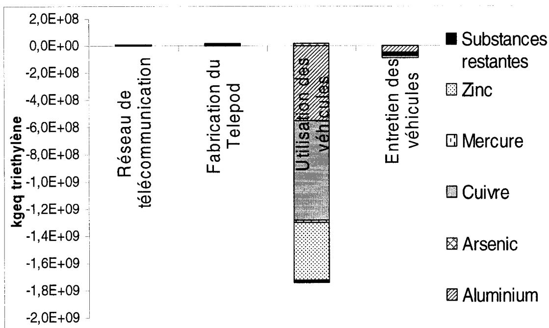
Figure 5.9 : Contribution des divers polluants à l'indicateur de catégorie de l'écotoxicité terrestre pour les différents processus impliqués dans l'ACV du Telepod.
