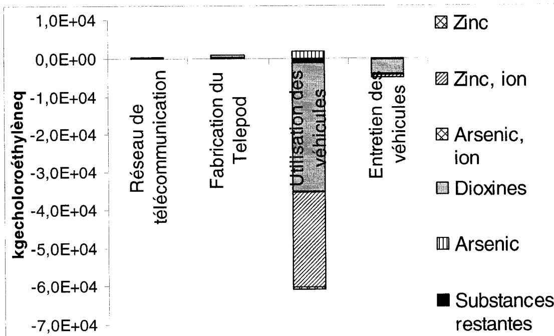
Figure 5.17 : Contribution des divers polluants à l'indicateur de catégorie de la toxicité autre que cancérogène pour les différents processus impliqués dans l'ACV du Telepod.
