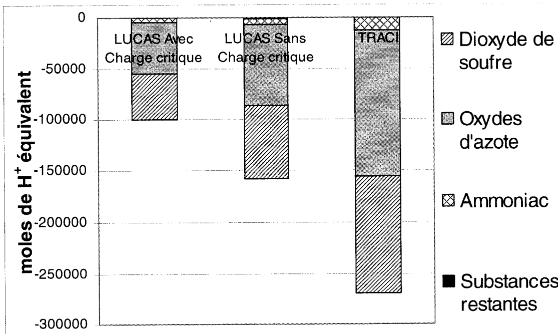
Figure 5.18 : Comparaison des indicateurs de catégories (étude de cas du Telepod) calculés avec les méthodes de LUCAS avec l'utilisation de la charge critique, de LUCAS sans l'utilisation de la charge critique et de TRACI pour la catégorie d'impact de l'acidification aquatique.
