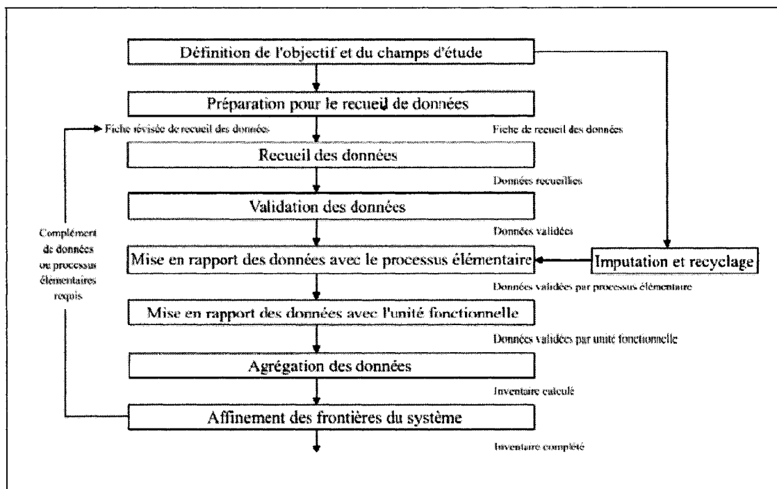
Figure 2.1 : Étapes opérationnelles composant une analyse d'inventaire selon ISO 14 041 (ISO 1998).
