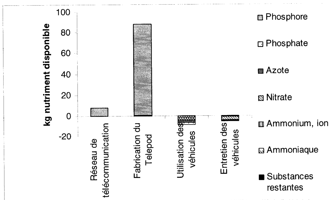
Figure 5.10 : Contribution des divers polluants à l'indicateur de catégorie de l'eutrophisation aquatique pour les différents processus impliqués dans l'ACV du Telepod.
