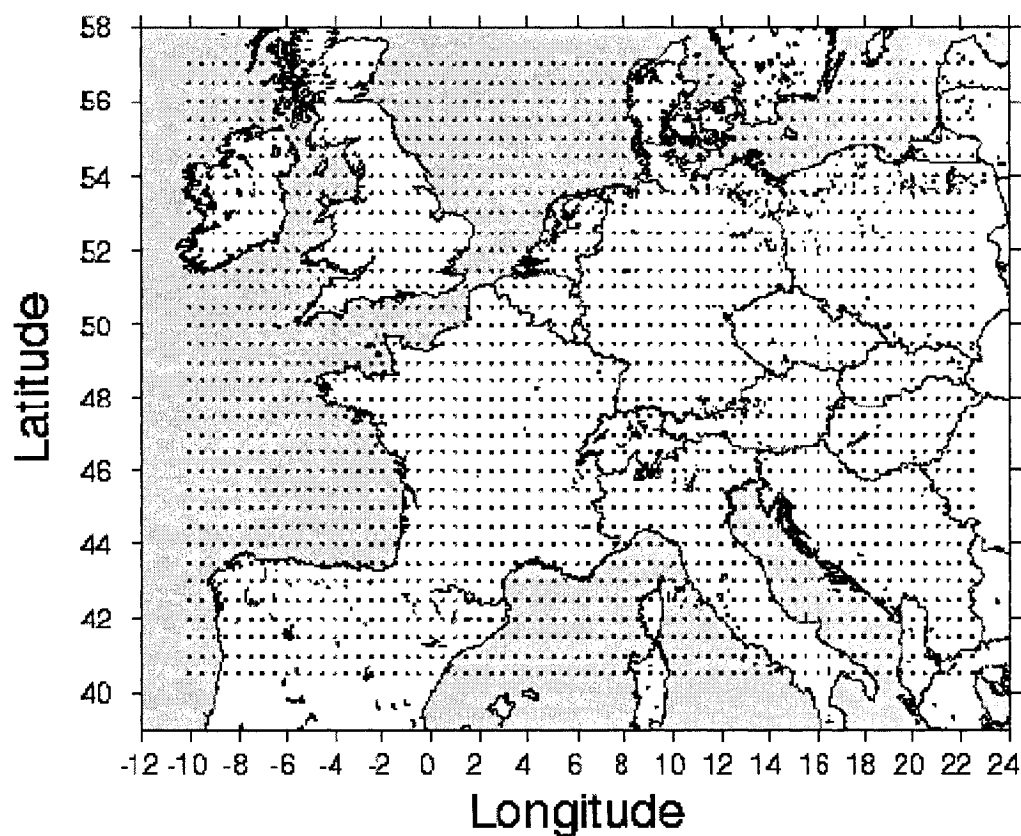
Figure 2.5 : Maillage typique utilisé dans les modèles de transport atmosphérique de polluants pour l'Europe : CHIMERE et RAINS. (Labouze, et al. 2004)
