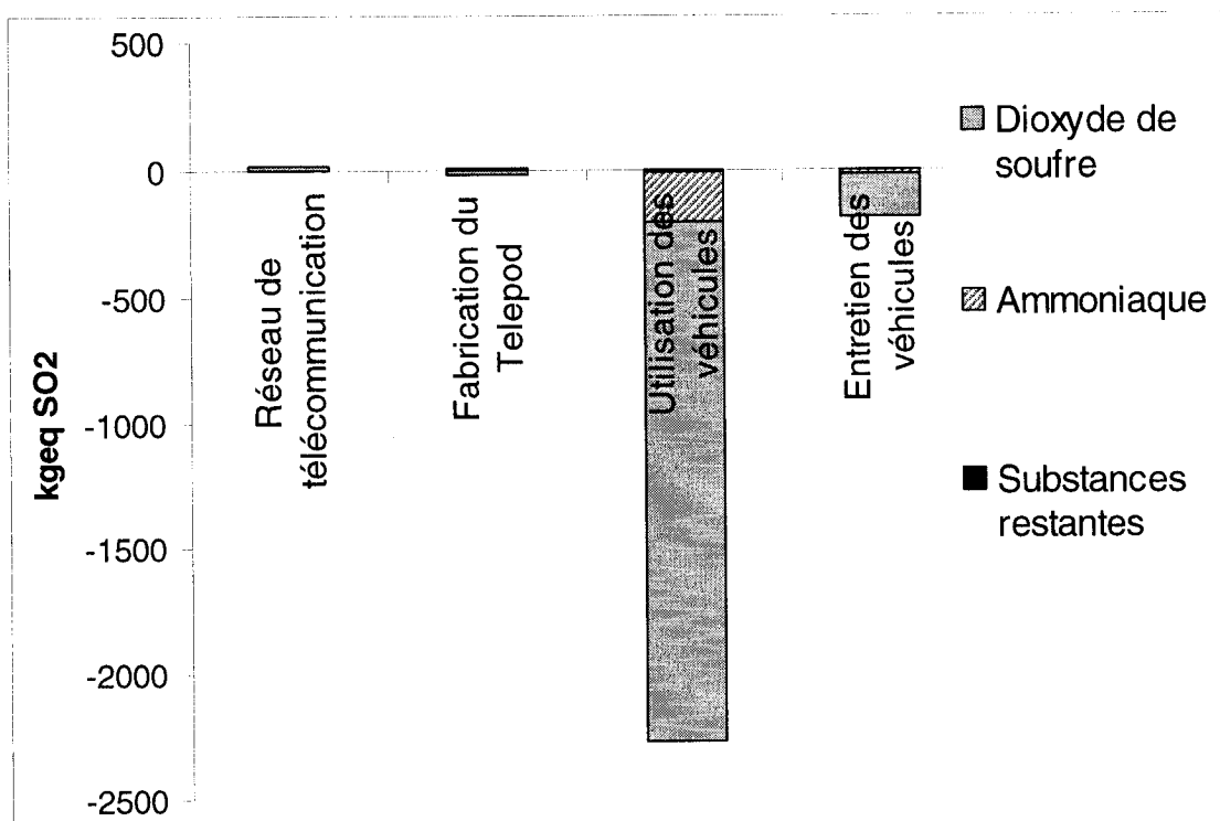
Figure 5.6 : Contribution des divers polluants à l'indicateur de catégorie de l'acidification aquatique pour les différents processus impliqués dans l'ACV du Telepod.
