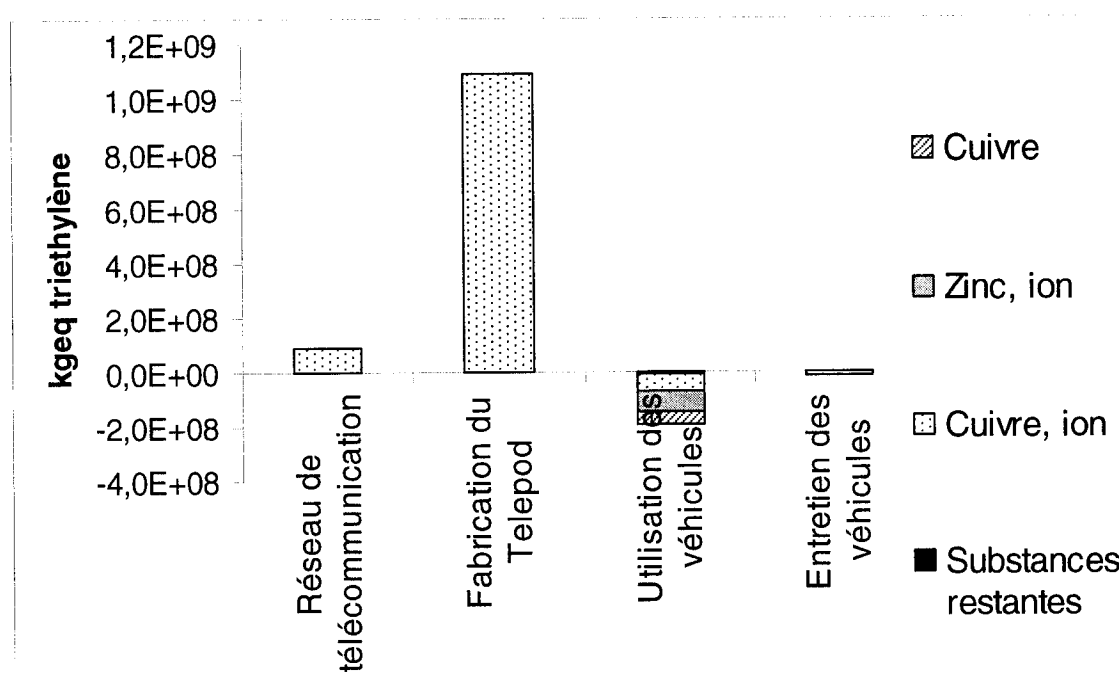
Figure 5.8 : Contribution des divers polluants à l'indicateur de catégorie de l'écotoxicité aquatique pour les différents processus impliqués dans l'ACV du Telepod.
