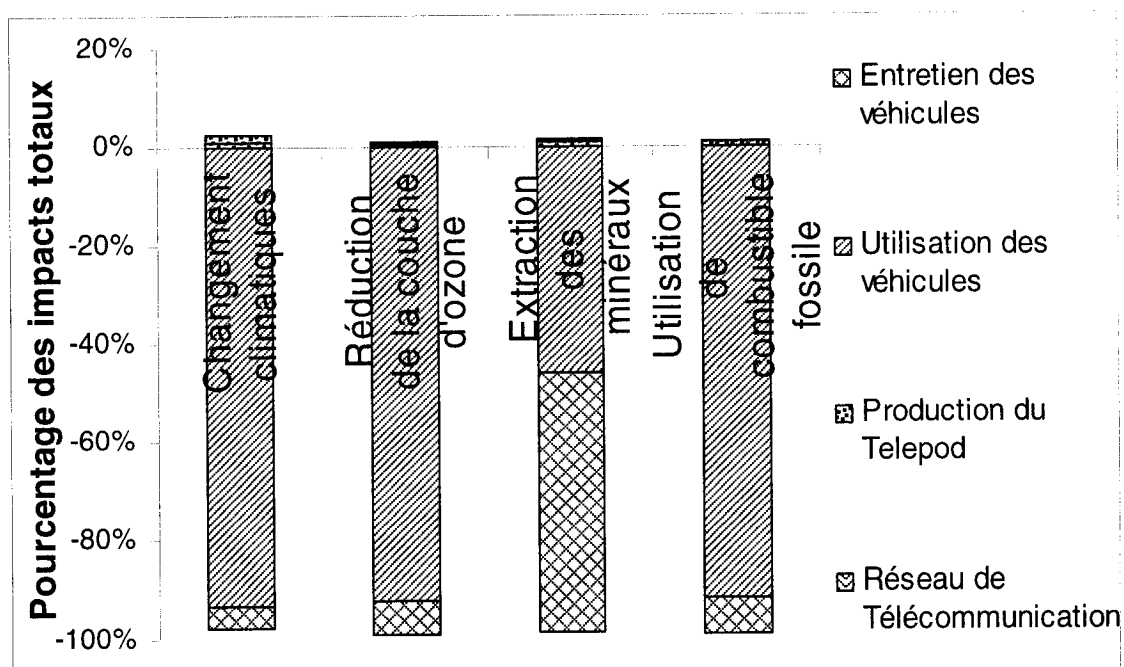
Figure 5.1 : Pourcentages des impacts totaux globaux associés à l'ACV Telepod normalisés sur une échelle de 100%.
