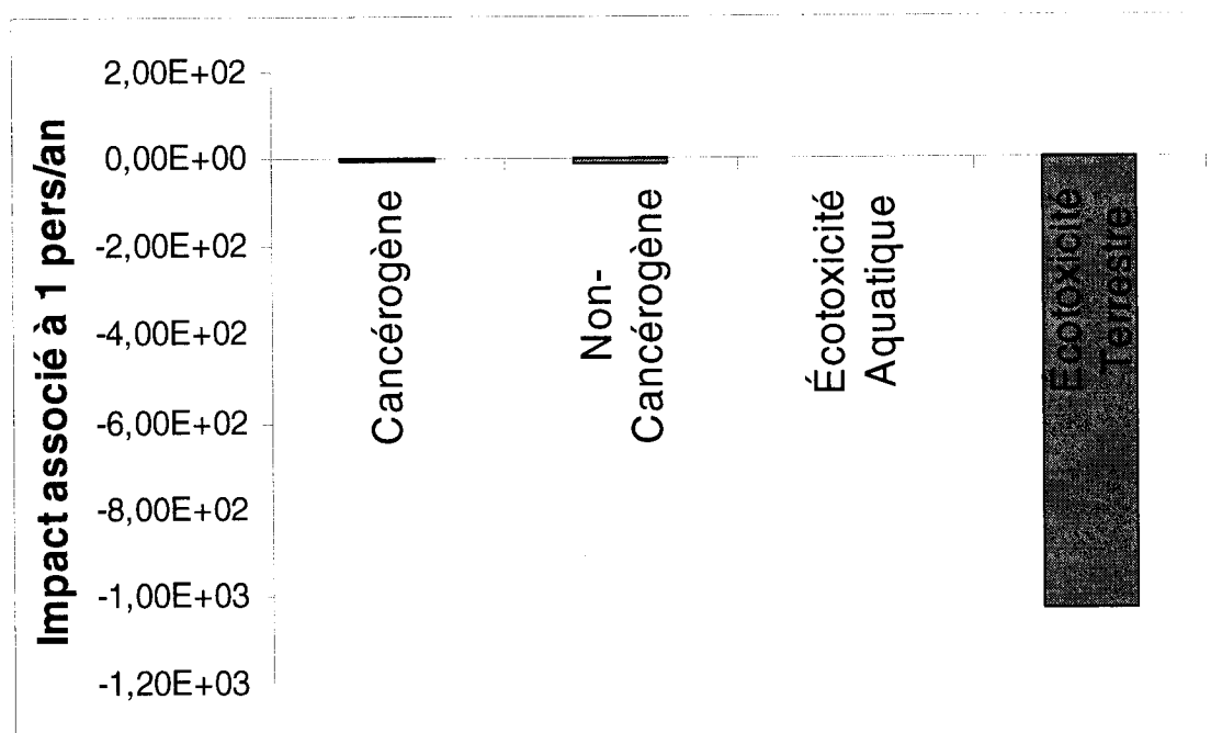
Figure 5.5 : Impacts totaux locaux normalisés associés à l'ACV Telepod.
