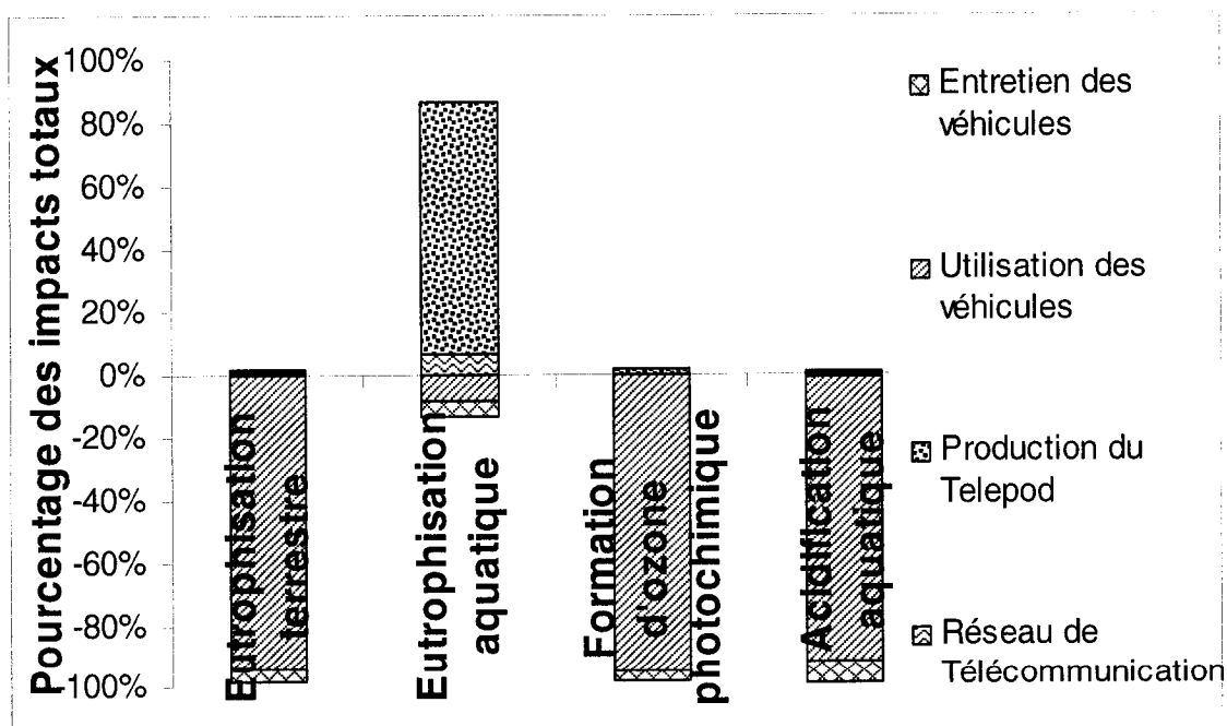
Figure 5.3 : Pourcentages des impacts totaux régionaux associés à l'ACV Telepod normalisés sur une échelle de 100%.
