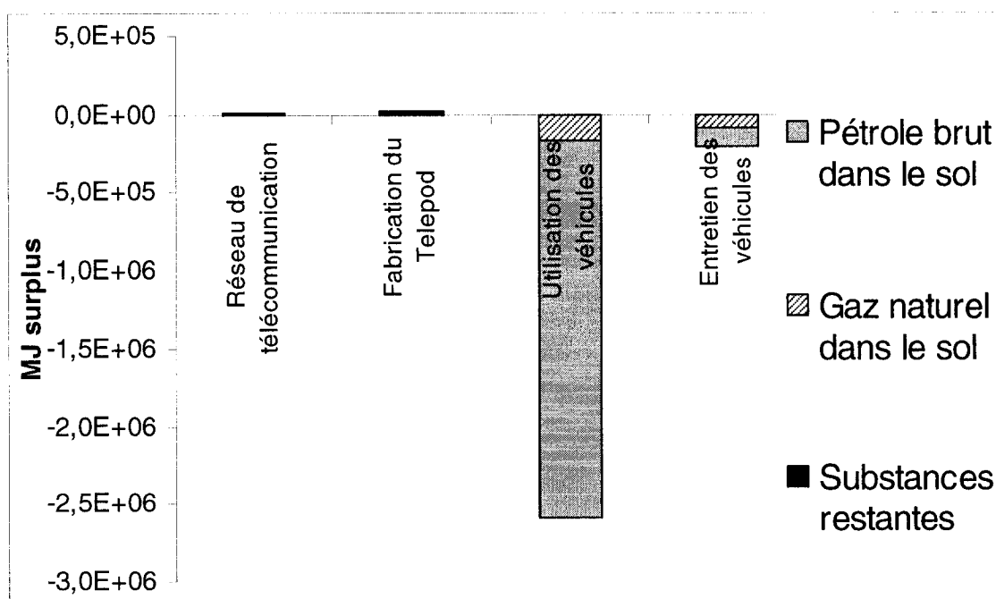
Figure 5.7 : Contribution de l'utilisation des divers combustibles fossiles à l'indicateur de catégorie d'utilisation de combustible fossile pour les différents processus impliqués dans l'ACV du Telepod.
