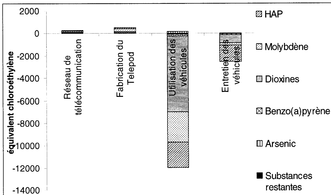
Figure 5.16 : Contribution des divers polluants à l'indicateur de catégorie de la toxicité cancérogène pour les différents processus impliqués dans l'ACV du Telepod.
