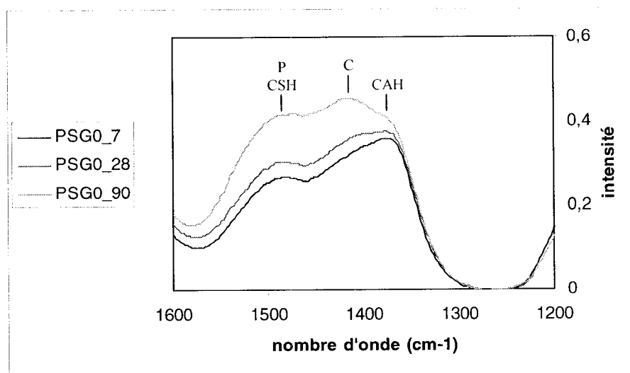
Figure 4.22 : Détails de la zone 1200\text{-}1400\text{ cm}^{-1} des spectres FTIR de l'échantillon PSG0 à différents temps de cure (P : portlandite, C : calcite)
