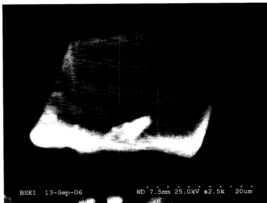
Figure 4.10 : Image MEB en mode électrons rétrodiffusés montrant un grain de portlandite bien cristallisé de l'échantillon QG0_90 (x2500)
