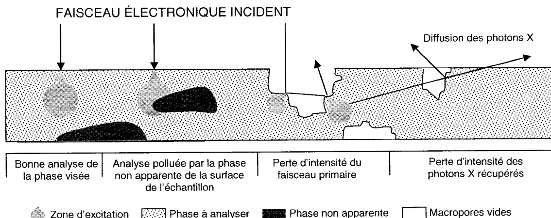
Figure 2.11 : Schéma synthétique des principales causes d'erreur d'analyse élémentaire à l'EDS (d'après Benzaazoua, 1996)
