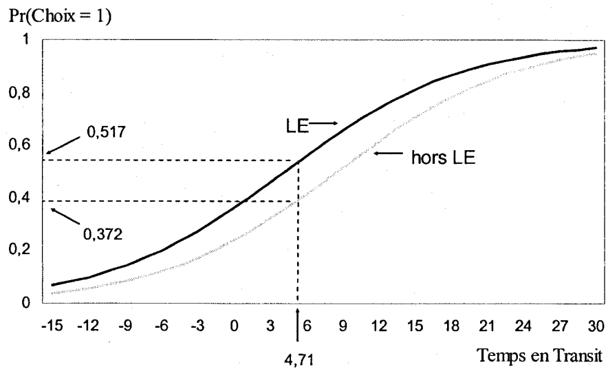
Figure 6.2: Effet de LE sur les probabilités estimées ( TT en abscisses).
