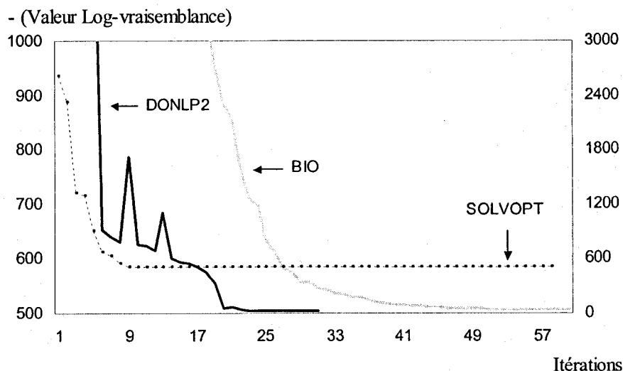
Figure 6.4: Comparaison des méthodes (classes de service régulières).
