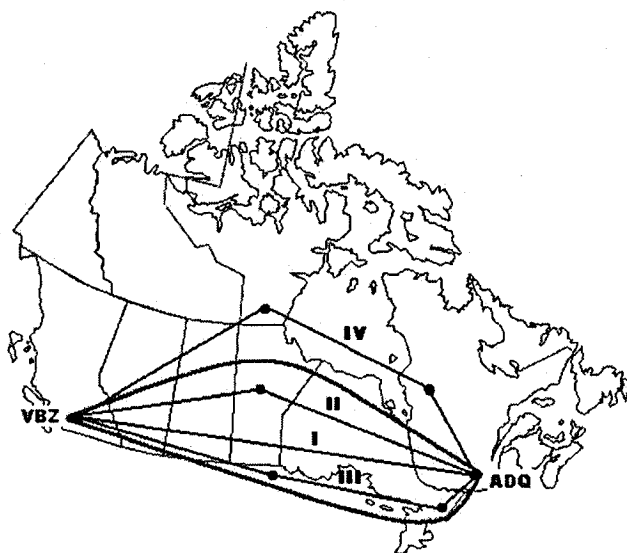
Figure 4.6: Règles de circuité et ensemble d'alternatives 17 .
