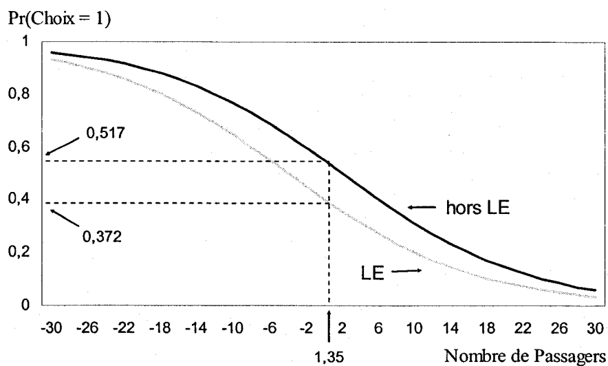
Figure 6.3: Effet de LE sur les probabilités estimées ( NP en abscisses).
