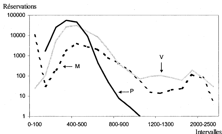
Figure 4.5: Étalement des tarifs (échelle logarithmique).
