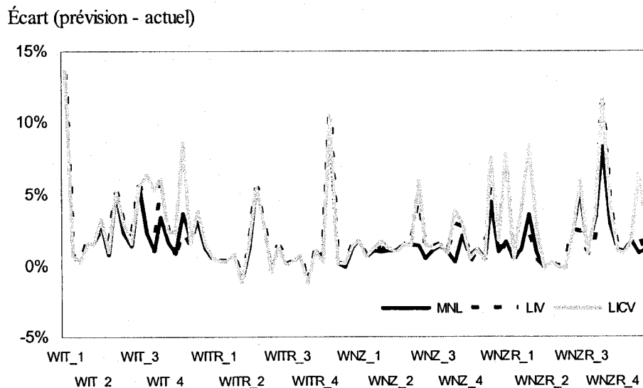
Figure 6.1: Écarts entre les prévisions et données observées.
