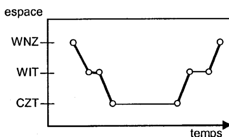
Figure 4.3: Voyage de l'exemple 4.1.
