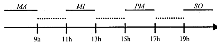
Figure 4.8: Intervalles d'heures de départ.
