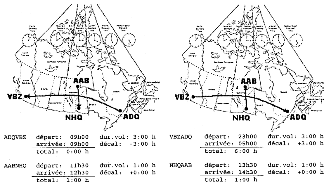
Figure 4.7: Durée de vol et décalage-horaire 19 .
