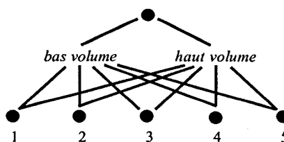
Figure 5.2: Structure imbriquée croisée de nids.
