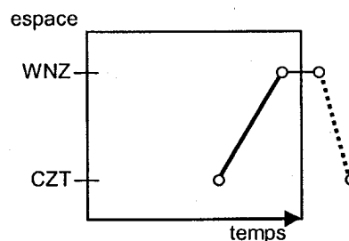
Figure 4.4: Voyage coupé par l'échantillon.
