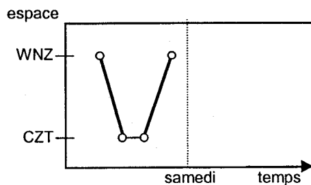
Figure 4.1: Voyage d'affaires type.
