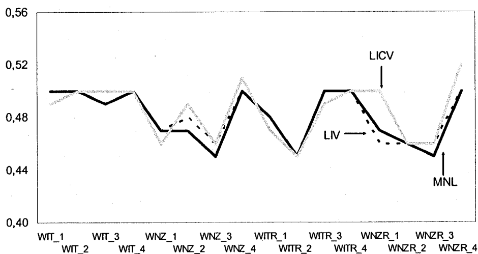
Figure 5.3: Comparaison des rho-carrés ajustés.
