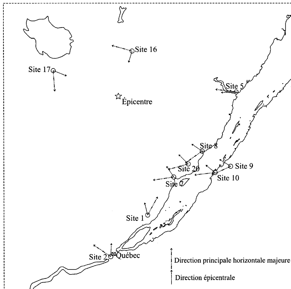
FIG. 3.3 Axes horizontaux principaux majeurs et axes épacentraux des enregistrements du séisme du Saguenay.
