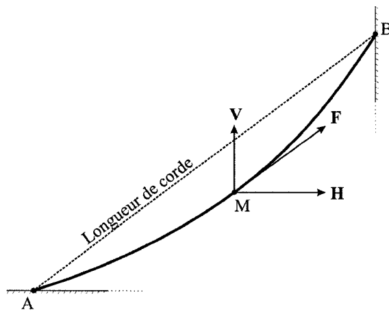
FIG. 4.6 Vue en profil de la déformée d'une chaînette.
