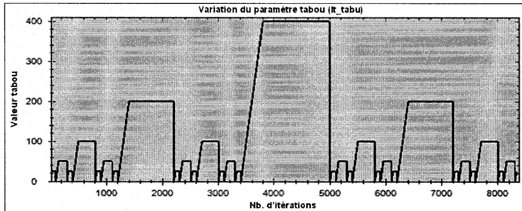
Figure 6 : Variation du paramètre Tabou ( It_{\text{tabu}} )
