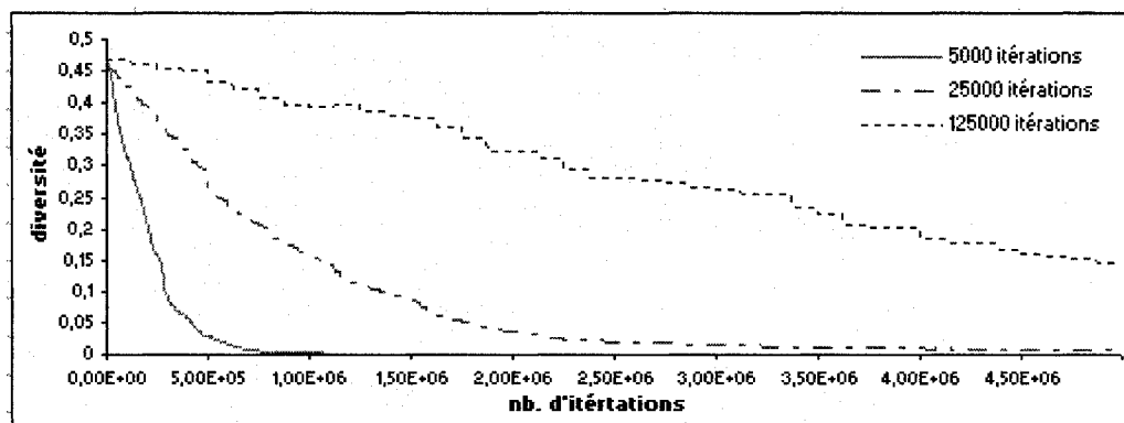
Figure 12 : Courbes d'évolution de la diversité (bcsstk32, k=16 , Imb=5\% ).
