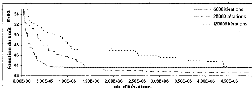
Figure 13 : Courbes d'évolution de la fonction de coût (bcsstk32, k=16 , Imb=5\% ).
