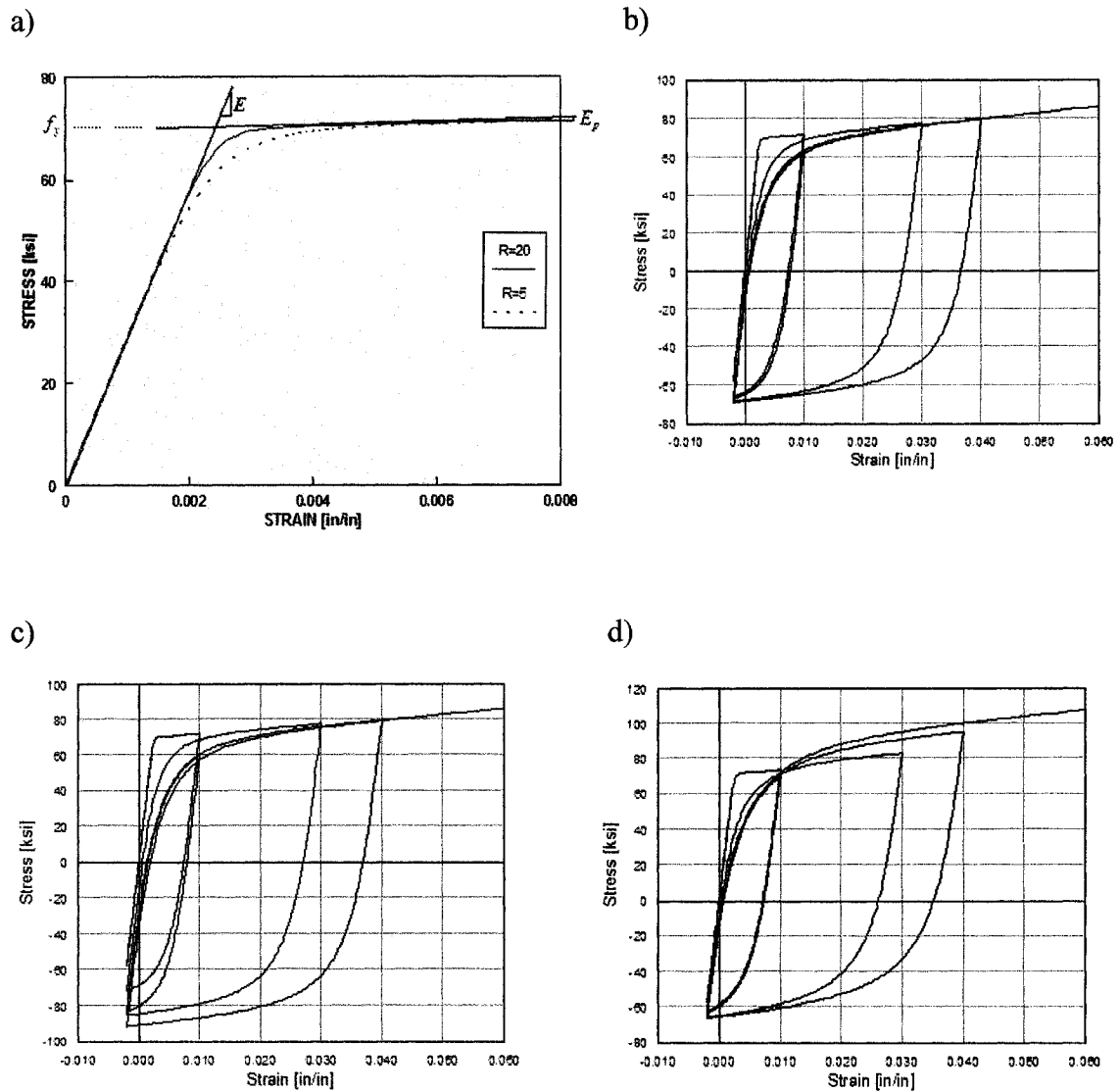
Fig. 3.3.1.1 Steel02 Material
