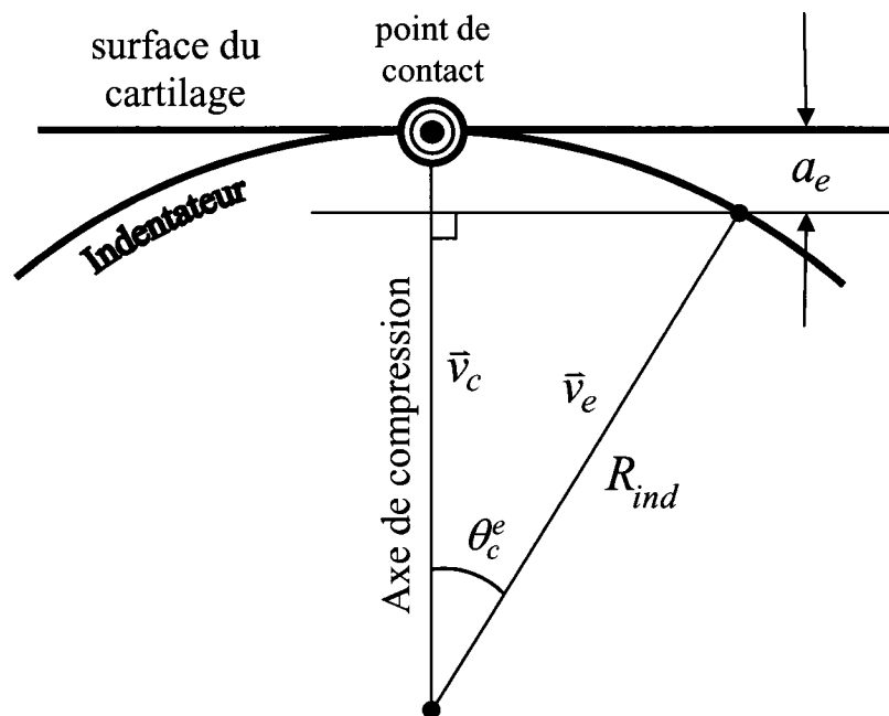
Figure 2-9: Schéma du contact entre l'indentateur sphérique et la surface du cartilage. Les vecteurs \vec{v}_c et \vec{v}_e , de longueurs R_{ind} , joignent respectivement le centre de l'indentateur sphérique au point de contact et à une microélectrode. La microélectrode est située à une distance a_e du point de contact parallèlement à l'axe de compression \vec{v}_c . L'angle entre les deux vecteurs \vec{v}_c et \vec{v}_e est \theta_c^e .
