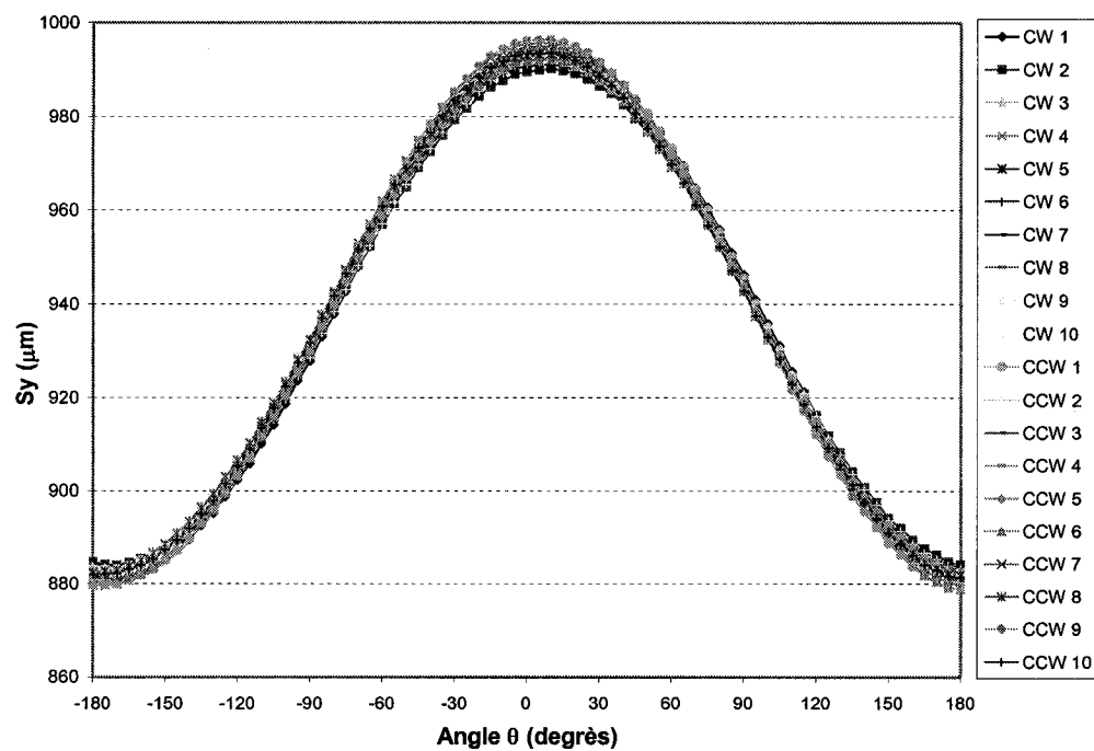
Figure G.8- Valeurs mesurées S_y sur la Mitsui Seiki HU-40
