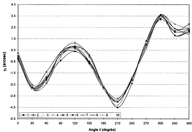
Figure F.5- Écart de positionnement angulaire \gamma_z pour la direction positive
