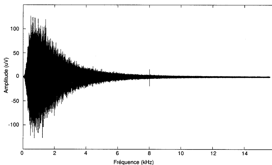
FIG. 2.3 Transformée DCT
