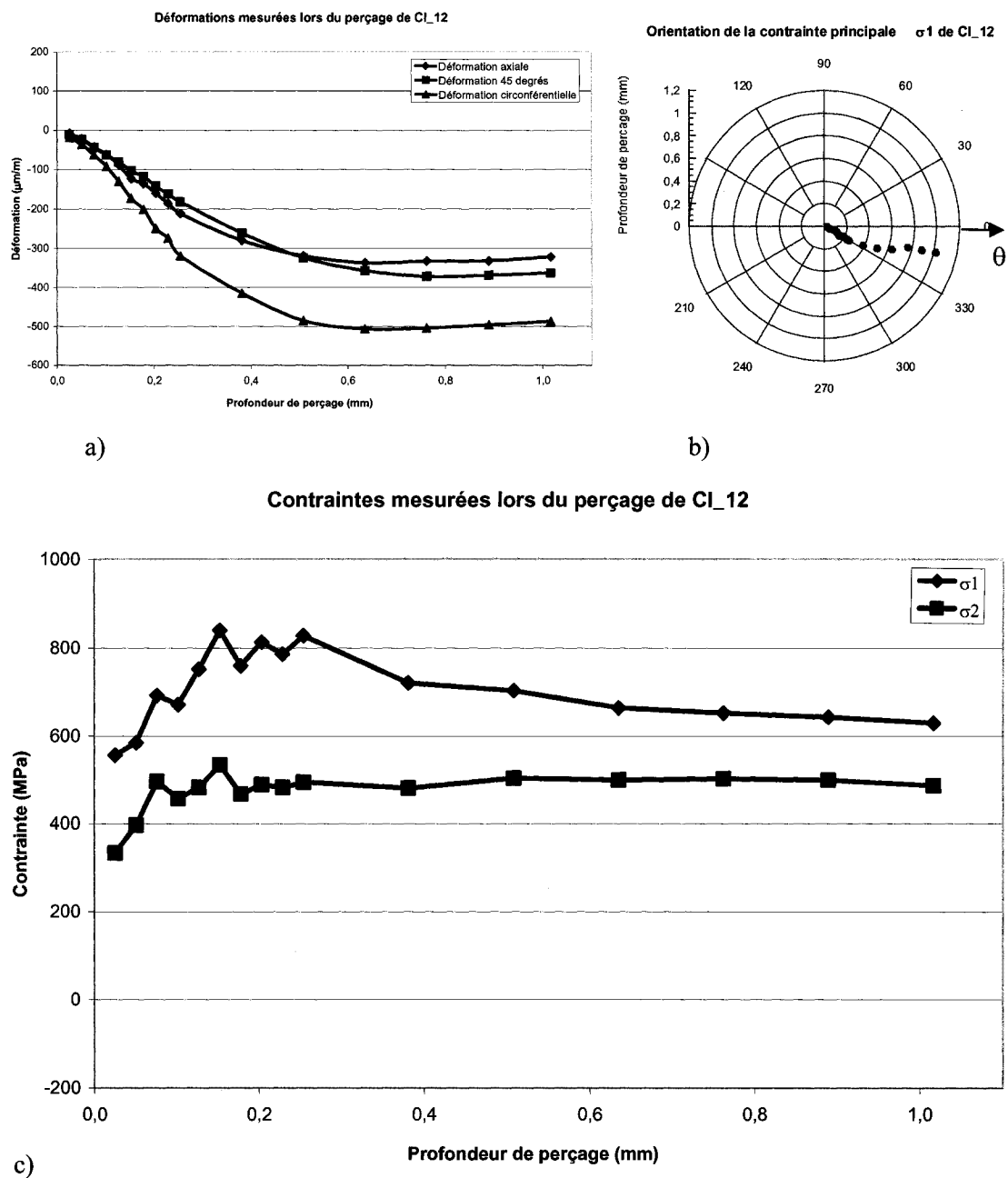
Figure E.5 : Résultats du perçage de CI_12 : a) Variation des déformations mesurées en fonction de la profondeur de perçage b) Variation de l'orientation de la contrainte principale par rapport à la direction circonférentielle c) Variation des contraintes principales calculées à l'aide de la méthode de la contrainte uniforme
