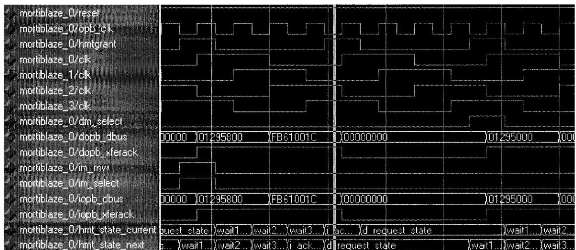
Figure 4.1 : Simulation de la fenêtre d'opération du Microblaze 0
