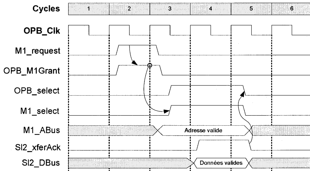
Figure 2.2 : Transaction de bus typique [IBM02]
