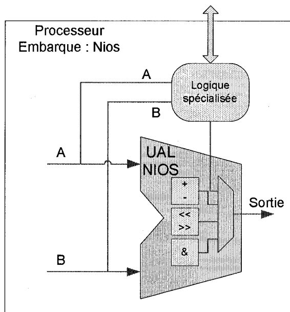
Figure 1.6 : Flot des instructions spécialisées du Nios II [ALTE04]
