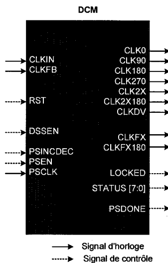
Figure 3.5: Schéma bloc d'un DCM [XILI04]
