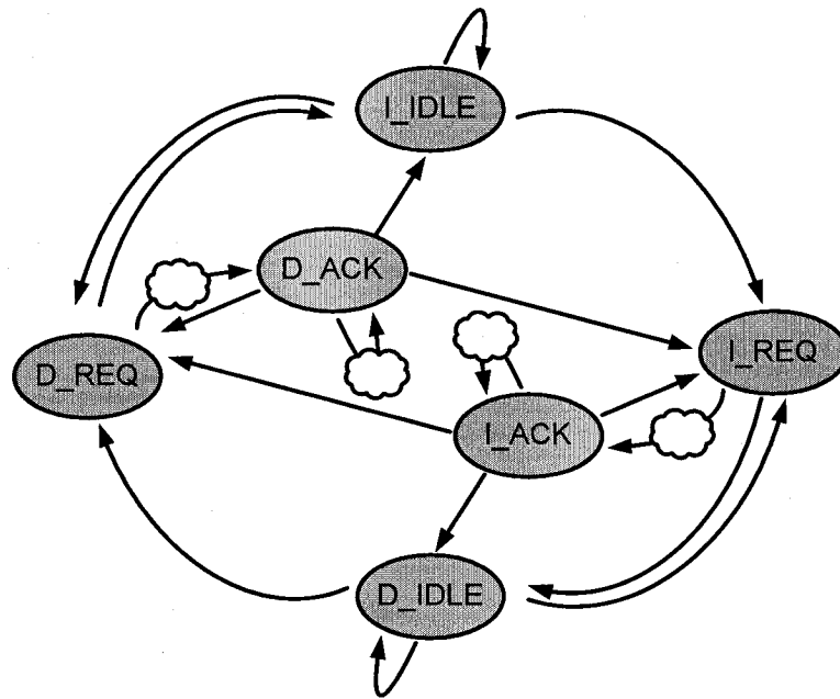
Figure 3.7: Machine à état du « Mortiblaze »
