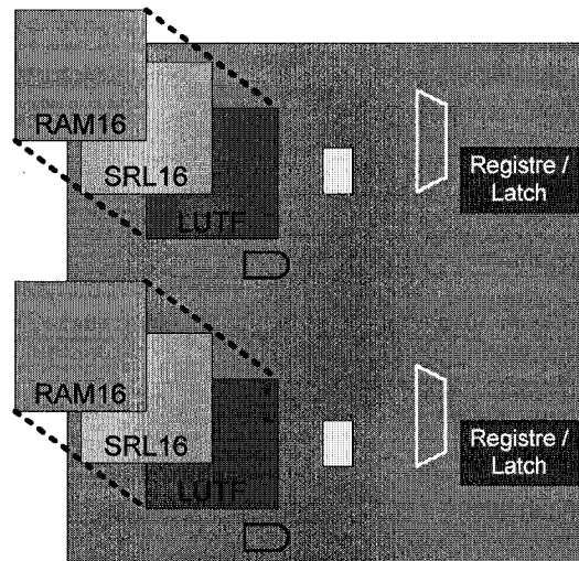
Figure 1.2 : Arrangement d'une tranche d'un Virtex 2 et Virtex 2 Pro [XILI04]
