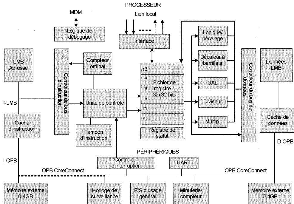
Figure 1.7 : Schéma bloc du Microblaze et de certains périphériques [XILI04c]
