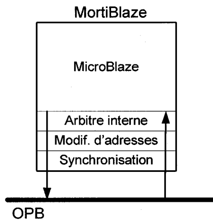
Figure 3.6: Shema bloc d'un « Mortiblaze »
