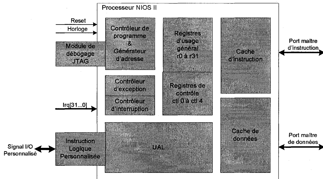
Figure 1.5 : Schéma bloc du Nios II [ALTE04a]
