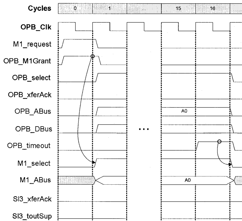
Figure 2.3 : Transaction trop longue : génération d'un timeout [IBM02]
