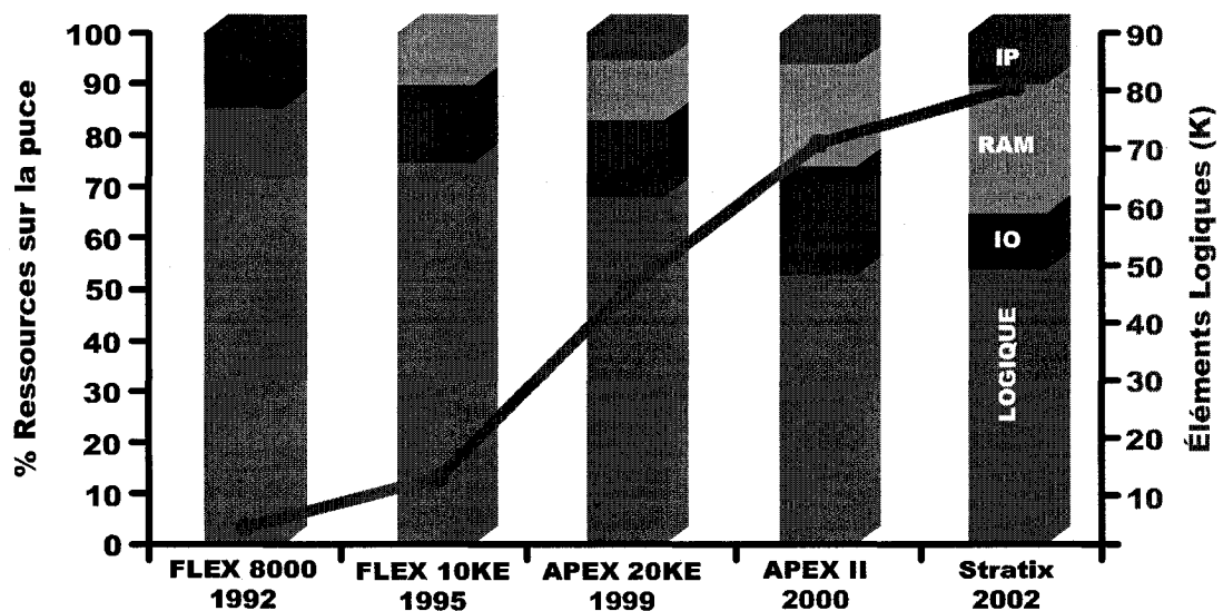
Figure 1.1 : Évolution du contenu des FPGA de Altera [ALTE04]
