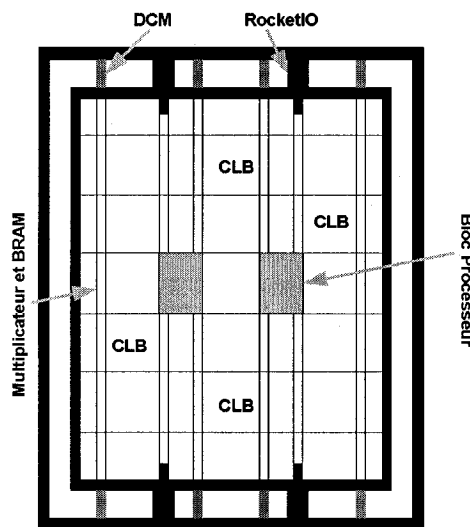
Figure 1.3 : Vue d'ensemble de l'architecture d'un Virtex 2 Pro [XILI04]
