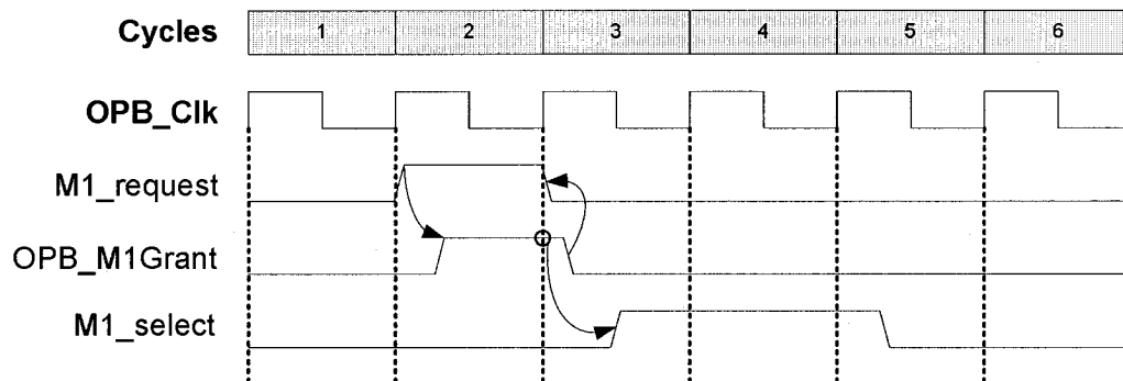
Figure 2.1 : Protocole d'arbitration typique de l'OPB [IBM02]
