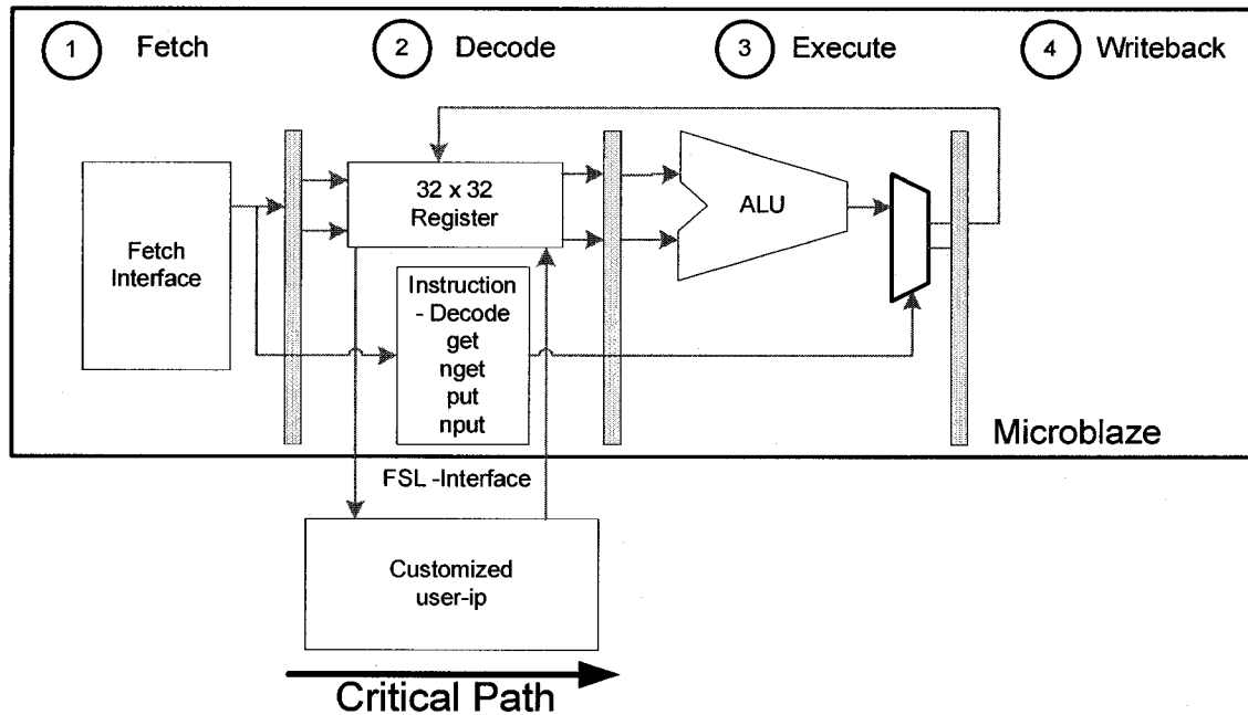
Figure 1.8 : Interface FSL dans le pipeline du Microblaze [XILI04c]
