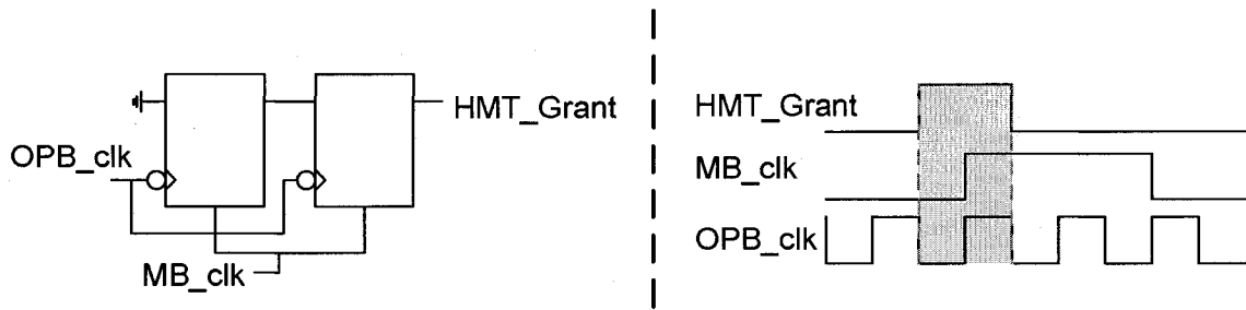
Figure 3.8 : Génération du signal de synchronisation.
