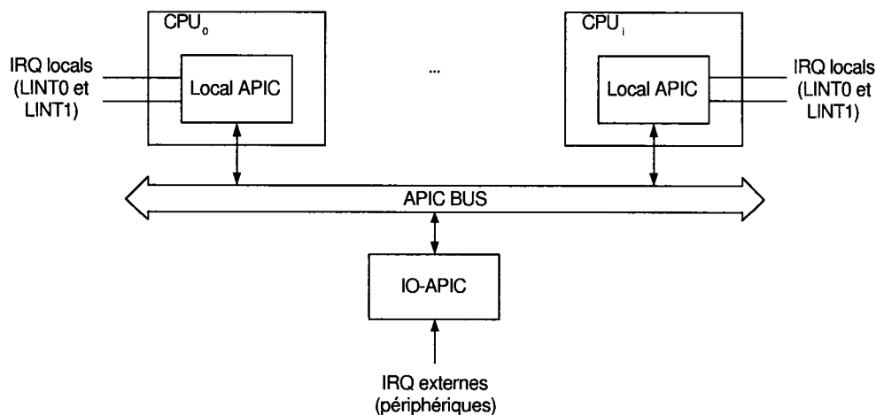
Figure 2.2 Schéma du APIC
