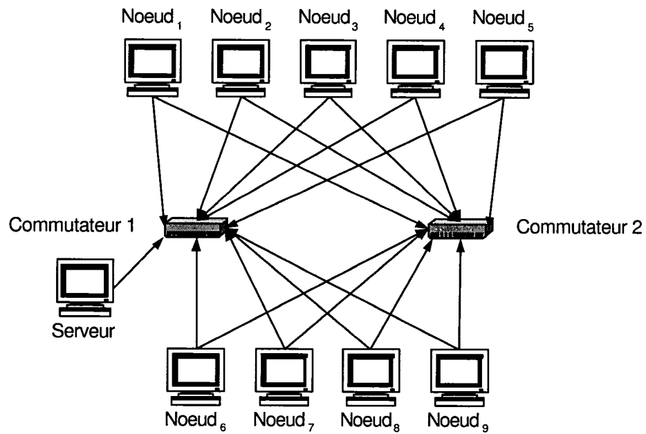
Figure 4.9 Architecture réseau de la grappe de calcul
