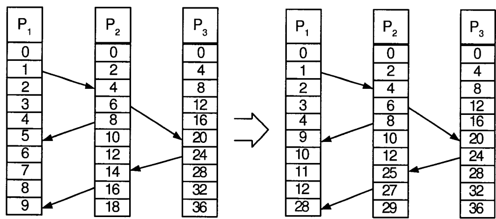
Figure 1.4 Horloge logique de Lamport
