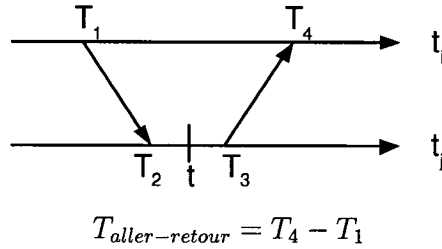
Figure 1.9 Temps d'aller-retour entre deux machines i et j
