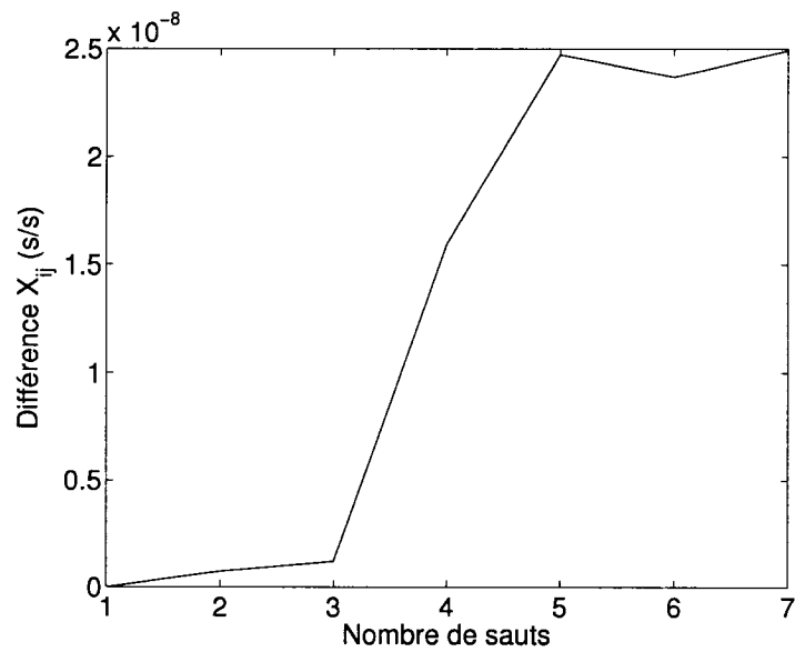
(a) Progression de la différence de X_{ij} en fonction du nombre de sauts (intervalle de confiance de 90%)
