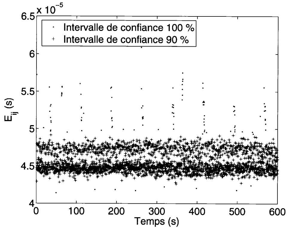
Figure 4.2 Marge d'erreur pour chaque aller-retour selon un intervalle de confiance de 90 et 100 %
