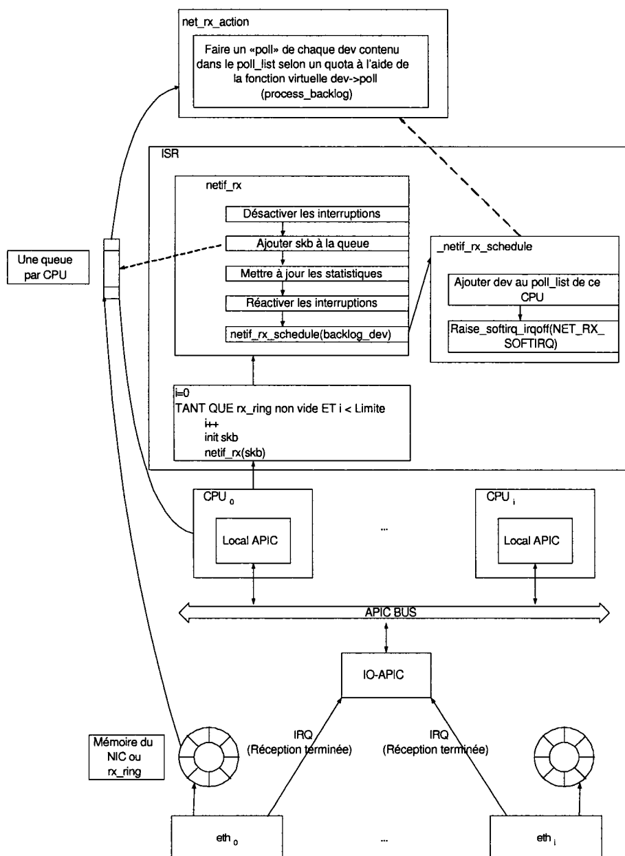
Figure 2.4 Réception de paquets selon l'approche OAPI
