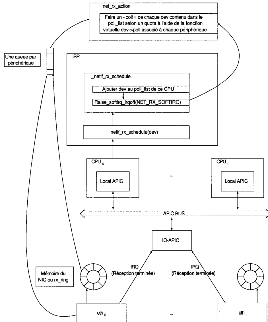
Figure 2.5 Réception de paquets selon l'approche NAPI
