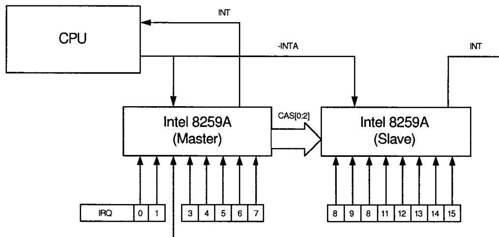
Figure 2.1 Schéma du PIC
