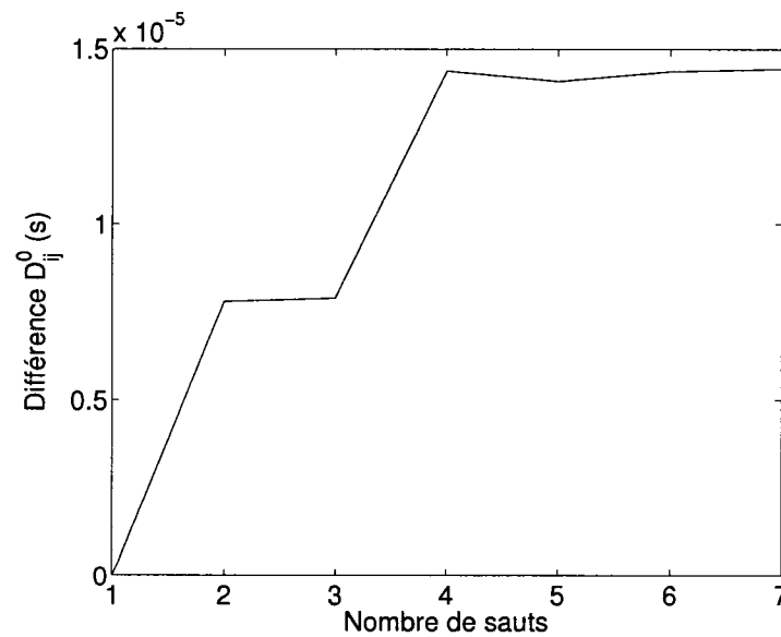
(b) Progression de la différence de D_{ij}^0 en fonction du nombre de sauts (intervalle de confiance de 90%)
