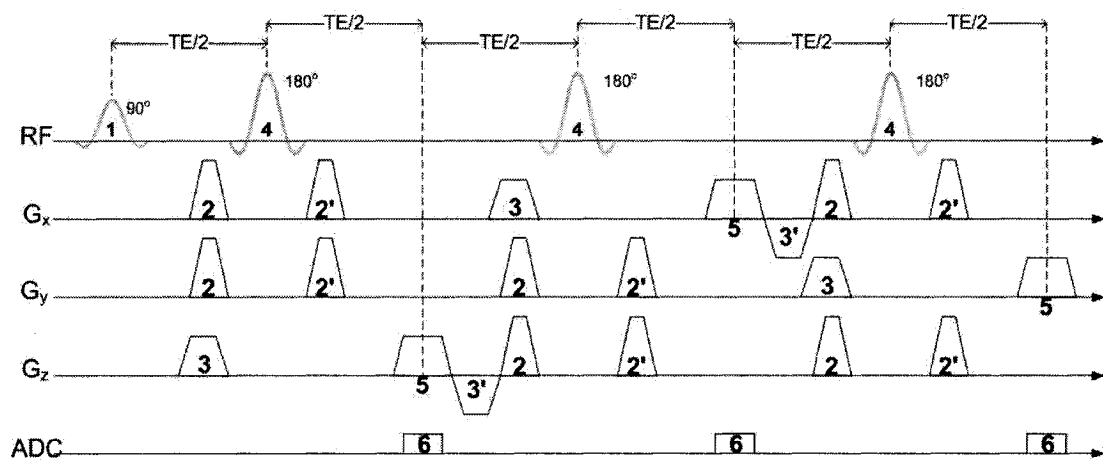
Figure 4.2: Séquence de tracking à écho de spin avec 'crushers'
