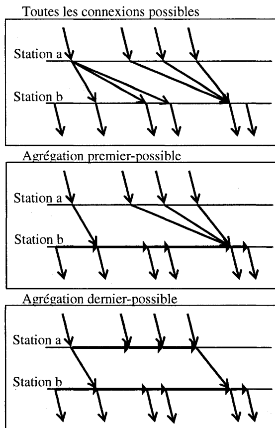
Figure 1.3 – Agrégation des connexions inter-tâches pour le réseau espace-temps
