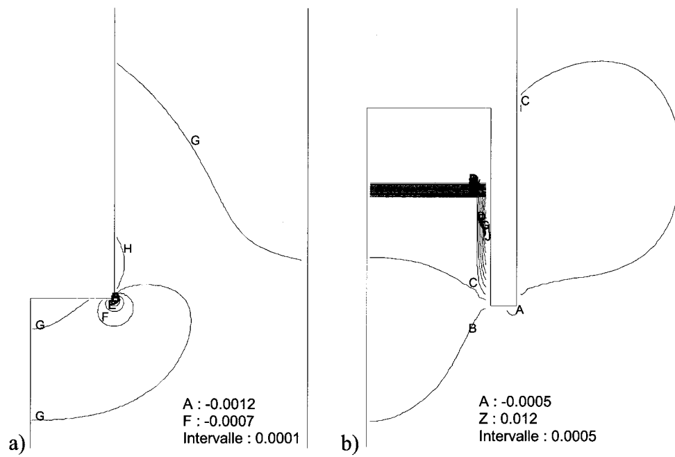
Figure 4.22 – Déformations moyennes.
