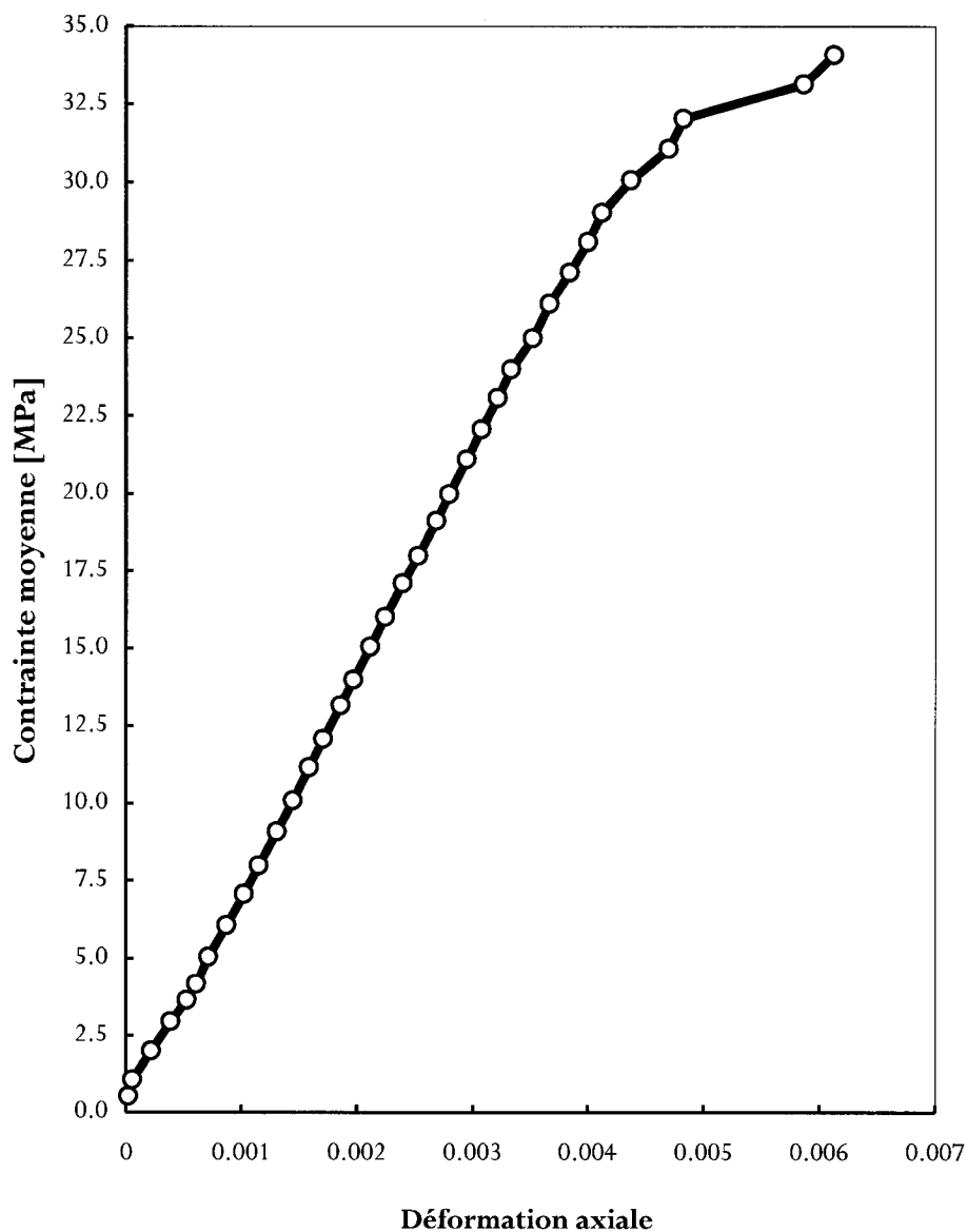
Figure 3.9 – Essai hydrostatique.
