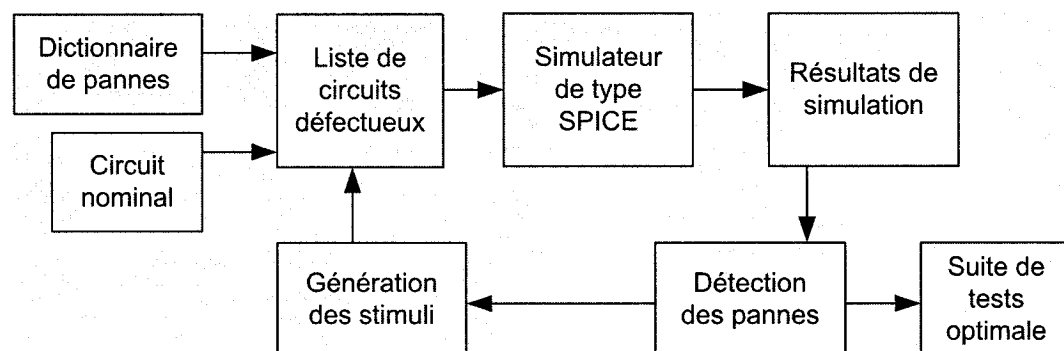
Figure 1.1 : Schéma-bloc de la simulation de pannes analogiques
