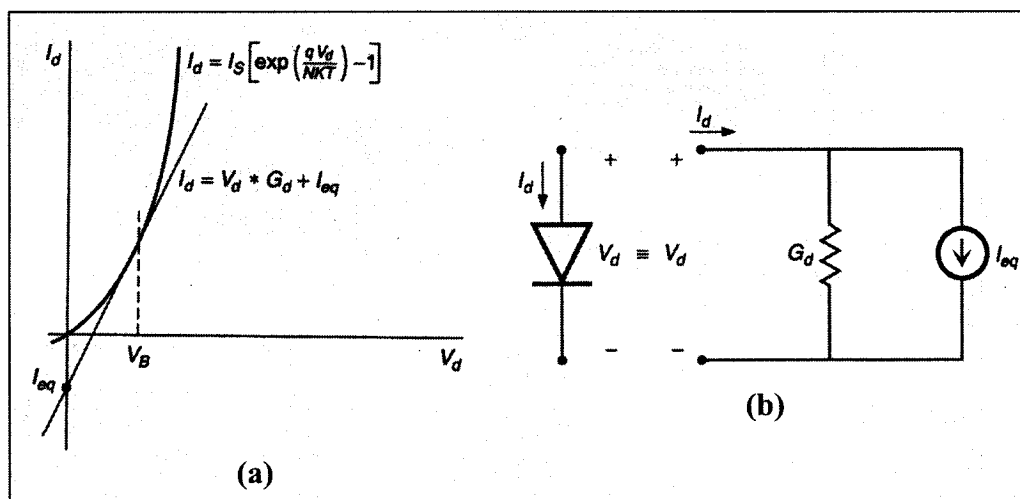
Figure A.3 : Exemple de linéarisation d'une diode (tirée de : [29])
