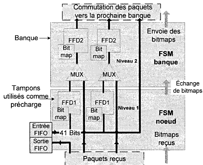
Figure 3-3. Modules du RoC avec ses chemins de données
