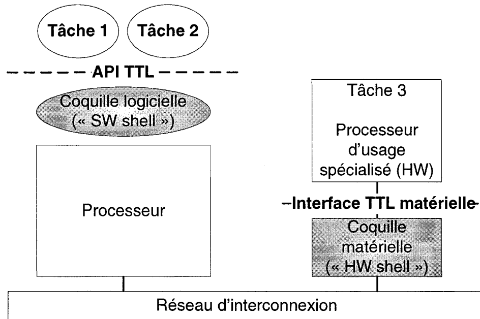
Figure III.1 L'interface TTL et ses coquilles logicielles et matérielles [3]
