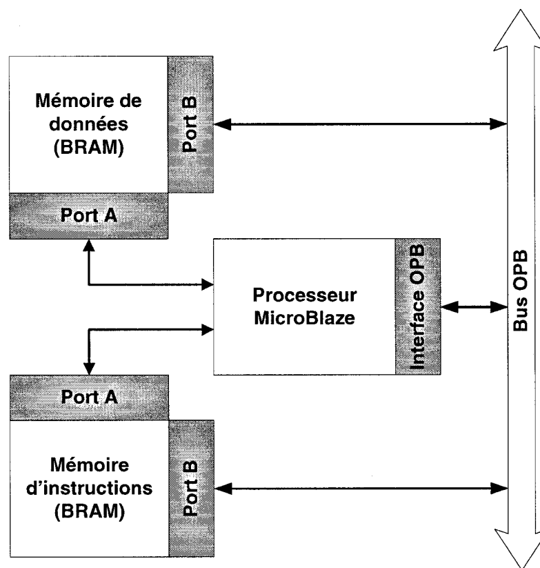
Figure 5.4 Organisation architecturale simplifiée d'un processeur MicroBlaze utilisant des mémoires locales accessibles globalement.
