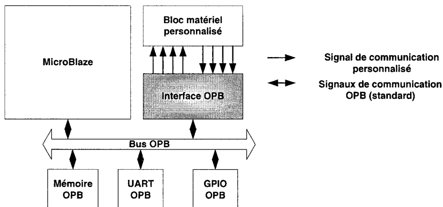
Figure 2.6 Plateforme conçue à partir de la méthodologie de conception basée sur l'assemblage de noyaux IP
