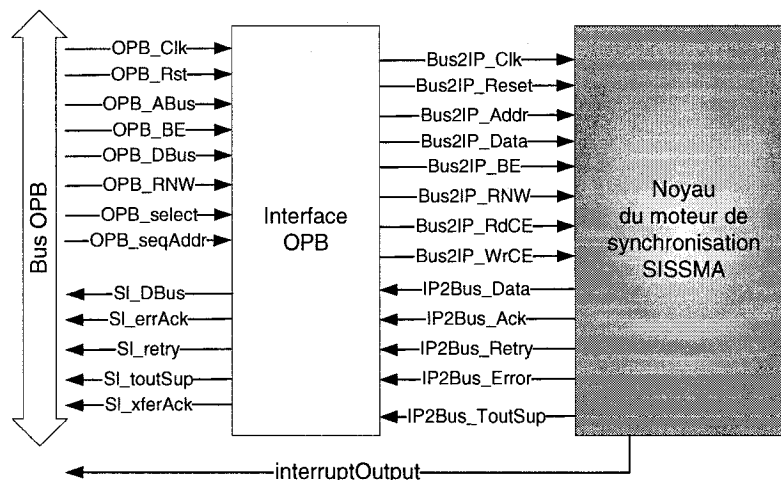
Figure 4.7 Interface de communication et noyau logique du moteur de synchronisation SISSMA
