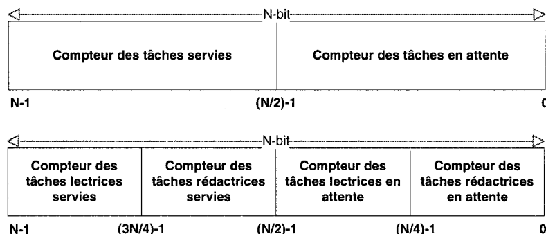
Figure 4.8 Structure du registre d'état d'un sémaphore du moteur de synchronisation SISSMA
