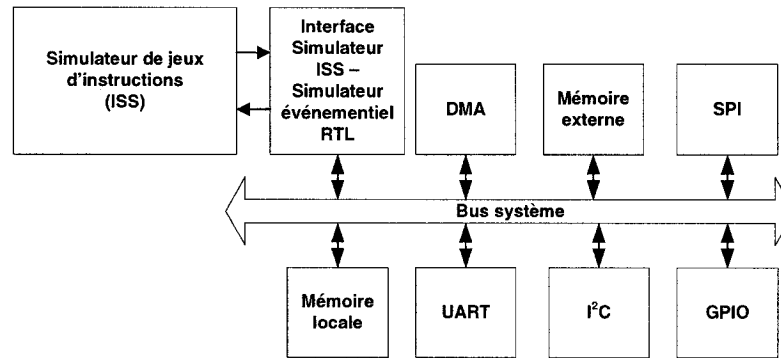
Figure 2.4 Configuration d'une co-simulation logicielle/matérielle entre un simulateur de jeux d'instructions et une partition matérielle
