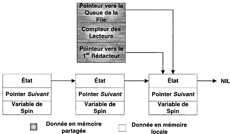
Figure 3.3 Organisation de la mémoire des objets de synchronisation MCS de type rédacteur/lecteur
