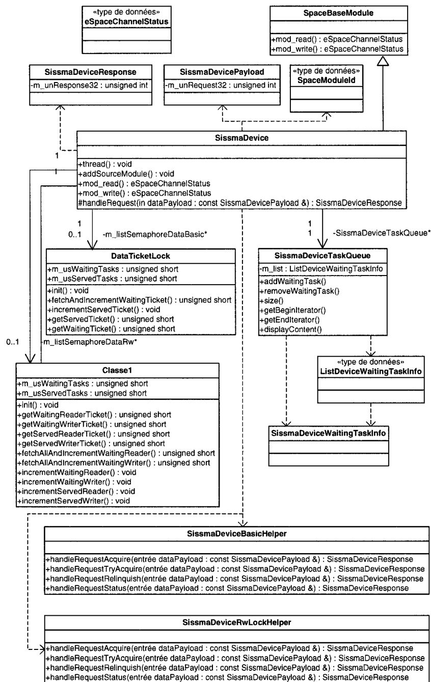
Figure 4.6 Diagramme de classe simplifié du modèle TLM du moteur de synchronisation SISSMA
