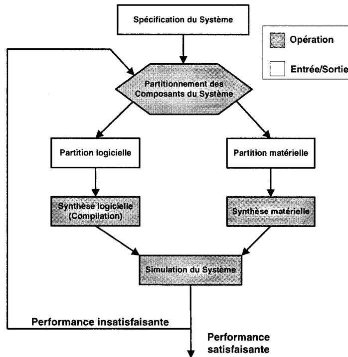
Figure 2.1 Processus de partitionnement logiciel/matériel
