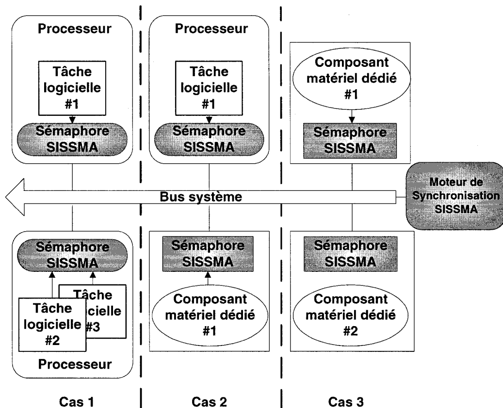
Figure 4.3 Cas d'utilisation de la synchronisation à distance lors de la configuration d'un sémaphore SISSMA
