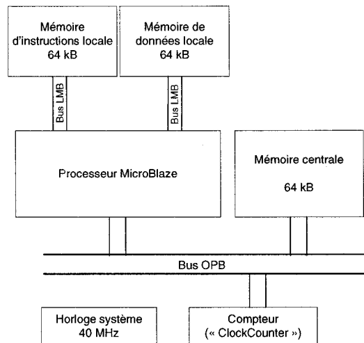
Figure 5.1 Architecture de la plateforme d'analyse monoprocesseur utilisée
