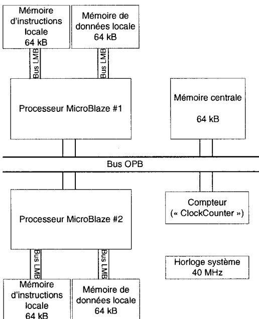
Figure 5.2 Architecture de la plateforme d'analyse multiprocesseur utilisée
