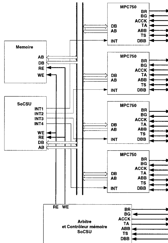
Figure 3.2 Architecture matérielle d'un système à 4 processeurs utilisant le composant SoCSU/SoCLC
