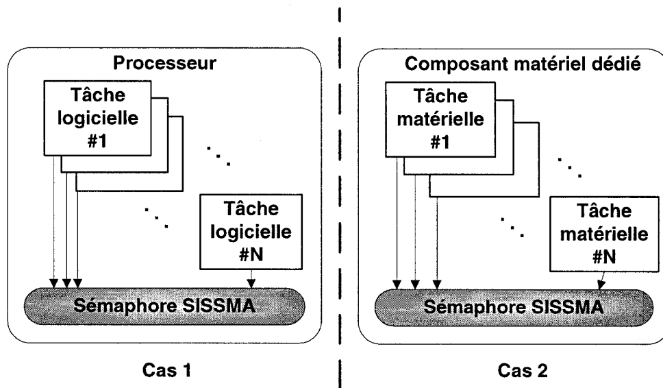
Figure 4.2 Cas d'utilisation de la synchronisation locale lors de la configuration d'un sémaphore SISSMA
