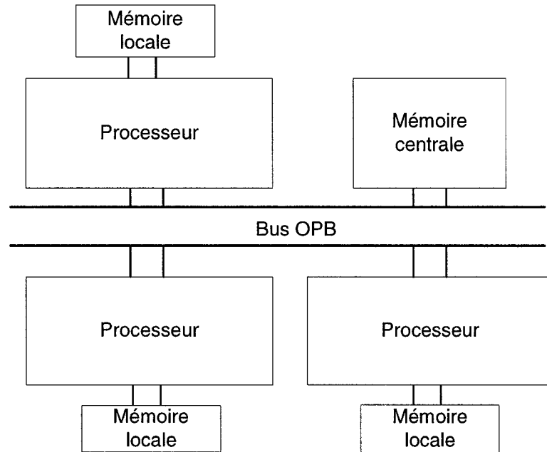
Figure 4.1 MPSoC typique ciblé par les présents travaux
