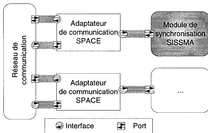
Figure 4.5 Organisation architecture du module SISSMA dans la plateforme SPACE simulation. Ce modèle a ensuite servi de guide lors de l'implantation de son équivalent VHDL.
