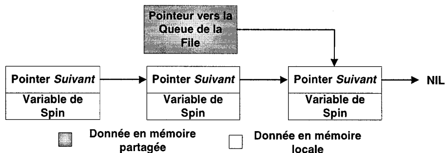
Figure 3.1 Organisation de la mémoire des objets de synchronisation MCS à exclusion mutuelle
