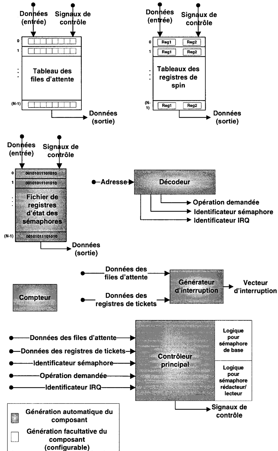
Figure 4.9 Composition matérielle du moteur de synchronisation SISSMA
