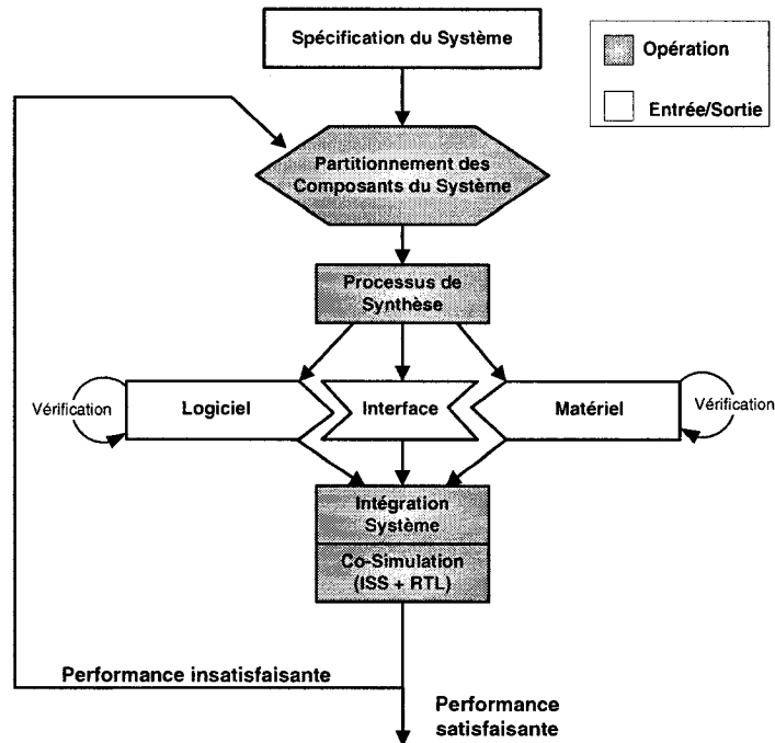
Figure 2.3 Flot de conception du codesign logiciel/matériel
