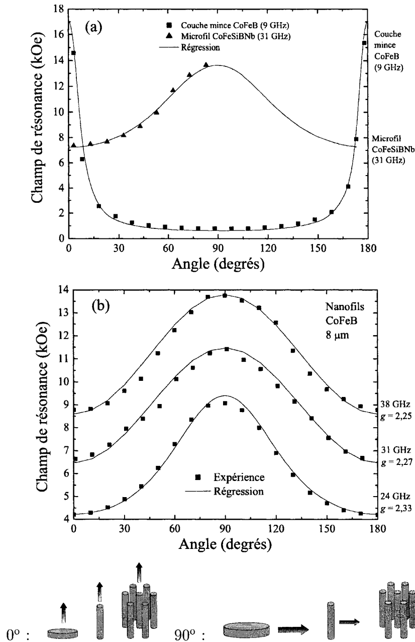
FIGURE 5.6 Champs de résonance en fonction de l'angle pour une couche mince de CoFeB à 9 GHz et un microfil de CoFeSiBNb à 31 GHz (a), un réseau de nanofils de CoFeB à plusieurs fréquences (b) ( 1 \text{ Oe} = 4\pi 10^{-3} \text{ A/m} ).
