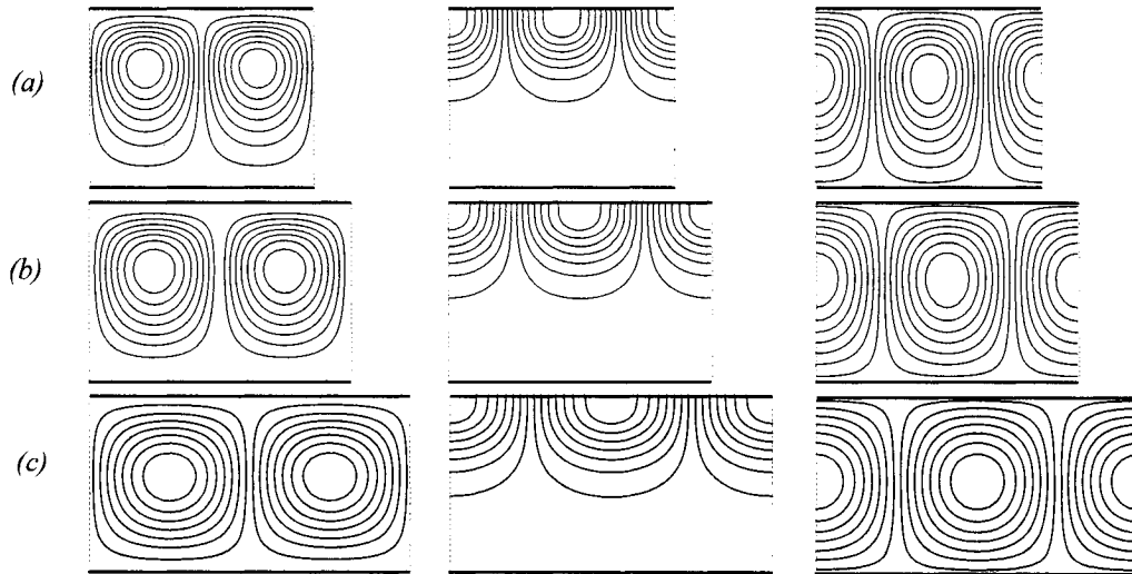
Figure 5.8 : Lignes de courant (à gauche), isoconcentration (au centre) et isothermes (à droite) pour Pe = 1 ; (a) Ra_T = -1000 , (b) Ra_T = 0 , (c) Ra_T = 1000
