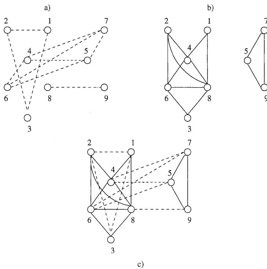
Figure 2.5 – a) Graphe d'incompatibilité de pièces b) Graphe d'incompatibilité temporelle c) Graphe d'intervalles de tâches
