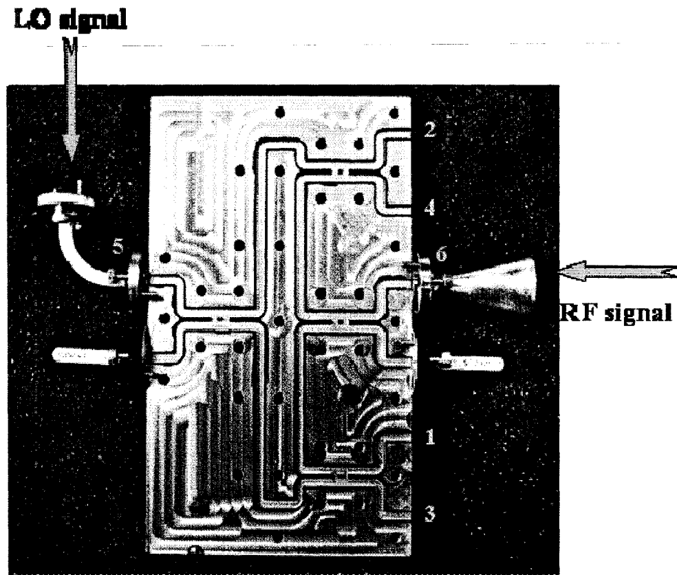
Figure 3.22. Photographie de la section longitudinale du circuit six-port fabriqué dans un bloc de laiton
