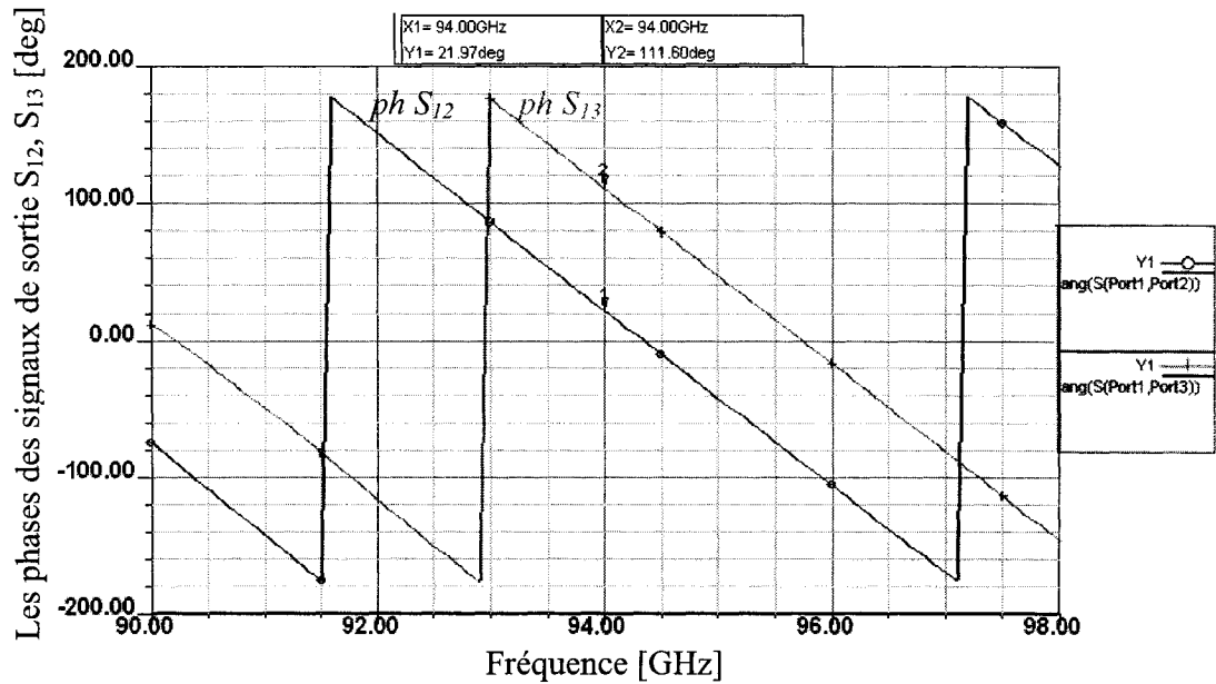
Figure 4.29. Les variations des phases des signaux de sortie S_{12} et S_{13} du coupleur hybride en guide d'onde, intégré au substrat, par rapport à la fréquence
