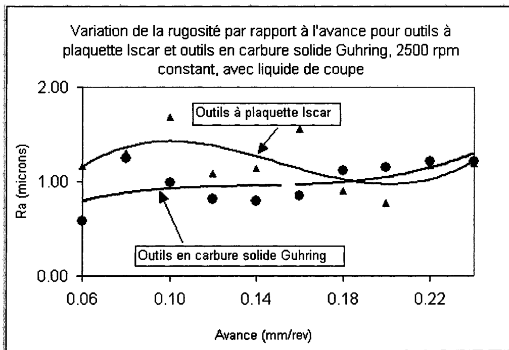
Figure 3.50: Variation de la rugosité Ra par rapport à l'avance pour forets à plaquette et forets en carbure solide, 2500 rpm avec liquide de coupe.
