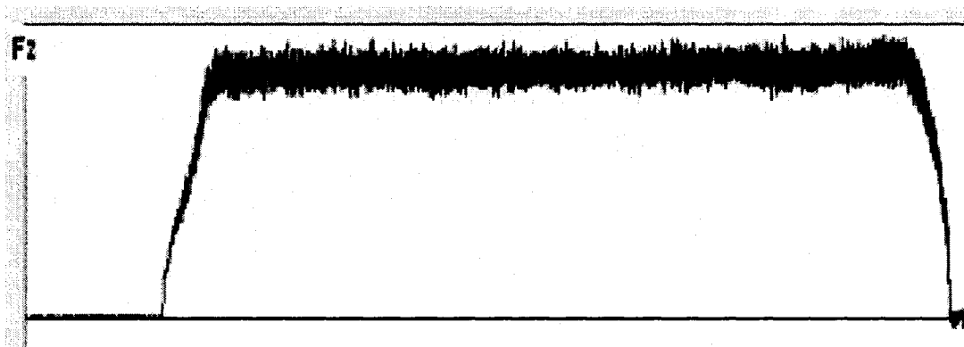
Figure: 3.71. Allure globale de la force F_z pour forets en carbure solide.
