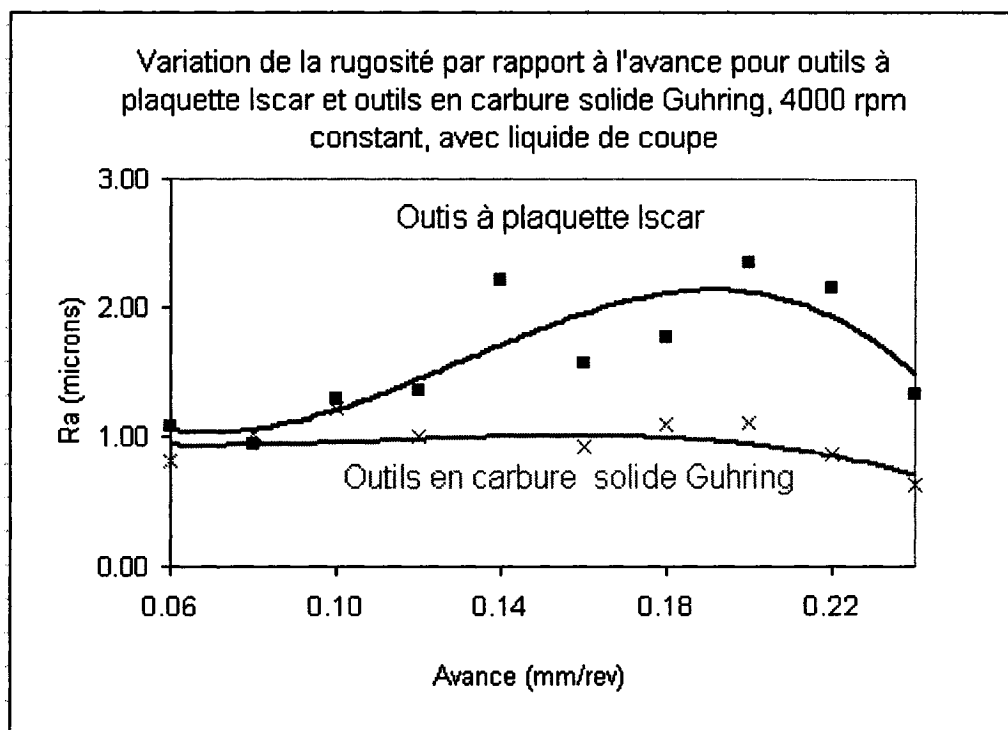
Figure 3.51: Variation de la rugosité Ra par rapport à l'avance pour forets à plaquette et forets en carbure solide, 4000 rpm avec liquide de coupe.
