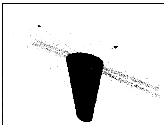
Figure 2.22 : Amélioration des résultats de la méthode MHM obtenus sur les anomalies magnétiques de la figure 2.13 en utilisant le critère de symétrie. Données du tableau de l'annexe C.4 - n° 10, 11 et 12 respectivement.
