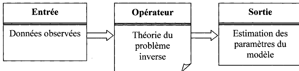
Figure 3.2 : Principe du problème inverse en géophysique
