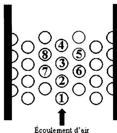
Figure 4.5 Schéma de la section d'essais utilisée par Mureithi et al. (2005)
