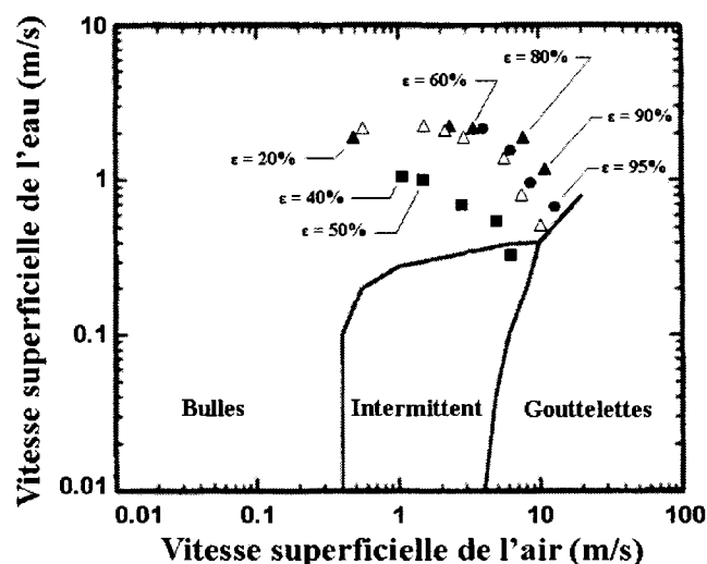
Figure 4.4 Carte de configuration d'écoulement diphasique pour un faisceau de tubes compacts Ulbrich et Mewes (1994) : ■ Vitesses critiques pour un tube flexible dans la direction de la portance, ▲ Vitesses critiques pour un tube flexible dans toutes les directions, Δ Vitesses critiques pour sept tubes flexibles dans toutes les directions disposés sur deux colonnes, ● Vitesses critiques pour sept tubes flexibles seulement dans la direction de l'écoulement situés au centre de la section d'essais.
