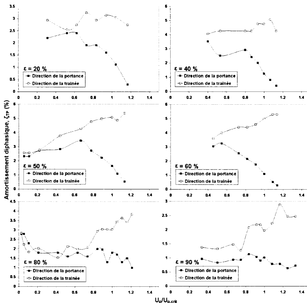
Figure 3.43 Évolution de l'amortissement diphase avec la vitesse de l'écoulement intertubes pour un tube flexible dans toutes les directions
