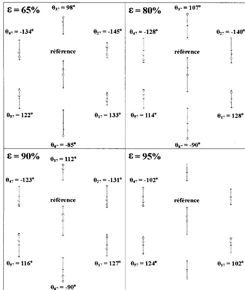
Figure 3.34 Modes instables de vibration, sept tubes flexible en grappe, tubes de 14 Hz libres de vibrer seulement dans la direction de l'écoulement : + position d'équilibre et limite du mouvement des tubes, O position des tubes à un temps arbitraire, \vee direction du mouvement des tubes au temps arbitraire.
