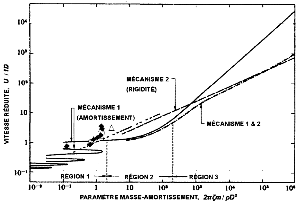
Figure 4.3 Courbe de stabilité théorique obtenue par Paisoussis et Price (1988) pour plusieurs tubes flexibles dans un faisceau rigide triangulaire tourné, P/D = 1,375 :
