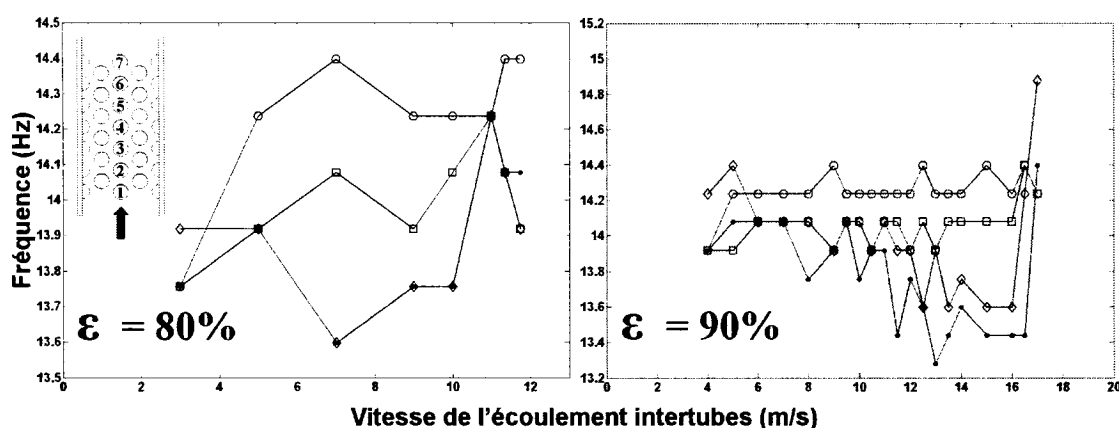
Figure 4.7 Évolution de la fréquence principale d'oscillation des tubes avec la vitesse de l'écoulement intertubes pour une colonne de tubes flexibles dans la direction de l'écoulement : —●— Tube 4, —◇— Tube 5, —□— Tube 6, —○— Tube 7
