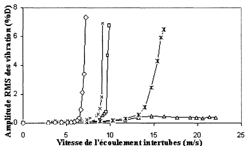
Figure 4.6 Résultats obtenus des tests d'instabilité en soufflerie rapportés par Mureithi et al. (2005) pour toutes les configurations testées (la réponse du tube 2 est montrée) : —△— un tube flexible, —*— deux tubes flexibles (tube 2 et 3), —×— sept tubes flexibles (tubes 2, 3, 4, 5, 6, 7 et 8), —□— une colonne flexible (tubes 1, 2, 3 et 4), —◇— tous les tubes flexibles
