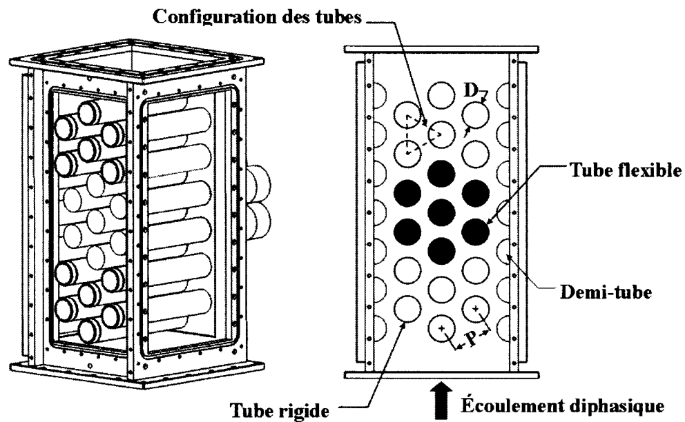
Figure 2.5 Paramètres géométriques et vue isométrique de la section d'essais
