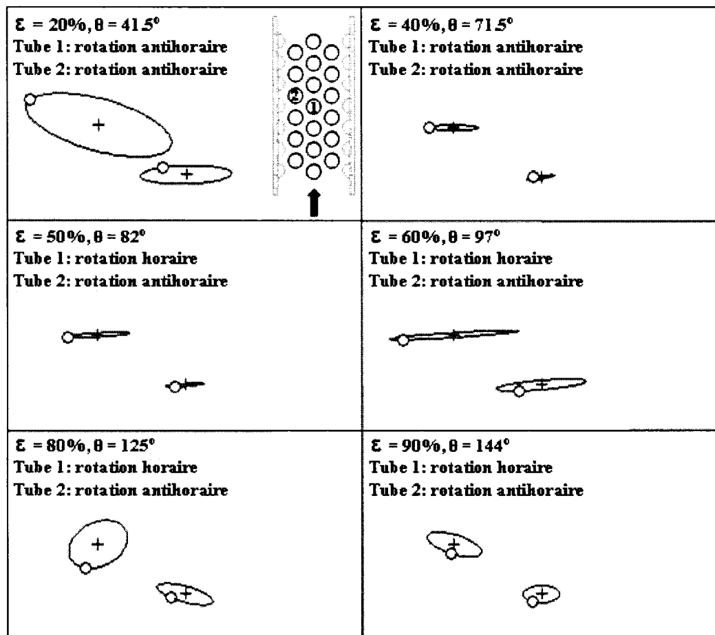
Figure 3.14 Modes instables de vibration à l'instabilité pour deux tubes adjacents libres de vibrer dans toutes les directions : + position d'équilibre des tubes, O position du centre des tubes à un temps arbitraire.
