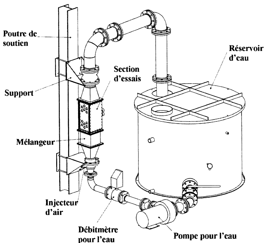
Figure 2.2 Boucle diphasique
