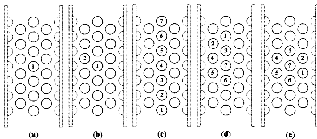
Figure 2.6 Configurations testées : (a) Un tube flexible, (b) Deux tubes adjacents flexibles, (c) Colonne centrale flexible, (d) Deux colonnes partiellement flexibles, (e) Six tubes flexibles regroupés autour du septième
