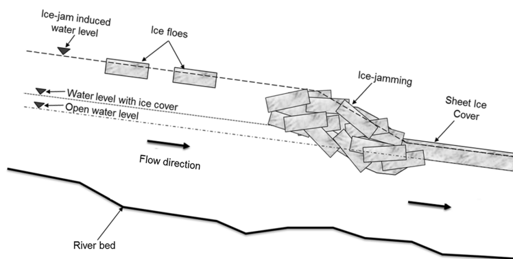
FIGURE 1.3 Vue schématique des embâcles fluviaux et des niveaux d'eau associés [6]
