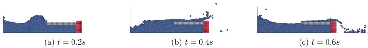
FIGURE 4.22 Ecoulement de l'eau en HPL sur plusieurs pas de temps
