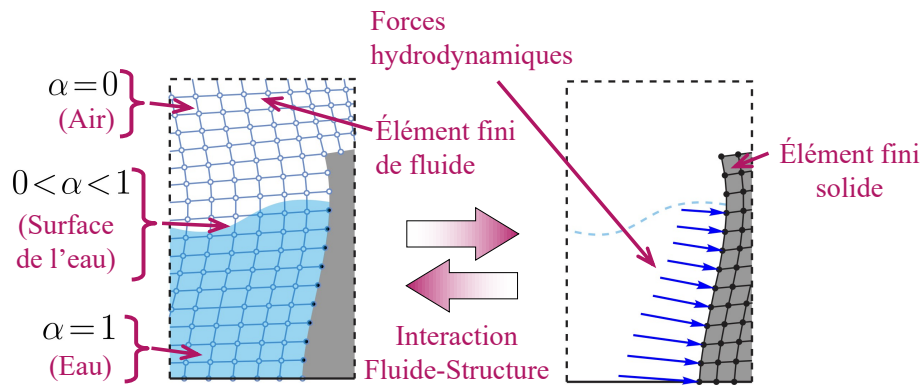
FIGURE 3.2 Schéma explicatif de la méthode de volume de fluide et de l'IFS (Communication personnelle de Bouaanani (2024))
