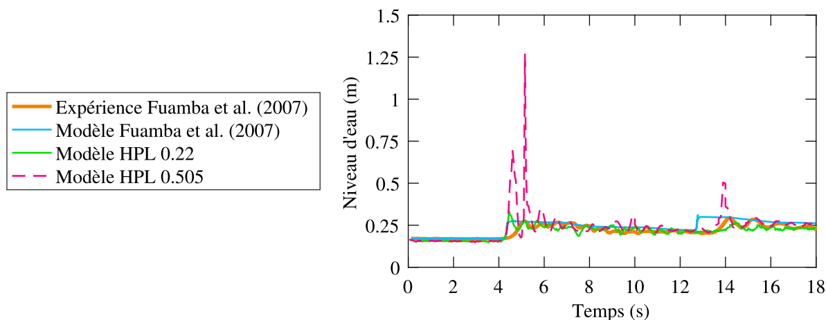
FIGURE 4.31 Hauteur d'eau sans glace au niveau de la structure, avec des structures de 0.22 m et de 0.505 m
