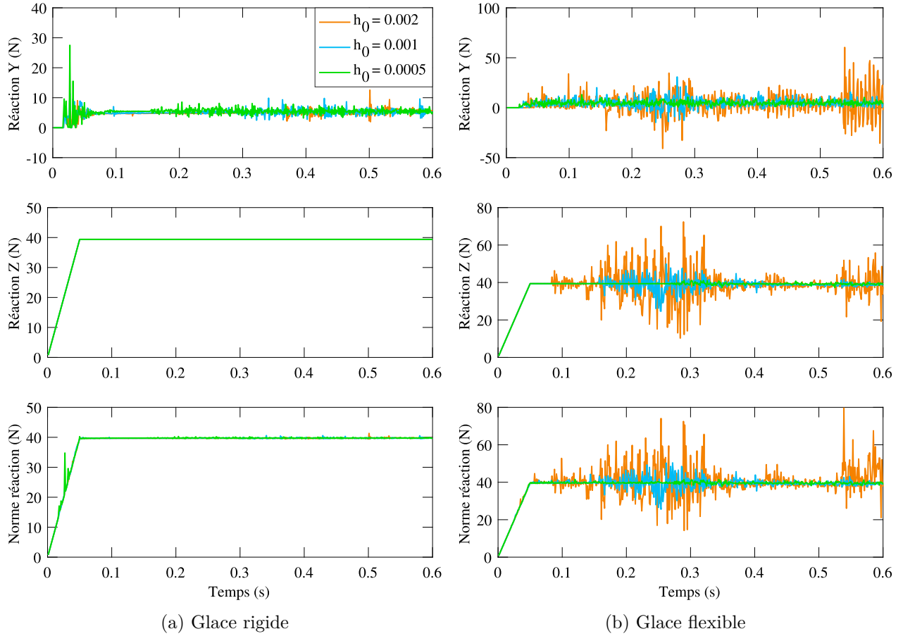
FIGURE 4.14 Comparaison de la réaction à la base de la structure selon plusieurs maillages
