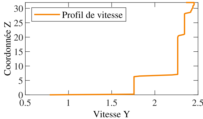
FIGURE 4.37 Profil de vitesse de l'écoulement appliqué à l'entrée du modèle (m/s)
