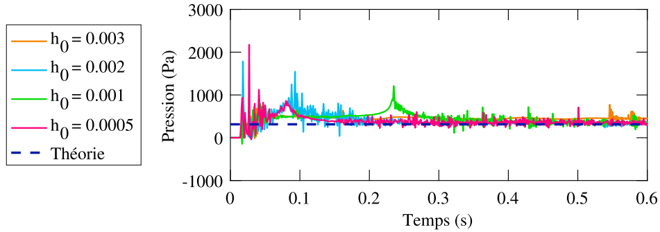
FIGURE 4.4 Pression à la base de la structure pour différents espacements h_0
