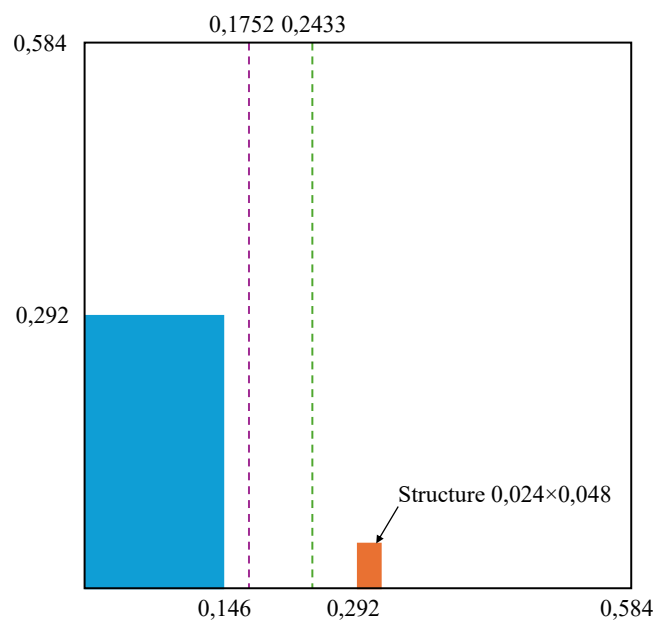
FIGURE 3.45 Emplacement des lignes de troncations (m)
