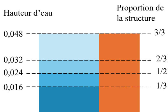
FIGURE 3.29 Niveaux de lits d'eau étudiés. Le niveau d'eau en mètre à gauche, la proportion par rapport à la structure à droite
