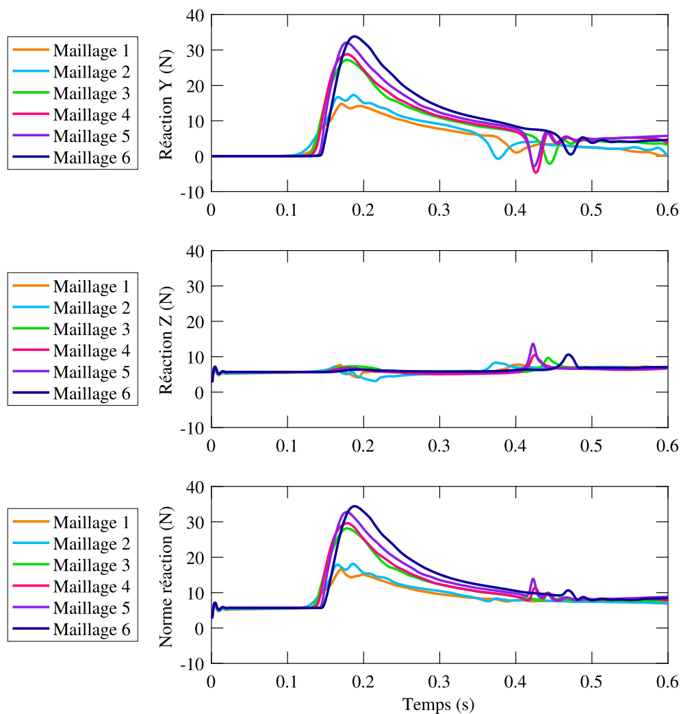
FIGURE 3.8 Réaction à la base de la structure flexible en amont selon les maillages 1 à 6
