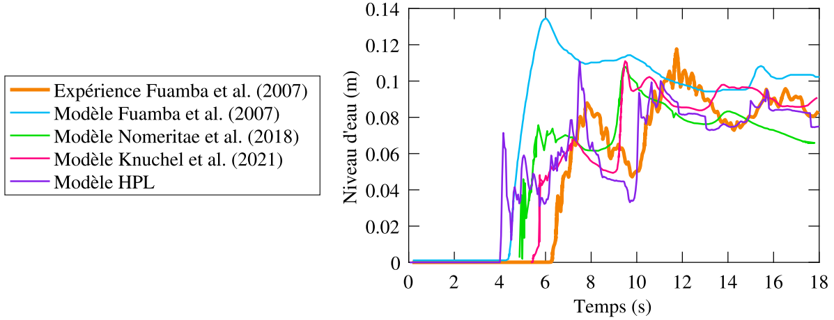
FIGURE 4.35 Hauteur d'eau avec glace au niveau de la structure au dessus du couvert, avec une structure de 0.505 m de haut
