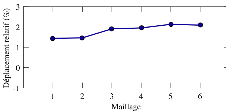
FIGURE 3.7 Déplacement relatif maximal au sommet de la structure flexible en amont selon les maillages 1 à 6
