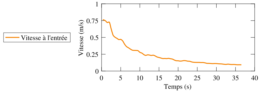
FIGURE 4.29 Profil de vitesse de l'écoulement appliqué au niveau du déversoir
