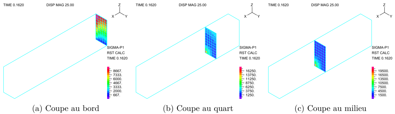
FIGURE 3.21 Coupes de contrainte principale maximale de la structure rigide
