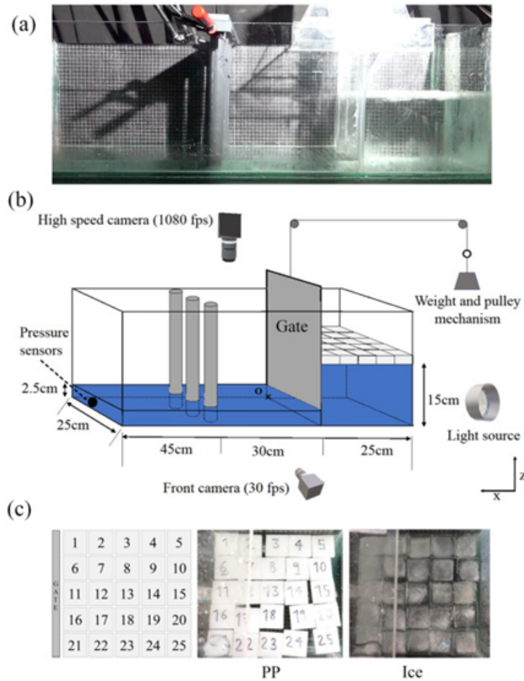
FIGURE 2.20 Configuration expérimentale de rupture de barrage. (a) image de la configuration (b) la configuration schématique et (c) la disposition initiale des blocs. [23]
