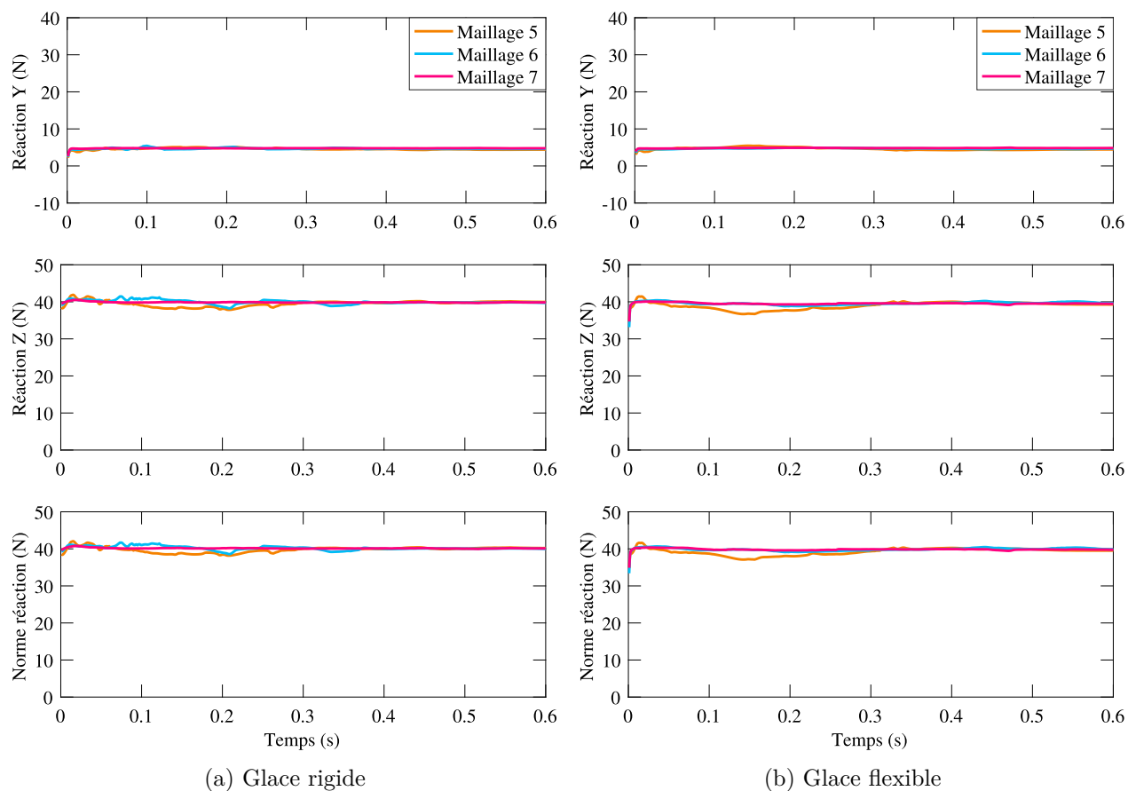
FIGURE 4.9 Comparaison de la réaction à la base de la structure selon plusieurs maillages
