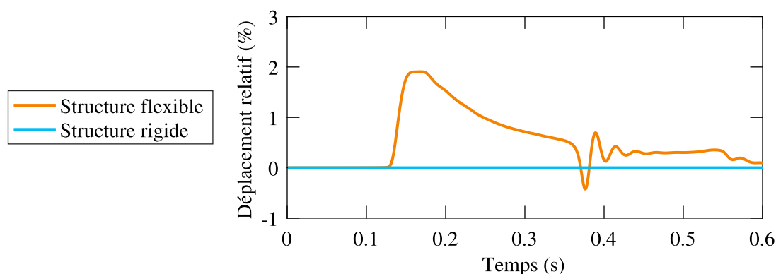
FIGURE 3.18 Déplacement au milieu de la structure en amont de l'écoulement
