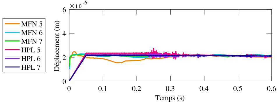
FIGURE 4.19 Comparaison du déplacement à l'extrémité inférieure du couvert de glace flexible pour plusieurs maillages
