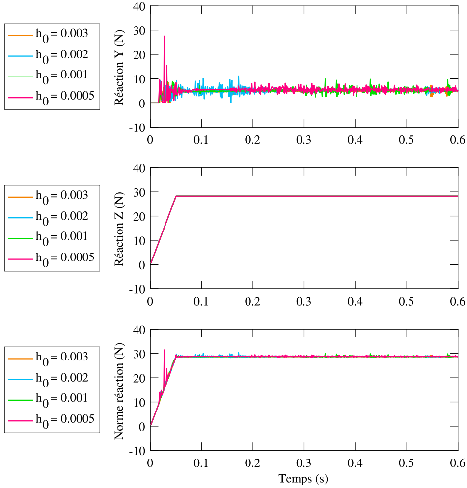
FIGURE 4.5 Réaction à la base de la structure pour différents espacements h_0
