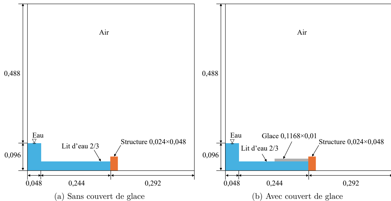
FIGURE 4.20 Dimensions de rupture de barrage modifiées (m)
