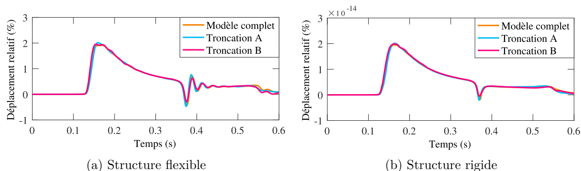
FIGURE 3.47 Comparaison du déplacement relatif au milieu du sommet des modèles complet, troncation A et troncation B
