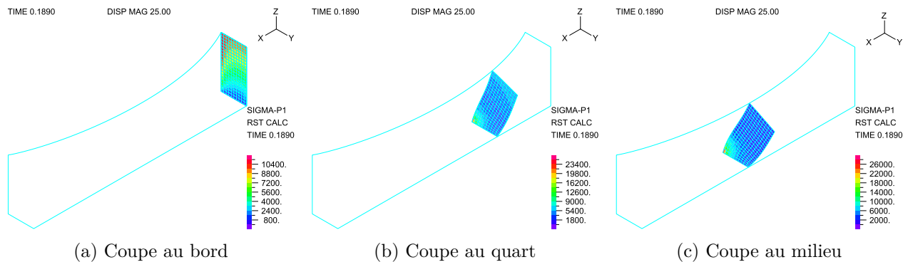
FIGURE 3.16 Coupes de contrainte principale maximale pour le maillage 6
