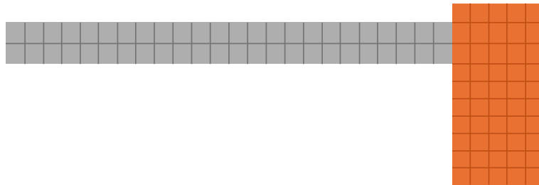
FIGURE 4.7 Maillage de la structure avec couvert de glace pour un maillage 5
