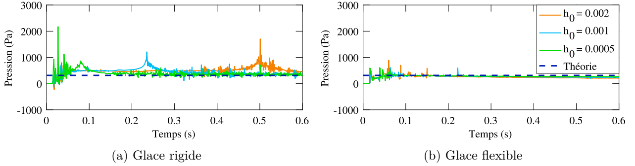
FIGURE 4.13 Comparaison de la pression à la base de la structure selon plusieurs maillages
