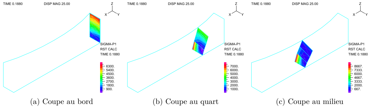
FIGURE 3.12 Coupes de contrainte principale maximale pour le maillage 2
