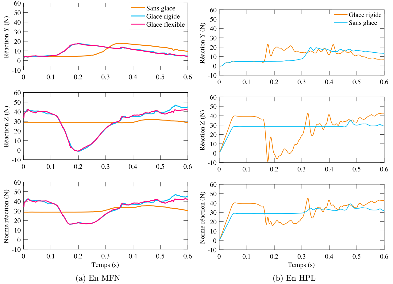
FIGURE 4.23 Réaction à la base de la structure selon différents couverts de glace
