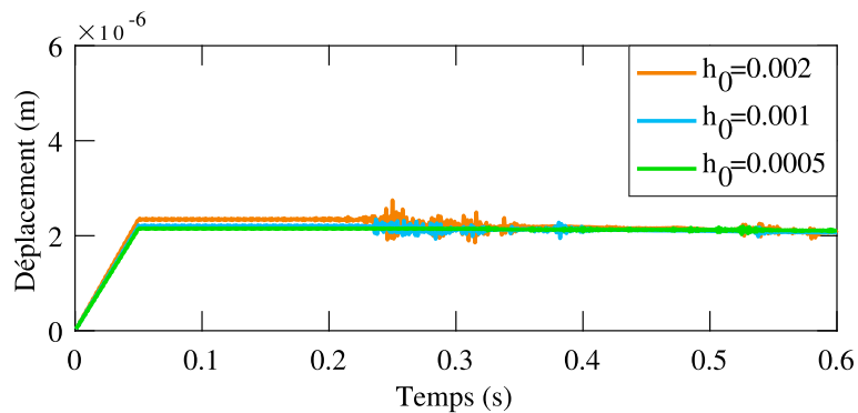
FIGURE 4.16 Déplacement à l'extrémité de la glace flexible selon plusieurs maillages
