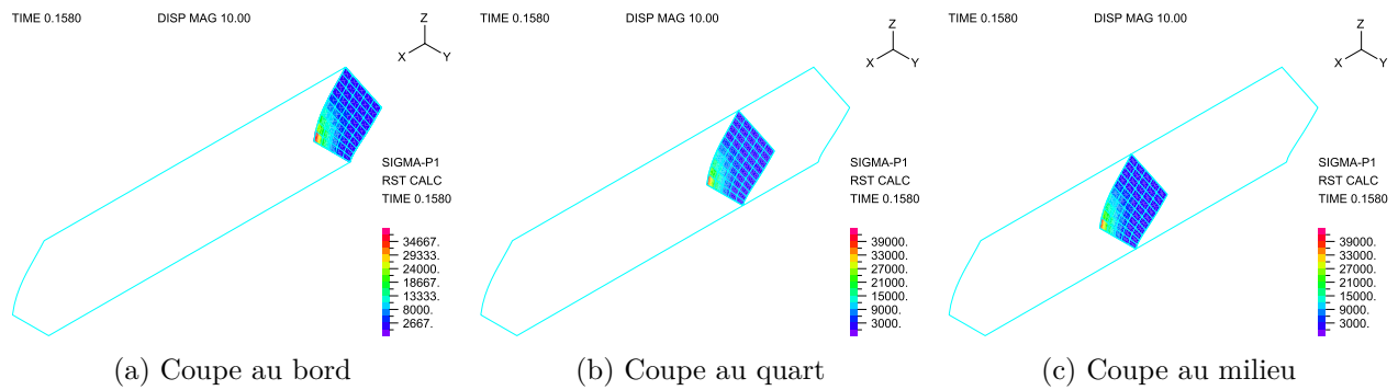
FIGURE 3.27 Coupes de contrainte principale maximale de la structure flexible avec bords libres pour le maillage 5
