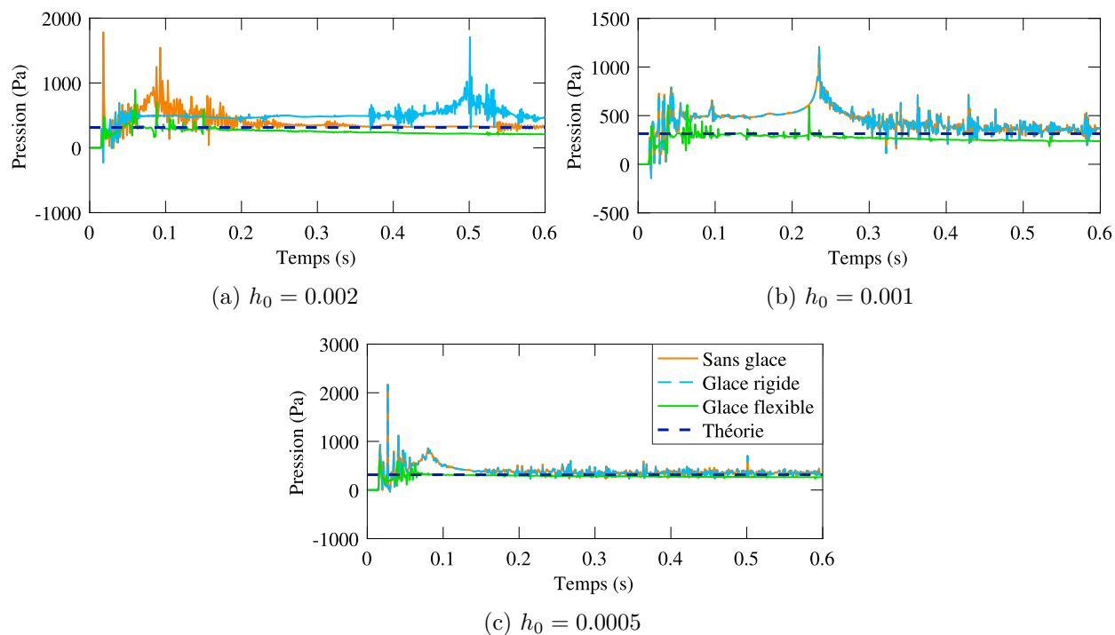
FIGURE 4.15 Comparaison de la pression à la base de la structure sans glace, avec glace rigide, flexible, selon plusieurs h_0
