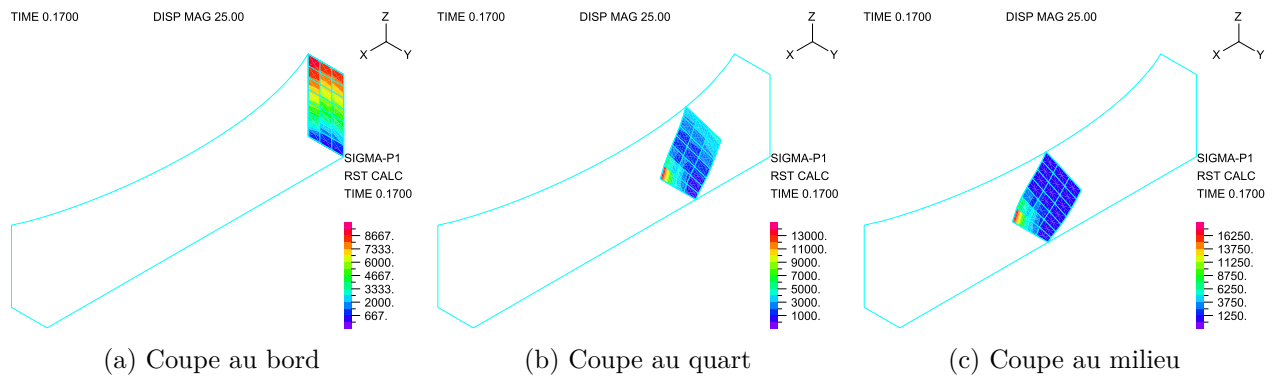
FIGURE 3.14 Coupes de contrainte principale maximale pour le maillage 4
