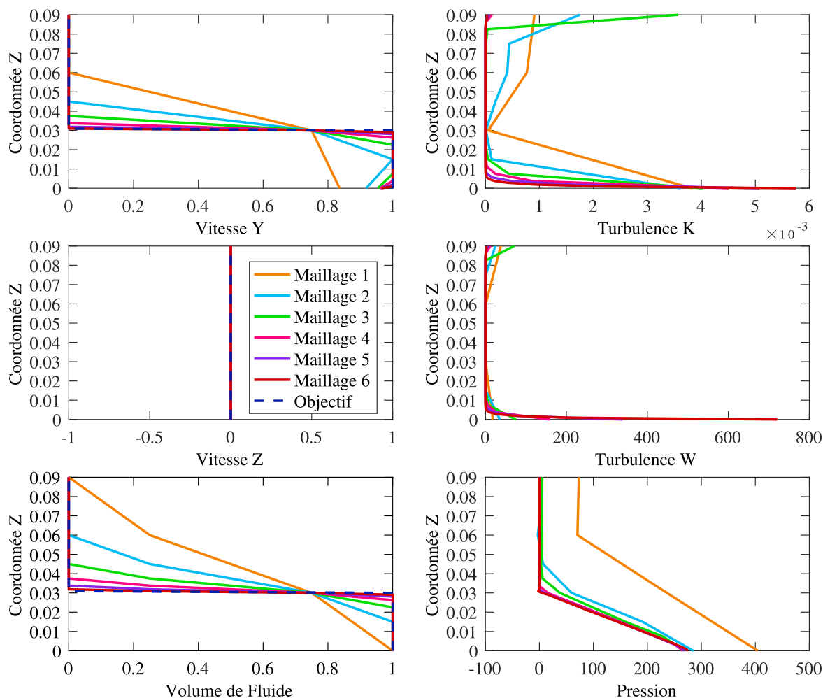
FIGURE 3.40 Comparaison des variables d'entrée et les valeurs considérées par la formulation FCBI-C, maillages 1a à 6a
