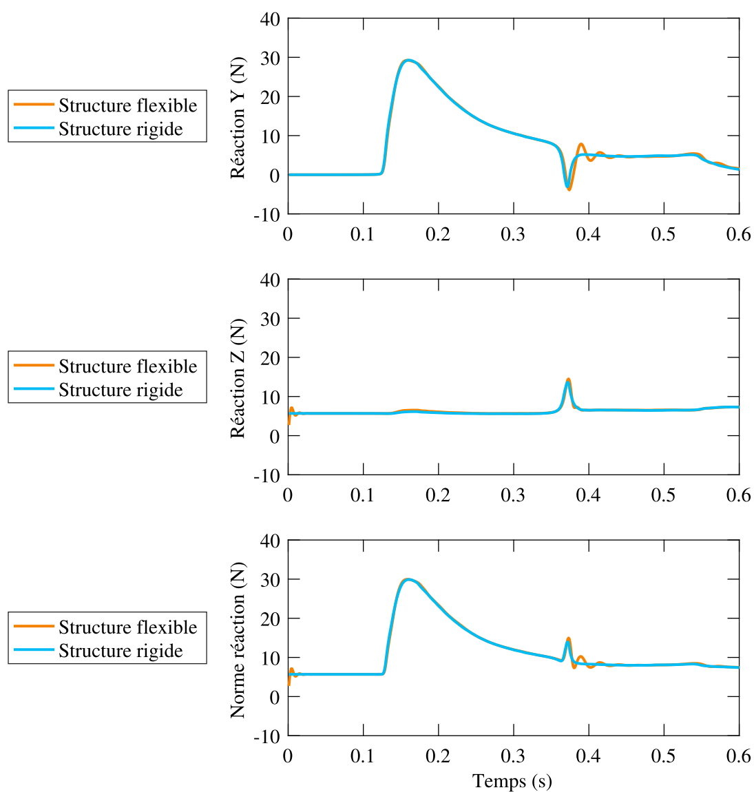
FIGURE 3.19 Réaction à la base des structures flexibles et rigides
