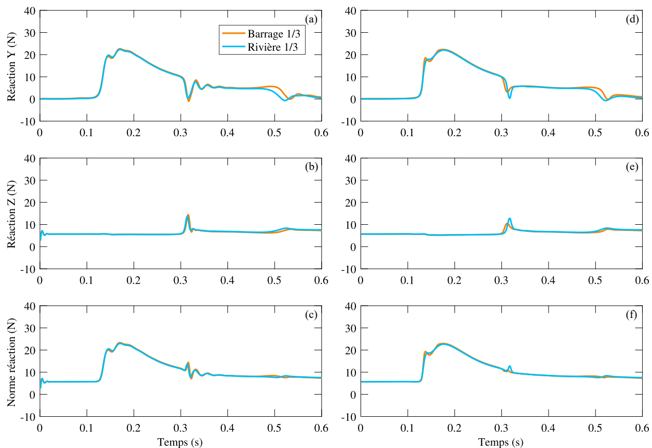
FIGURE 3.32 Réactions selon la configuration du lit d'eau pour de la structure flexible en (a) en Y, (b) en Z, (c) norme, de la structure rigide en (d) en Y, (e) en Z, (f) norme
