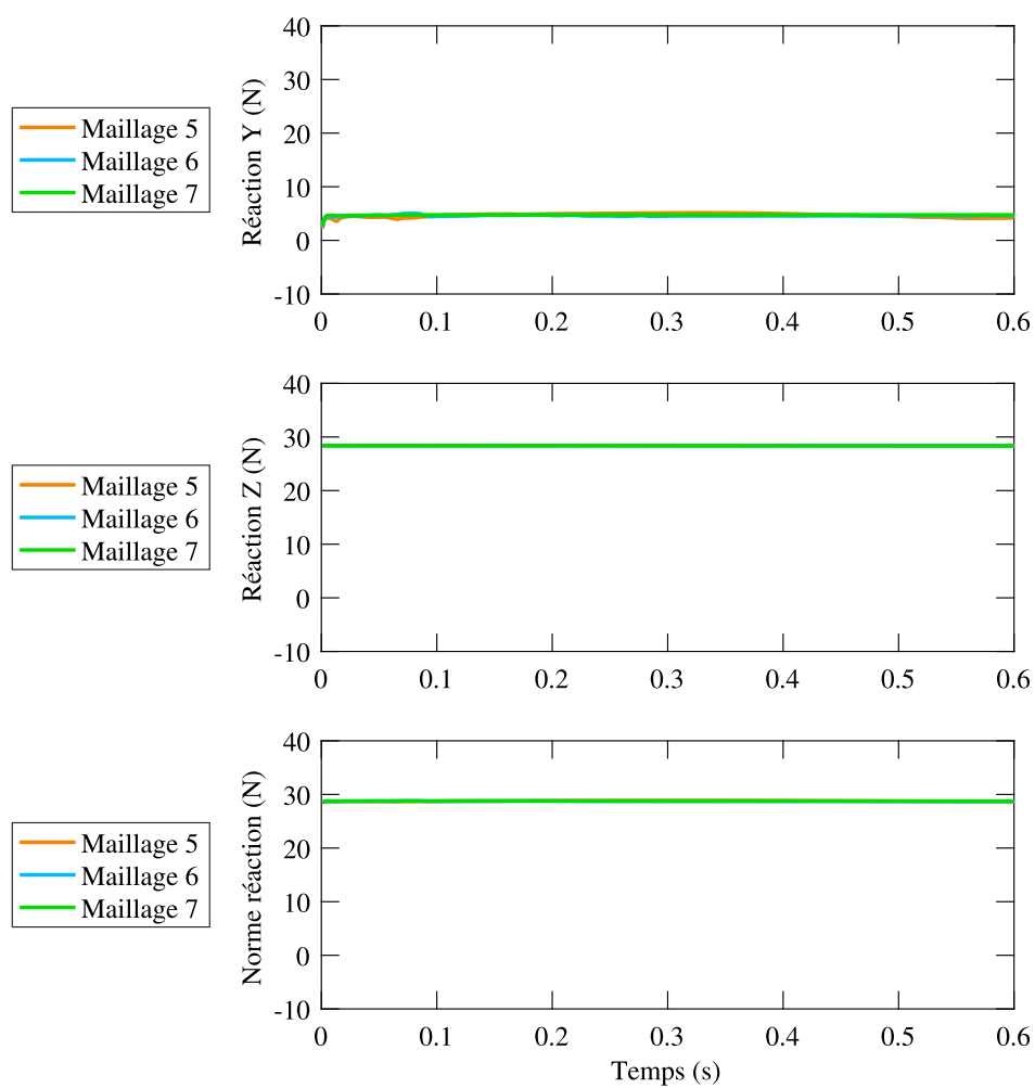
FIGURE 4.3 Réaction à la base de la structure selon plusieurs maillages
