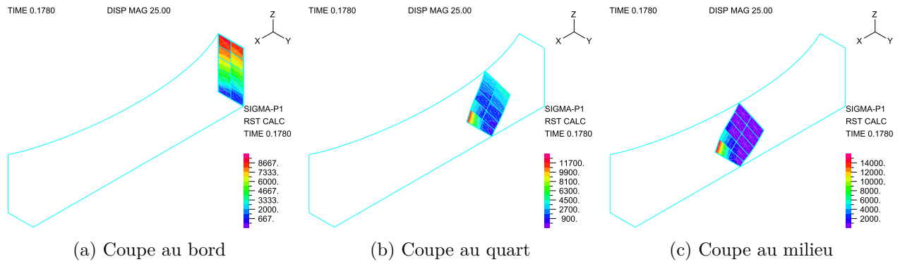
FIGURE 3.13 Coupes de contrainte principale maximale pour le maillage 3
