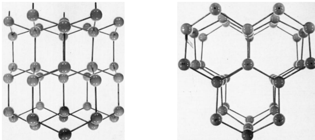
FIGURE 2.13 Arrangement des atomes d'oxygène dans la glace [16]
