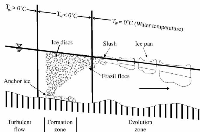
FIGURE 2.15 Étapes du développement de la glace fluviale [18]
