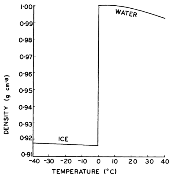
FIGURE 2.14 Densités de la glace et de l'eau saturée en air à la pression atmosphérique [17]
