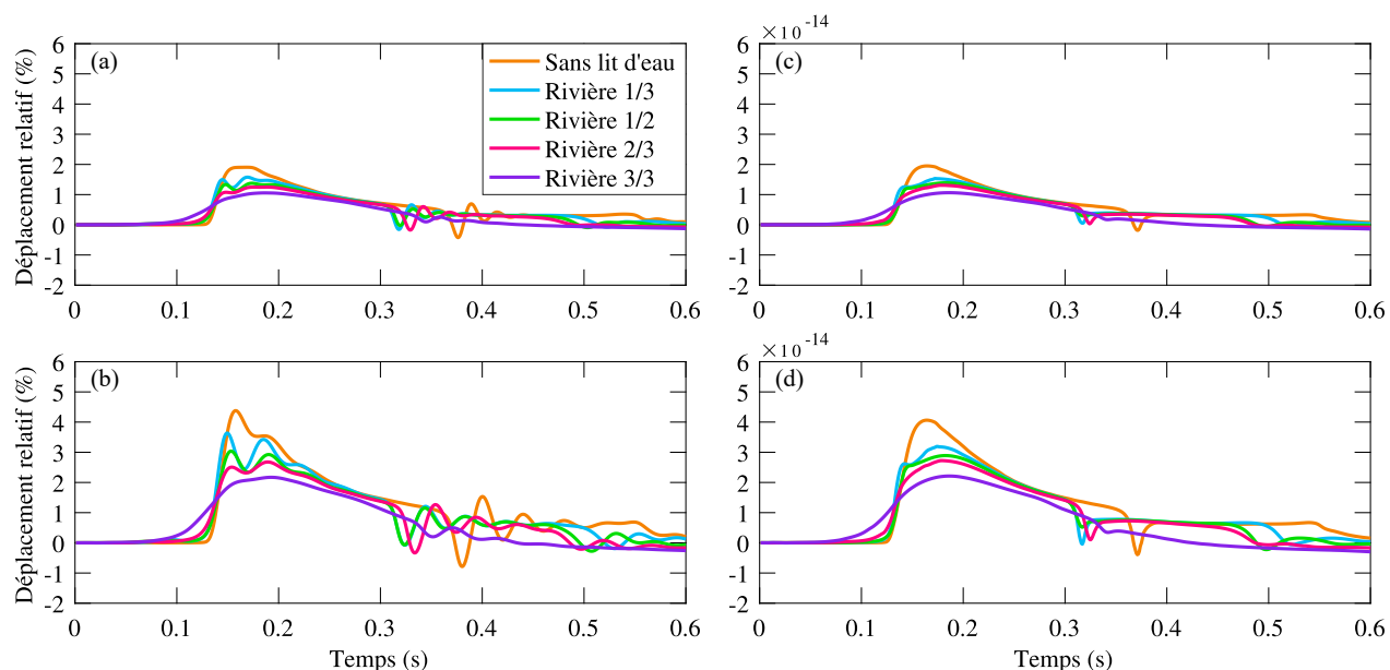
FIGURE 3.34 Déplacement relatif au sommet en amont de la structure flexible (a) avec bords fixes, (b) bords libres, pour la structure rigide (c) bords fixes, (d) bords libres en configuration rivière
