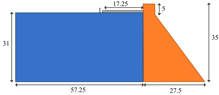
FIGURE 4.36 Dimensions du modèle préliminaire du barrage en taille réelle (m)
