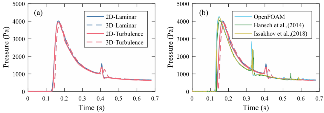
FIGURE 3.4 Comparaison de la pression au milieu de la structure sur la surface en amont (a) en 2D et 3D de Jianguo et al. (2024) [2] (b) résultats numériques de Hänsch et al. (2014) [25]; Isshakov et al. (2018) [26]; OpenFOAM
