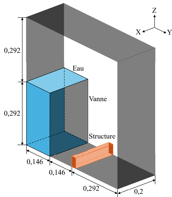
FIGURE 3.22 Schéma du cas de Koshizuka et al. [24] en 3D avec conditions aux bords
