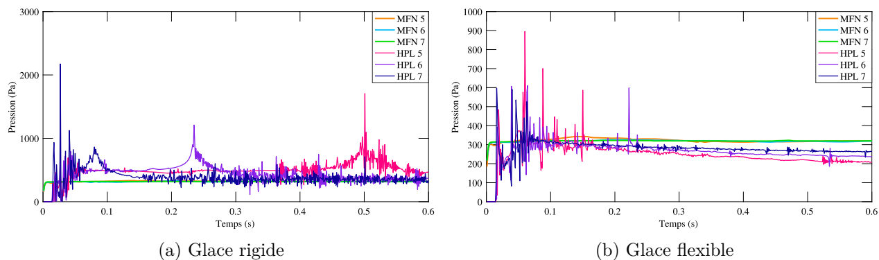
FIGURE 4.17 Comparaison de la pression à la base de la structure selon plusieurs maillages
