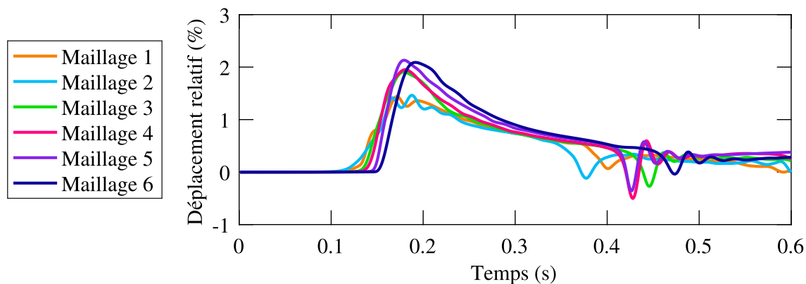
FIGURE 3.6 Déplacement relatif au sommet de la structure flexible en amont selon les maillages 1 à 6
