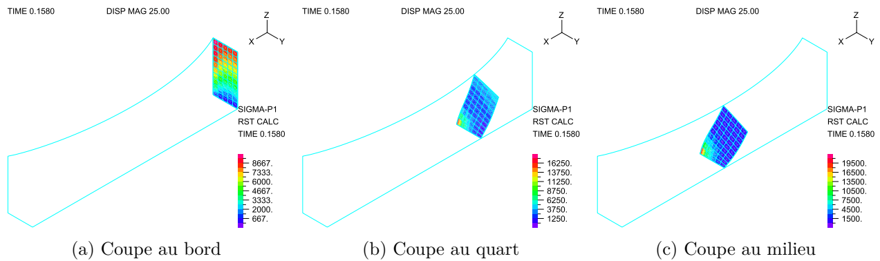
FIGURE 3.15 Coupes de contrainte principale maximale pour le maillage 5
