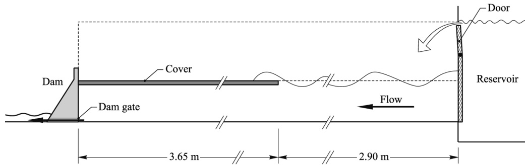
FIGURE 4.24 Coupe longitudinale du dispositif expérimental de Fuamba et al. (2007) [21]
