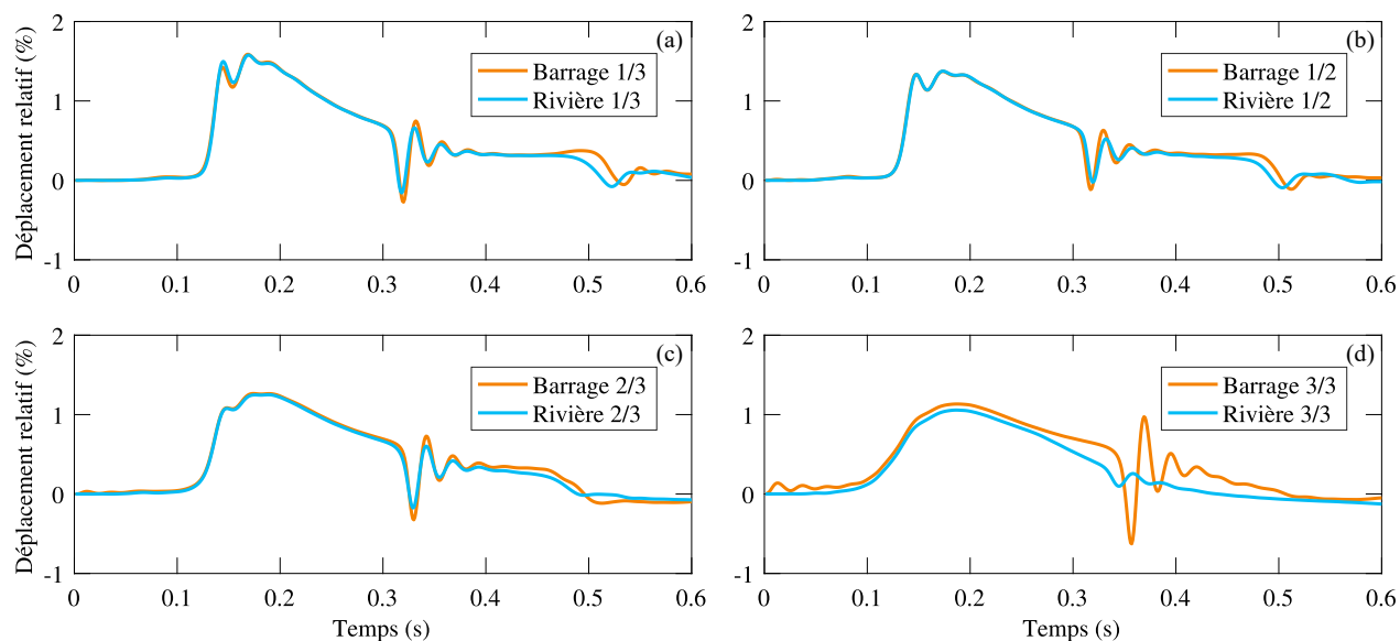
FIGURE 3.30 Déplacement relatif au sommet en amont de la structure flexible avec bords fixes pour un lit d'eau en configuration barrage pour les niveaux (a) 1/3, (b) 1/2, (c) 2/3, (d) 3/3
