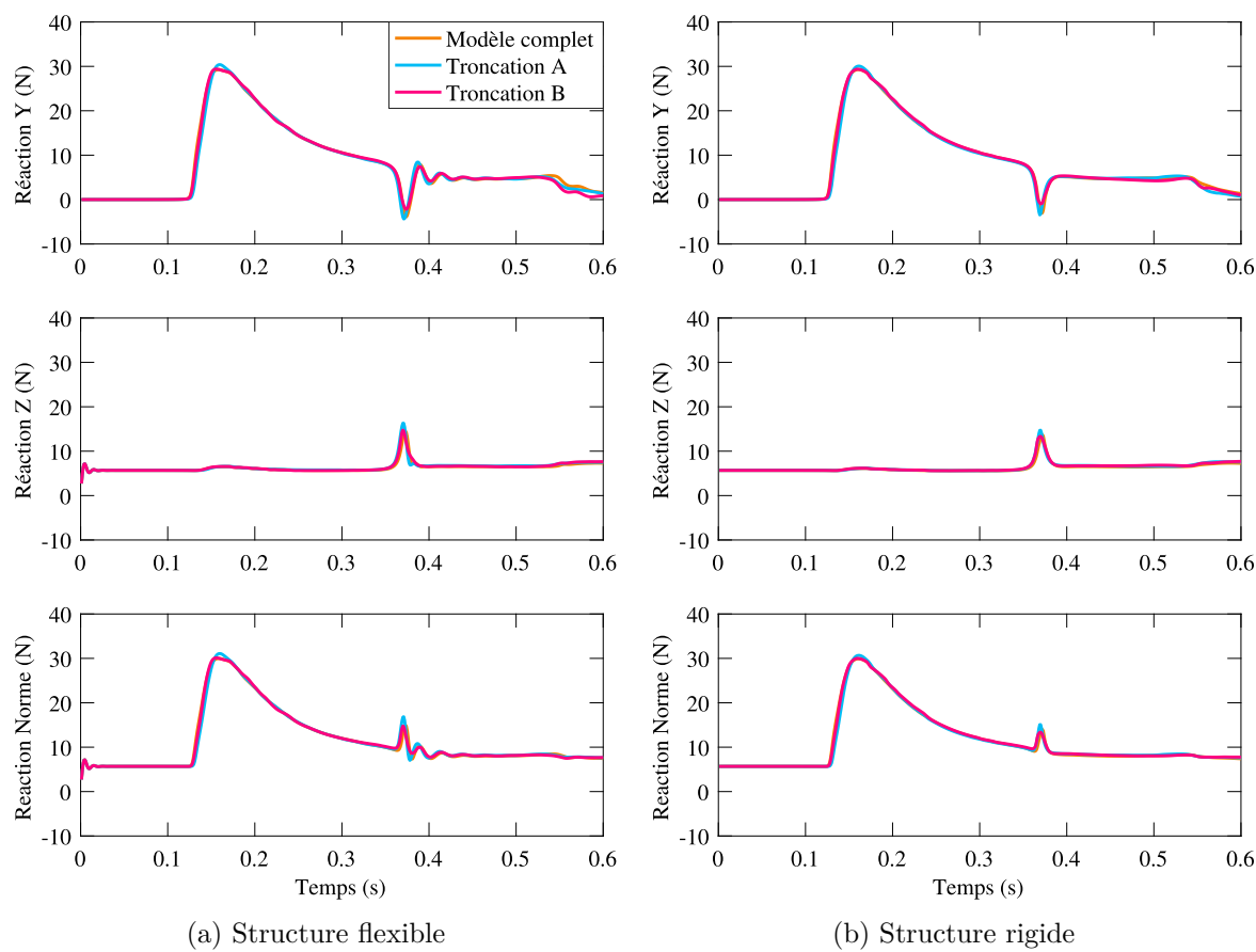
FIGURE 3.48 Comparaison de la réaction à la base des modèles complet, troncation A et troncation B
