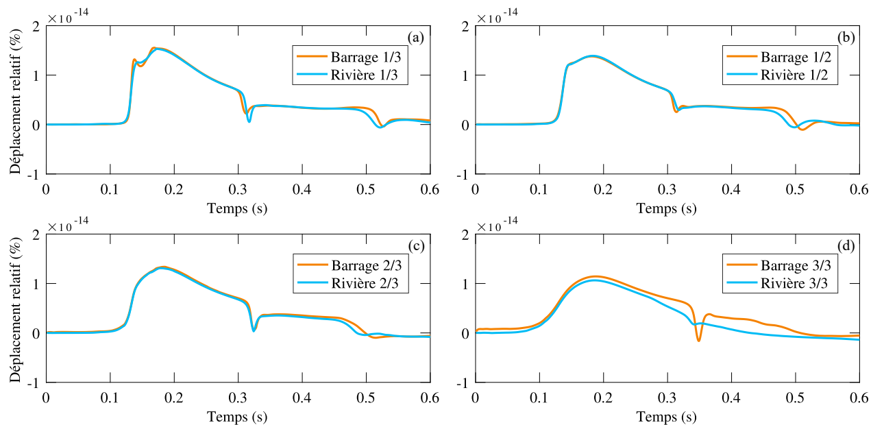
FIGURE 3.31 Déplacement relatif au sommet en amont de la structure rigide avec bords fixes pour un lit d'eau en configuration barrage pour les niveaux (a) 1/3, (b) 1/2, (c) 2/3, (d) 3/3
