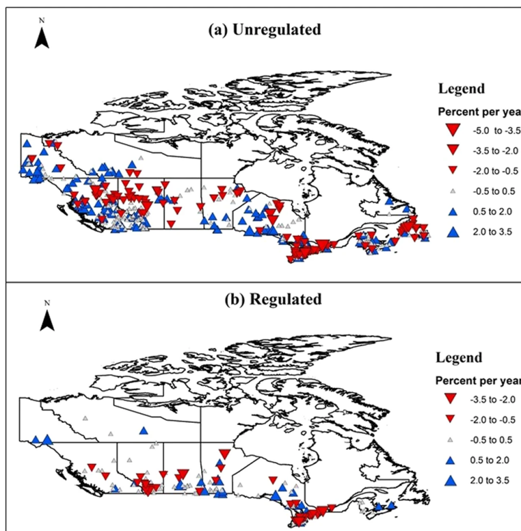
FIGURE 2.12 Tendances observées des débits de pointe des crues dues aux embâcles de 1903 à 2015. Le triangle rouge descendant (valeurs négatives) indique une diminution de l'ampleur (en pourcentage par an), tandis que le triangle bleu ascendant (valeurs positives) représente une augmentation de l'ampleur (en pourcentage par an) des embâcles. La taille du triangle est proportionnelle à l'ampleur de la tendance. [13]
