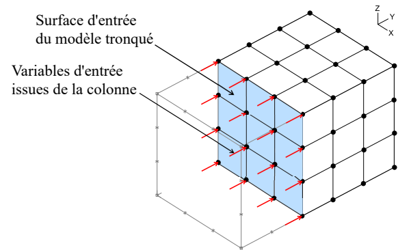
(b) Application des variables de fluide sur le modèle tronqué, maillage 1a
