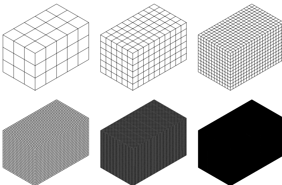
FIGURE 3.37 Définition des maillages 1a à 6a
