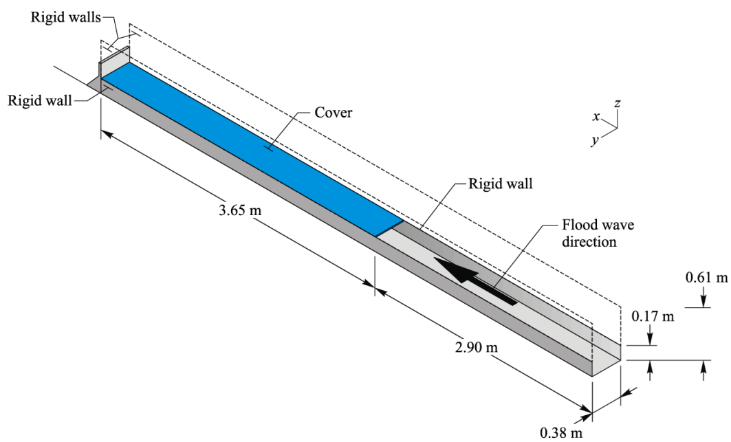
FIGURE 4.25 Dispositif expérimental de Fuamba et al. (2007) [21]
