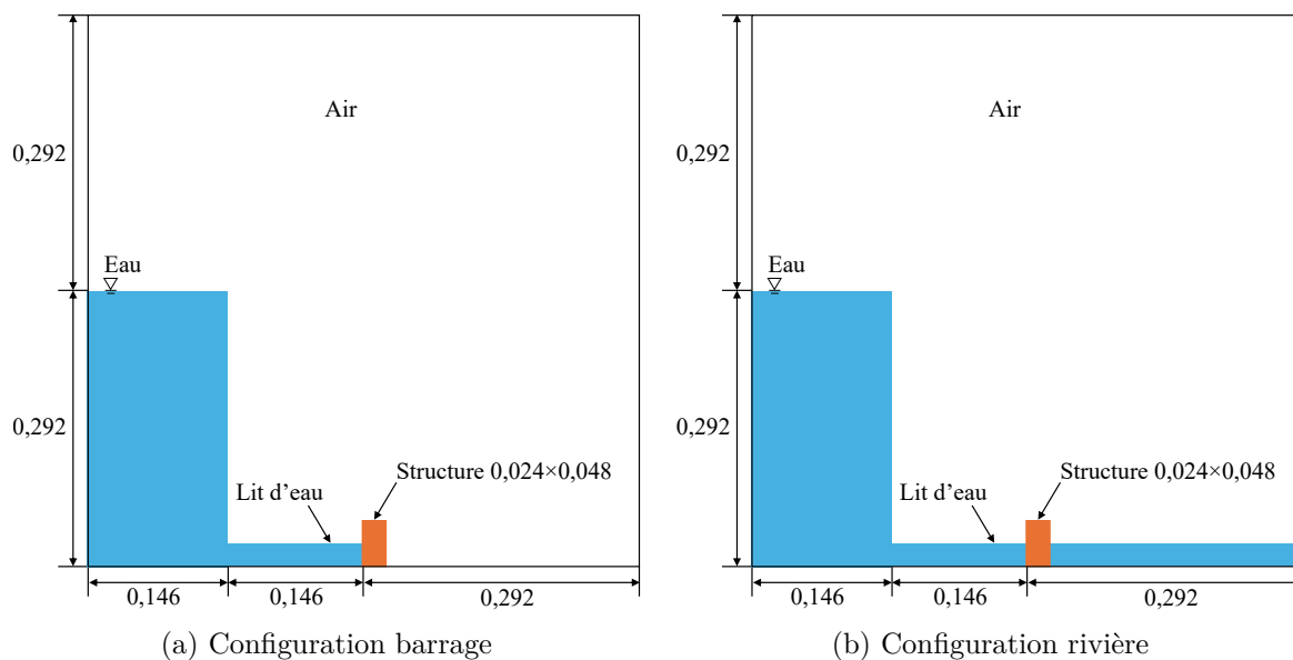
FIGURE 3.28 Modèle avec lit d'eau pour différentes hauteurs en m
