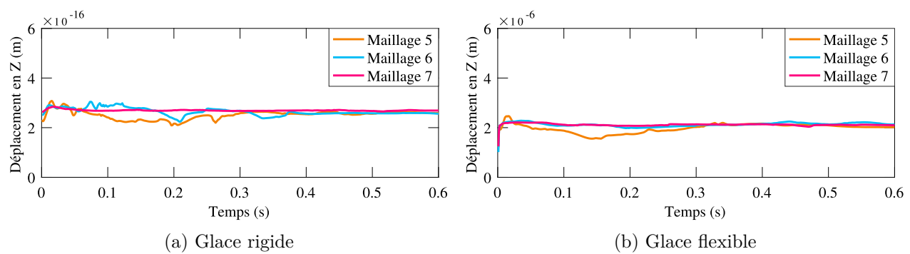
FIGURE 4.12 Comparaison du déplacement du couvert de glace selon Z selon plusieurs maillages
