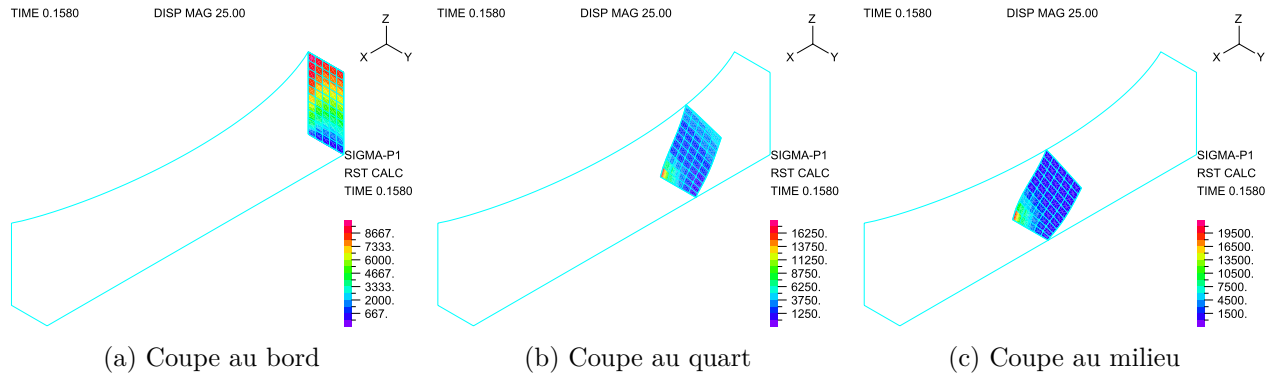
FIGURE 3.20 Coupes de contrainte principale maximale de la structure flexible
