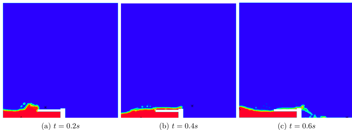
FIGURE 4.21 Écoulement de l'eau en MFN sur plusieurs pas de temps
