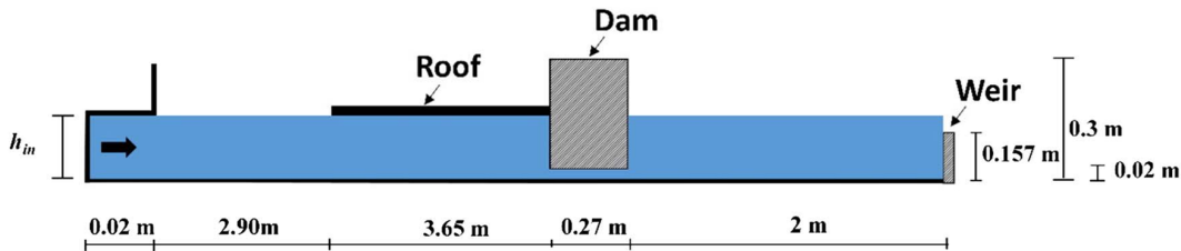
FIGURE 4.27 Modèle de Nomeritae et al. (2018) [27] avec conditions initiales
