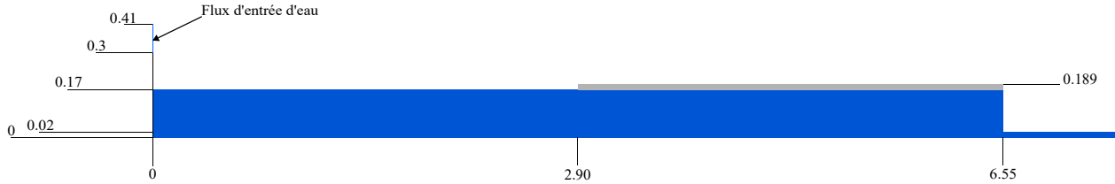
FIGURE 4.33 Dimensions du canal avec la glace
