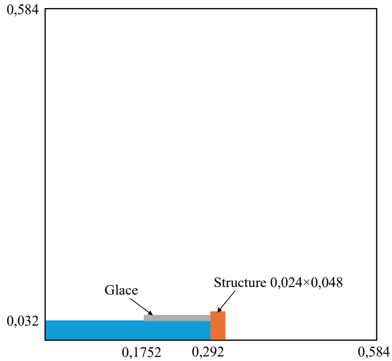
FIGURE 4.6 Cas avec un couvert de glace
