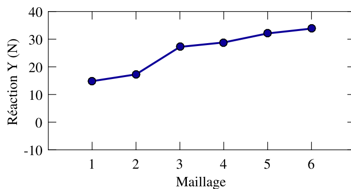
FIGURE 3.9 Réaction Y maximale à la base de la structure flexible selon les maillages 1 à 6
