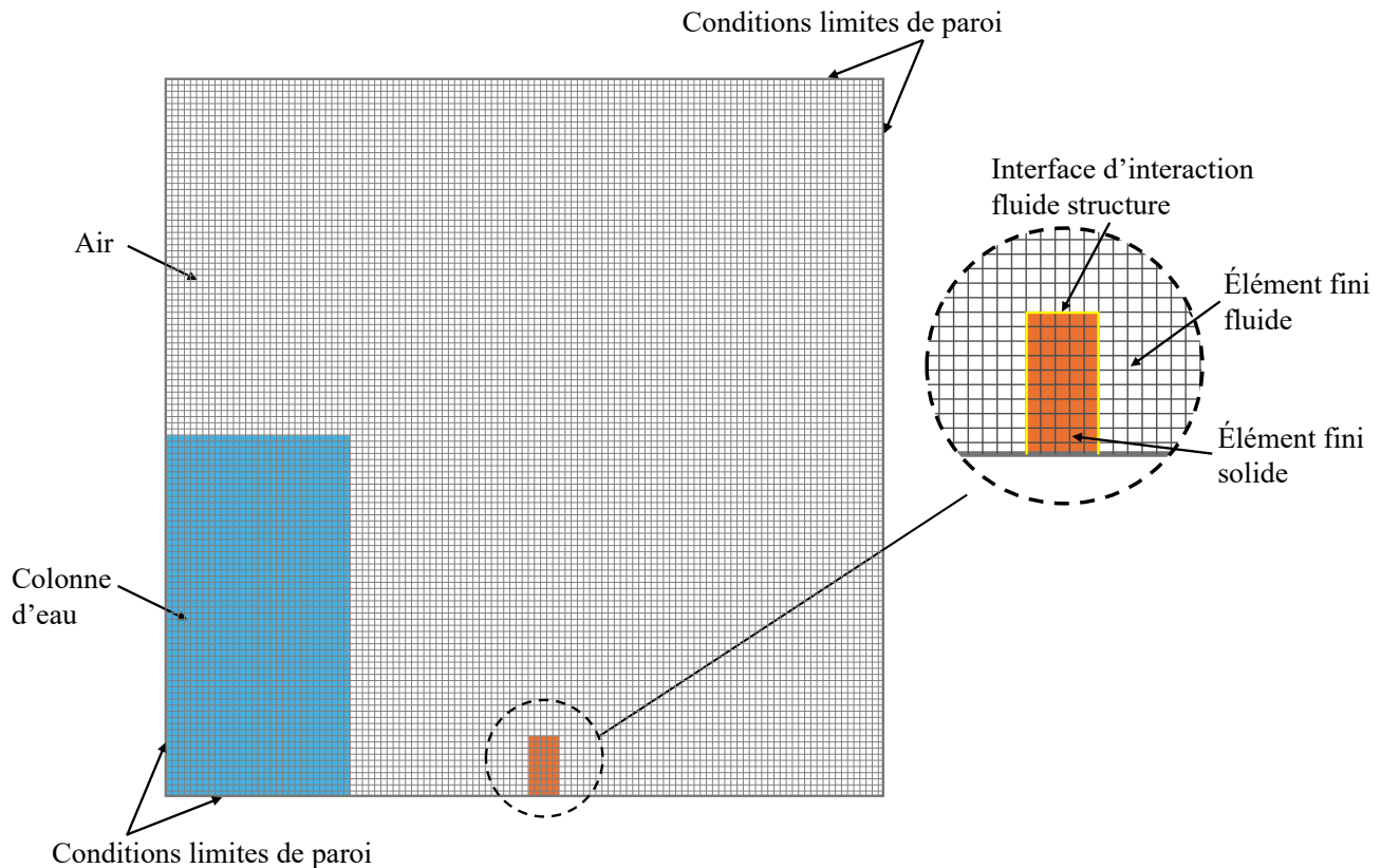
FIGURE 3.3 Schéma du modèle éléments finis (Adapté d'une communication personnelle de Bouaanani (2024))
