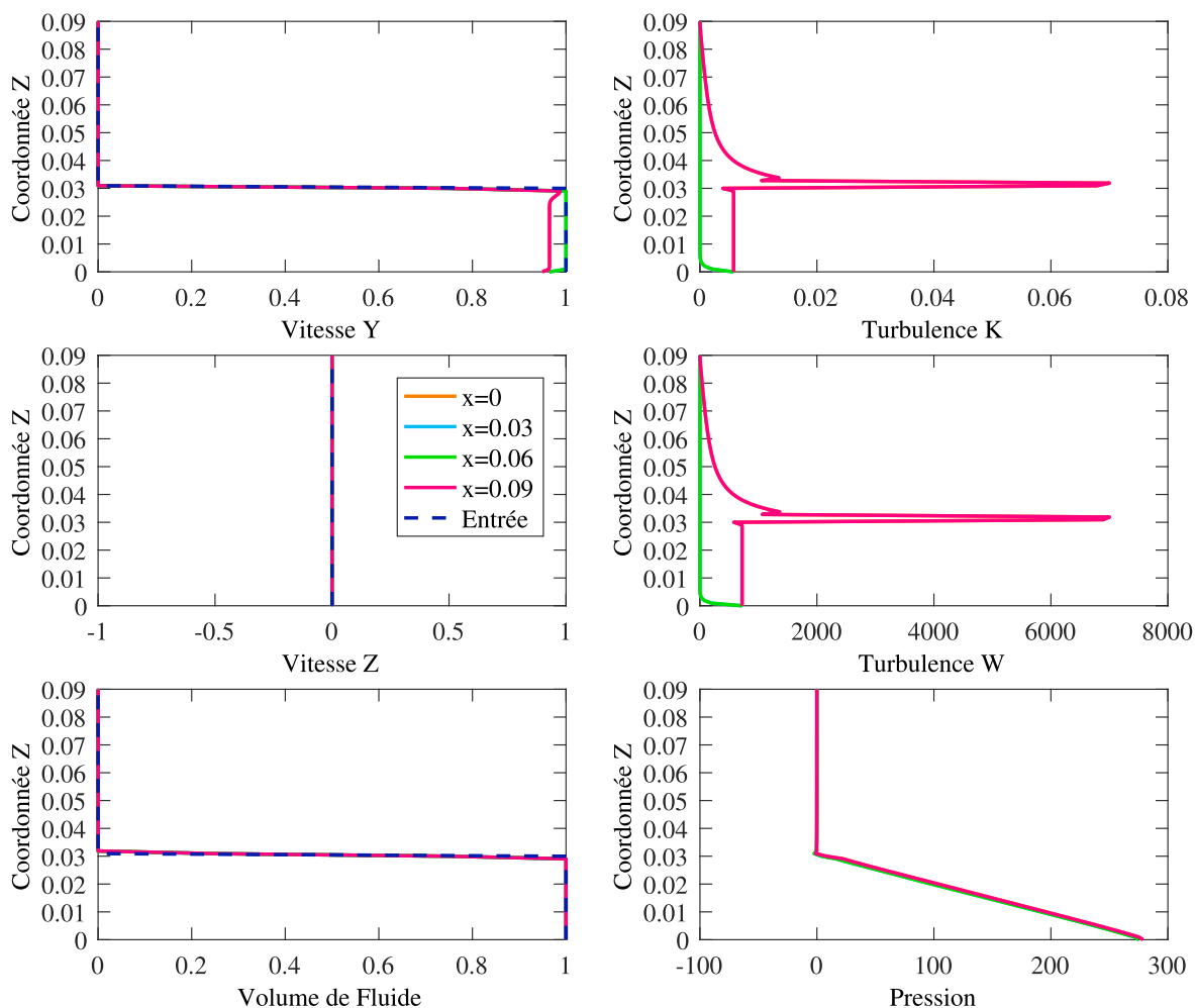
FIGURE 3.39 Comparaison des variables d'entrée et les valeurs considérées par la formulation FCBI-C, maillage 6a
