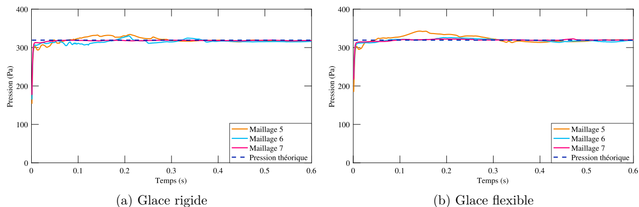
FIGURE 4.8 Comparaison de la pression à la base de la structure selon plusieurs maillages
