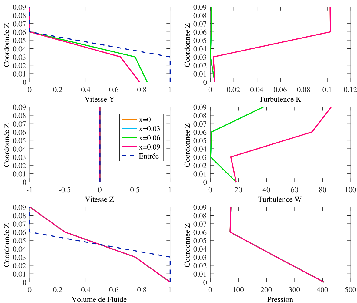
FIGURE 3.38 Comparaison des variables d'entrée et les valeurs considérées par la formulation FCBI-C, maillage 1a
