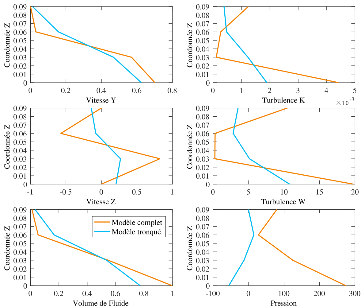
FIGURE 3.43 Comparaison des variables d'entrée et les valeurs considérées par la formulation FCBI-C à la surface de troncation à x = 0.03 , maillage 1a
