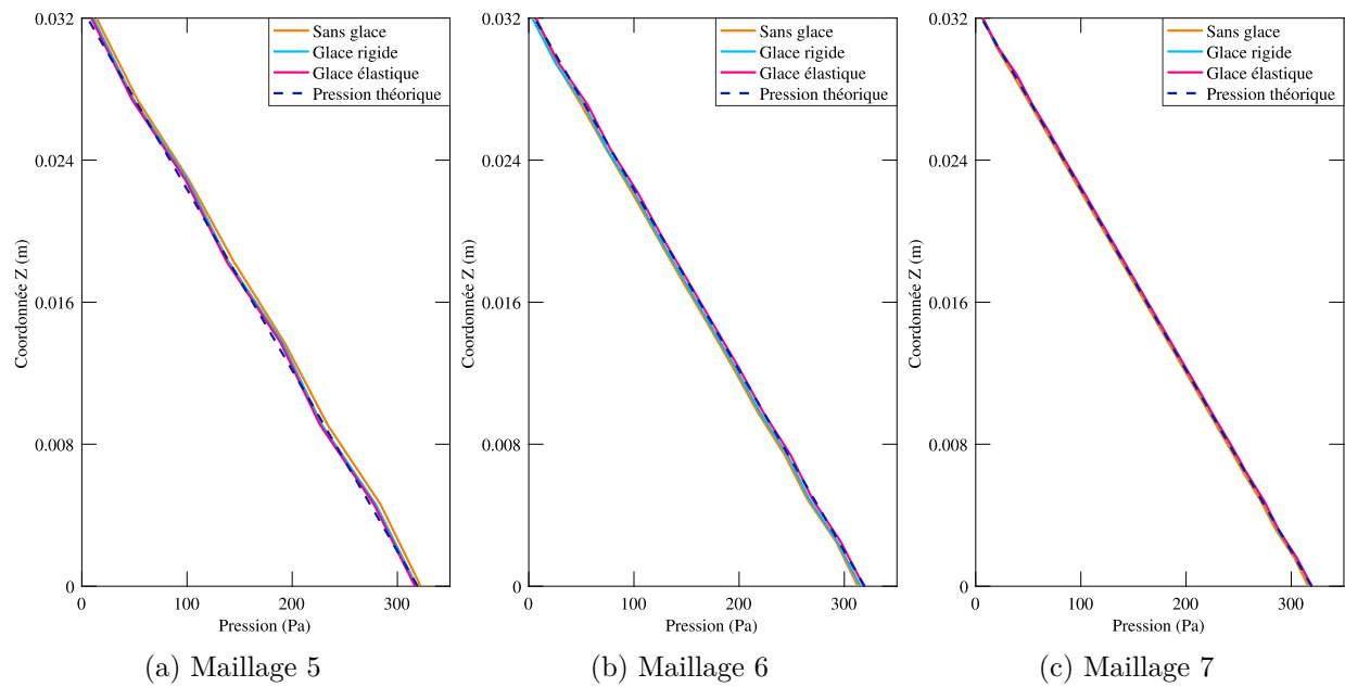
FIGURE 4.11 Triangle de pression le long de la structure avec glace rigide, flexible, et sans glace, à 0.5s
