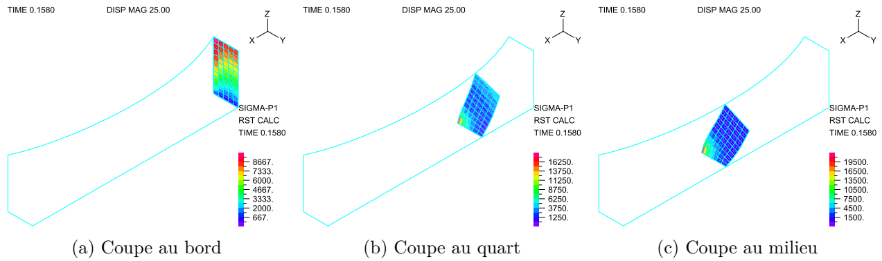
FIGURE 3.26 Coupes de contrainte principale maximale de la structure flexible avec bords fixes pour le maillage 5
