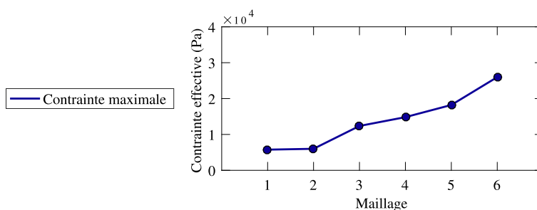
FIGURE 3.17 Contrainte principale maximale pour les maillages 1 à 6
