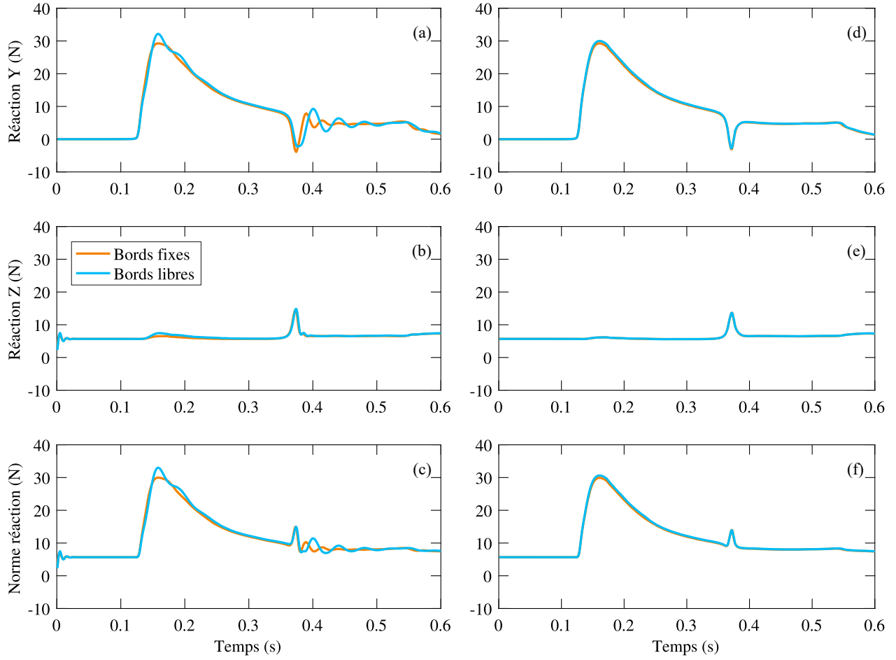
FIGURE 3.25 Réactions selon les conditions de bord pour de la structure flexible en (a) en Y, (b) en Z, (c) norme, de la structure rigide en (d) en Y, (e) en Z, (f) norme
