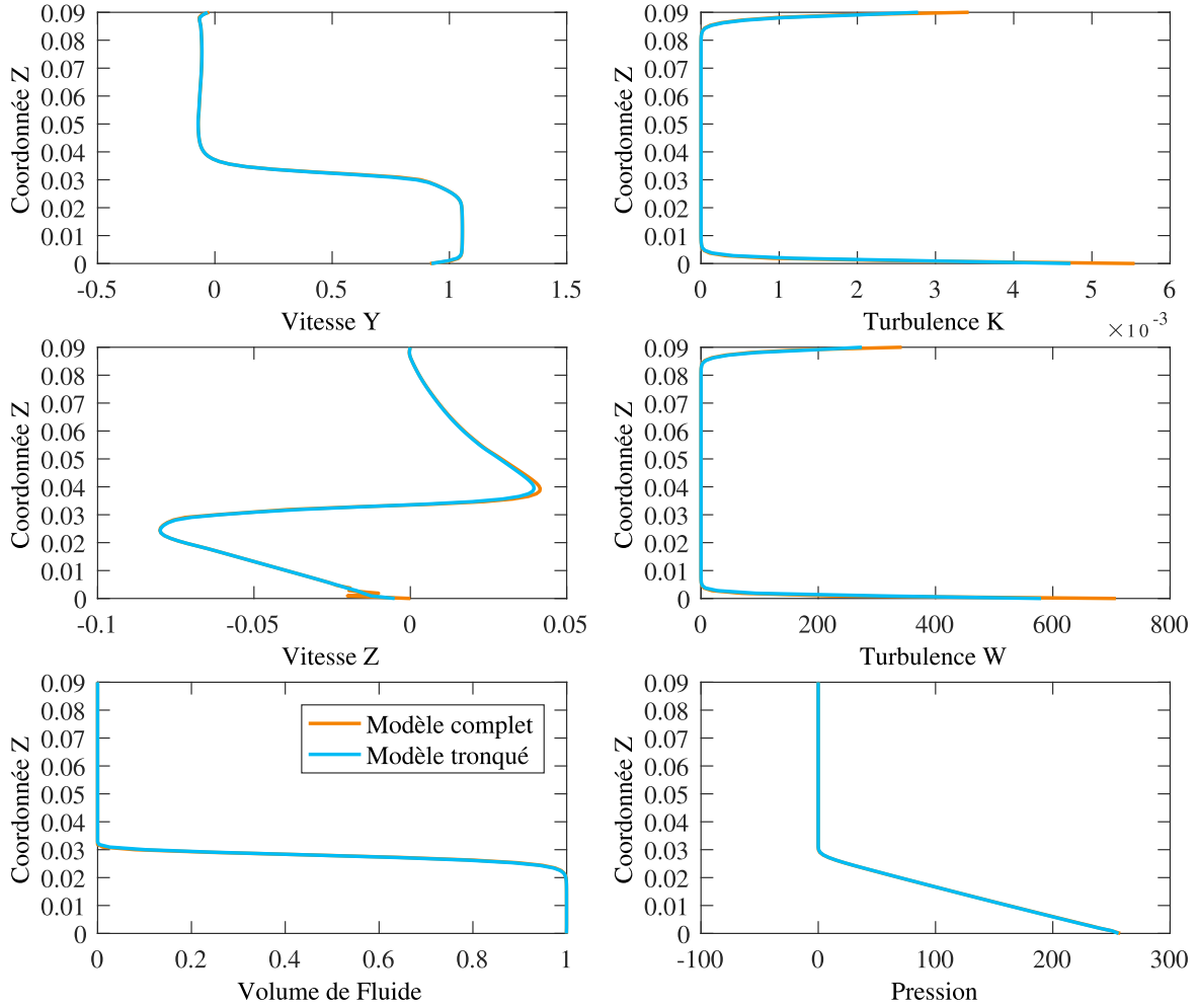
FIGURE 3.44 Comparaison des variables d'entrée et les valeurs considérées par la formulation FCBI-C à la surface de troncation à x = 0.03 , maillage 6a
