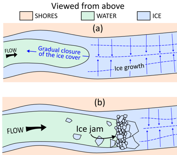
FIGURE 2.16 Formation d'un couvert de glace uniforme [19]
