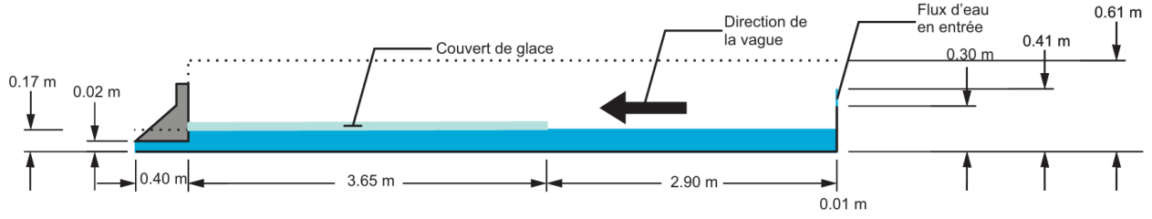
FIGURE 4.28 Modèle de Knuchel et al. (2021) [28] avec conditions initiales
