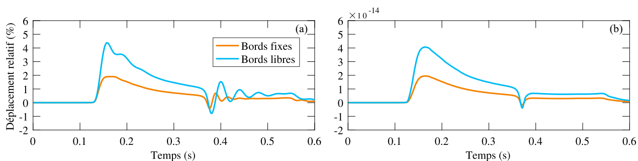
FIGURE 3.24 Déplacement relatif en fonction des conditions de bords pour les structures (a) flexible et (b) rigide
