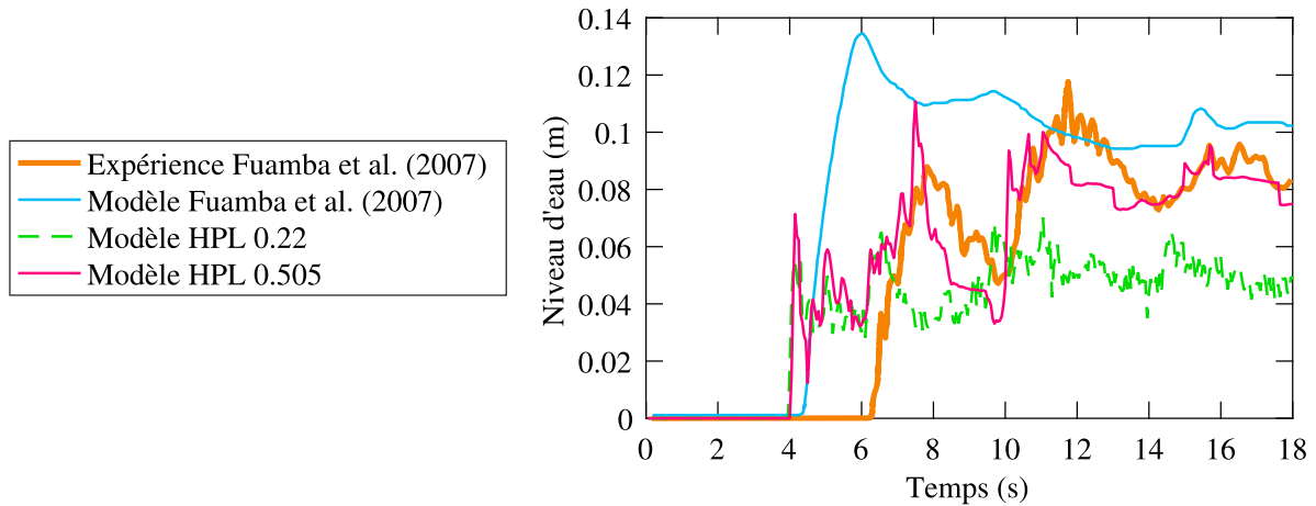
FIGURE 4.34 Hauteur d'eau avec glace au niveau de la structure au dessus du couvert, avec des structures de 0.22 et 0.505 m de haut
