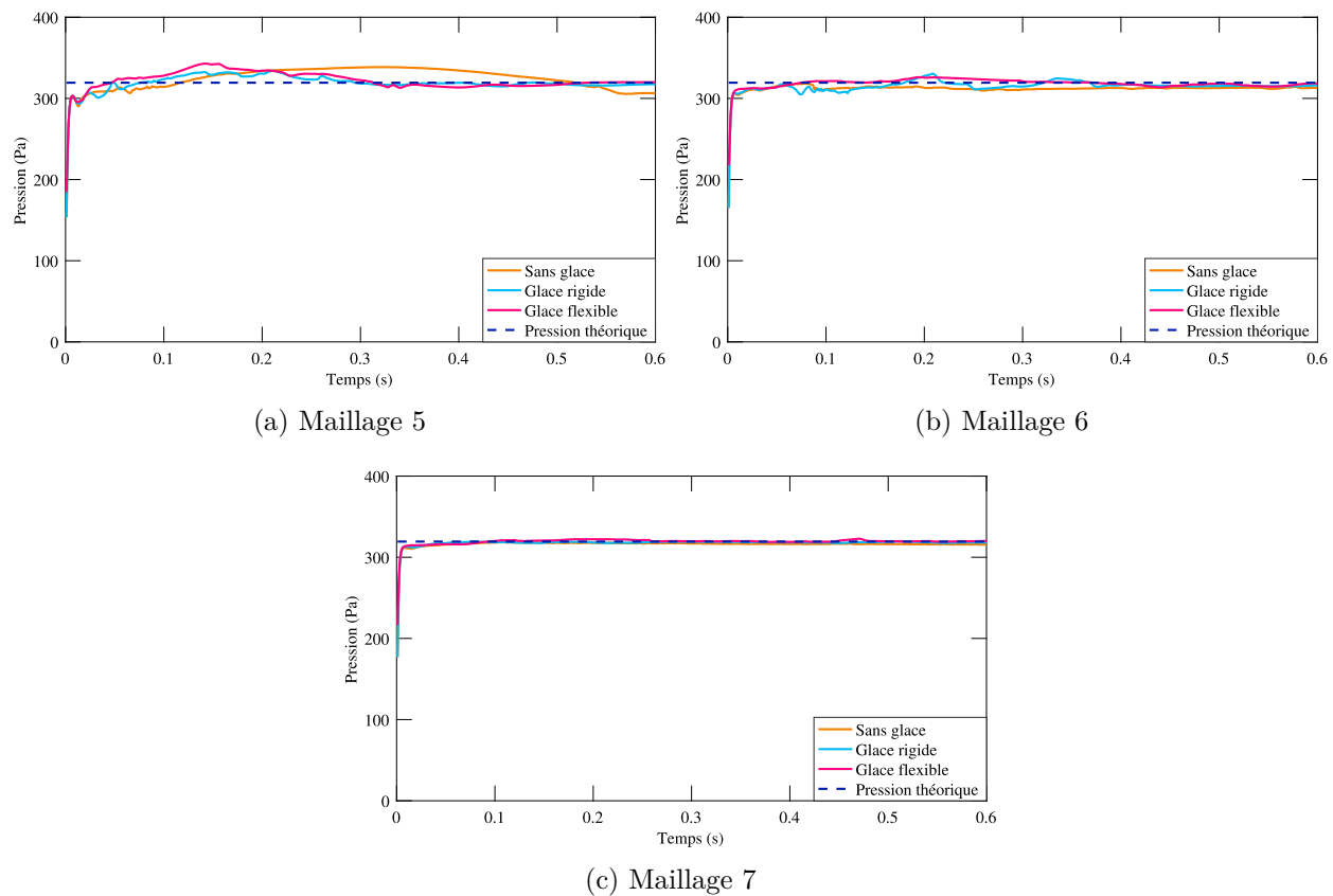
FIGURE 4.10 Comparaison de la pression à la base de la structure sans glace, avec glace rigide, flexible, selon plusieurs maillages
