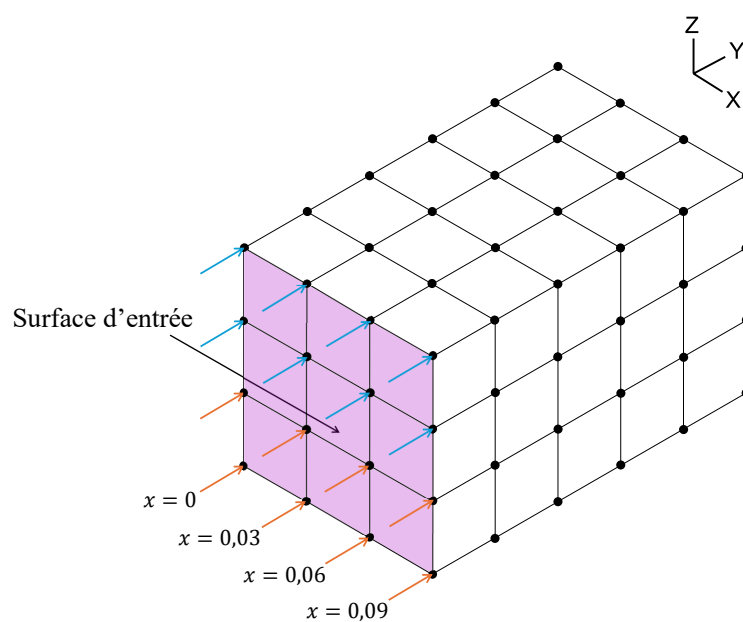
FIGURE 3.36 Définition des variables d'entrée à la surface d'entrée (en violet)
