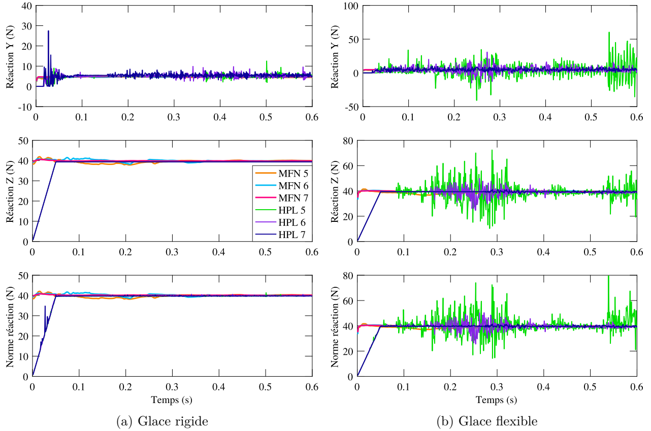
FIGURE 4.18 Comparaison de la réaction à la base de la structure selon plusieurs maillages
