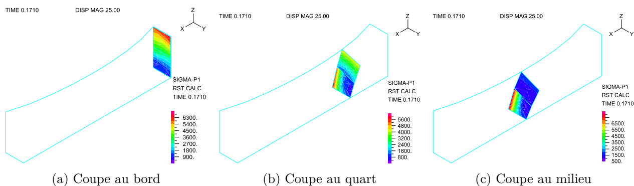
FIGURE 3.11 Coupes de contrainte principale maximale pour le maillage 1
