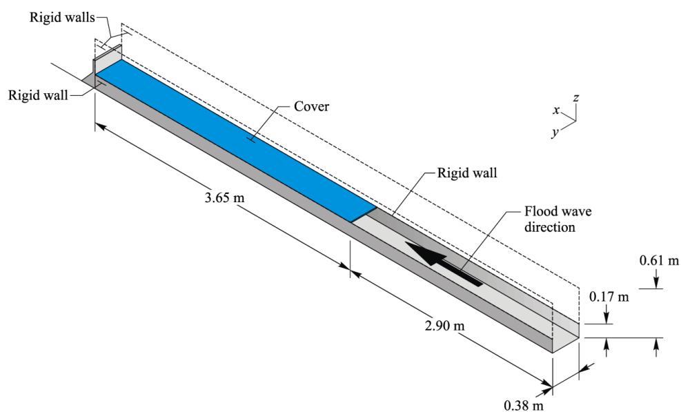
FIGURE 2.18 Dispositif expérimental pour l'étude de l'impact d'un couvert de glace rigide. [21]
