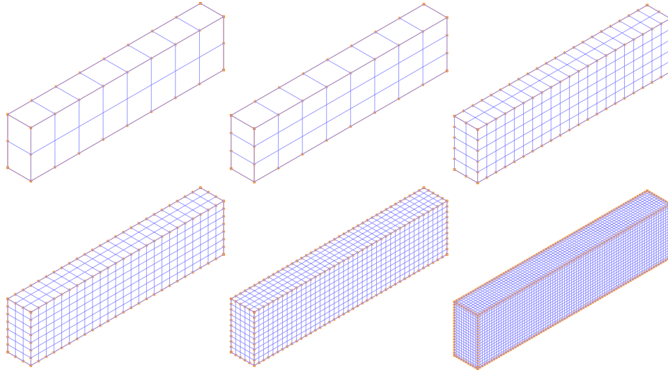
FIGURE 3.5 Structure avec maillage de 1 à 6
