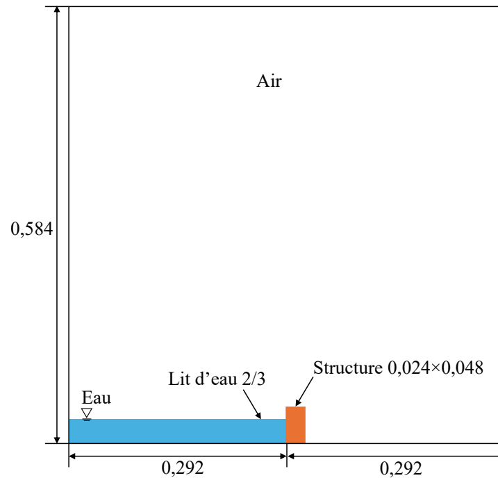
FIGURE 4.1 Cas statique avec lit d'eau au niveau 2/3 en configuration barrage
