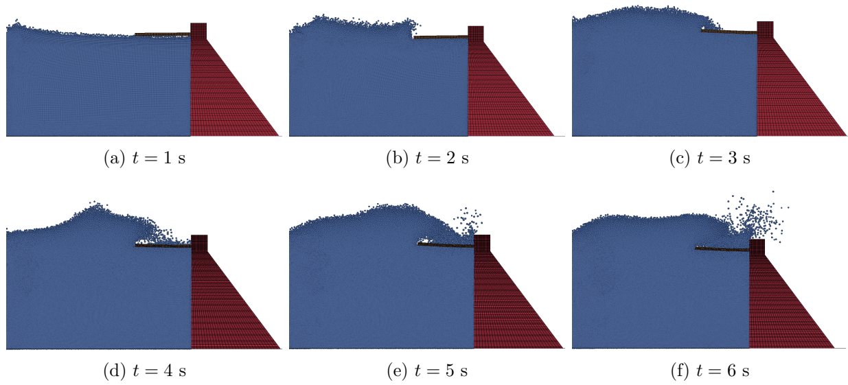
FIGURE 4.39 Ecoulement de l'eau en HPL sur plusieurs pas de temps
