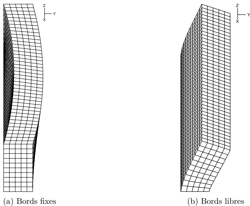
FIGURE 3.23 Cas avec structure flexible selon différentes conditions de bords à t = 0.15 s avec un facteur d'amplification de 10
