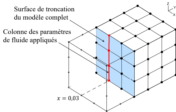
(a) Définition des paramètres appliqués provenant du modèle complet, maillage 1a
