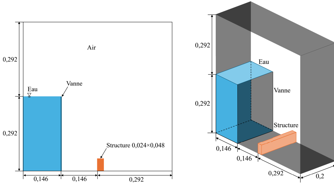
FIGURE 3.1 Dimensions (m) du dispositif expérimental de Koshizuka et al. (1995) [24]
