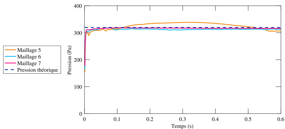
FIGURE 4.2 Pression à la base de la structure selon plusieurs maillages
