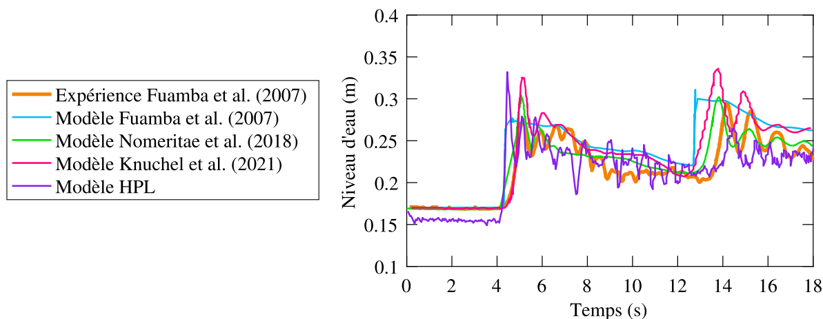
FIGURE 4.32 Hauteur d'eau sans glace au niveau de la structure, avec une structure de 0.22 m
