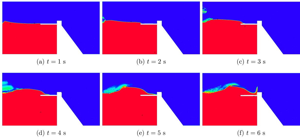
FIGURE 4.38 Ecoulement de l'eau en MFN sur plusieurs pas de temps
