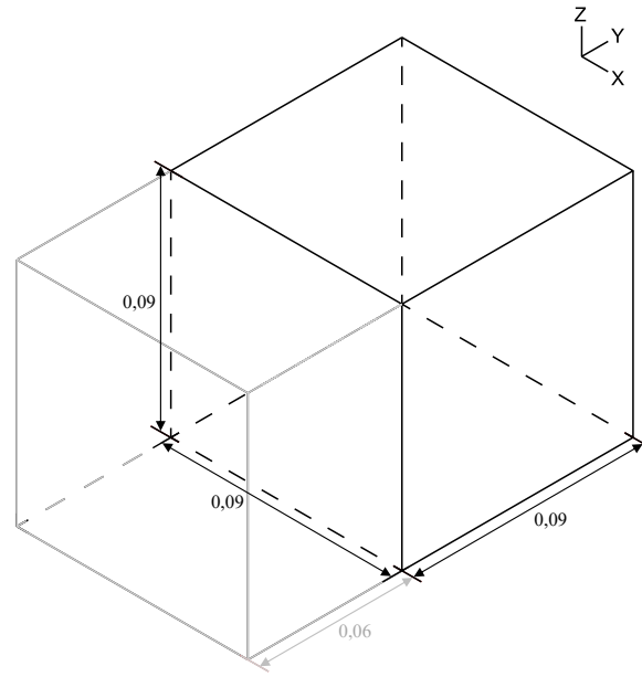
FIGURE 3.41 Dimensions du modèle 3D tronqué en (m)
