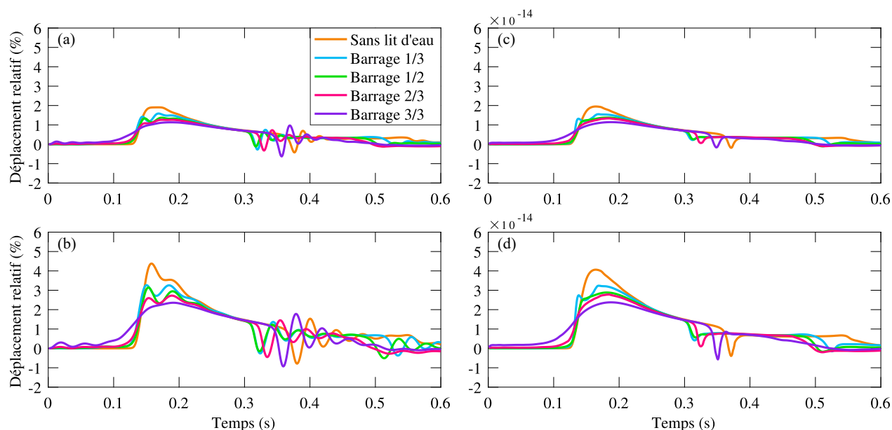
FIGURE 3.33 Déplacement relatif au sommet en amont de la structure flexible (a) avec bords fixes, (b) bords libres, pour la structure rigide (c) bords fixes, (d) bords libres en configuration barrage
