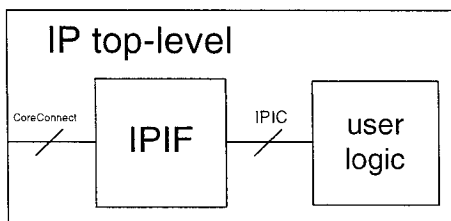
Figure 3.4 Structure d'un patron d'IP utilisant IPIF
