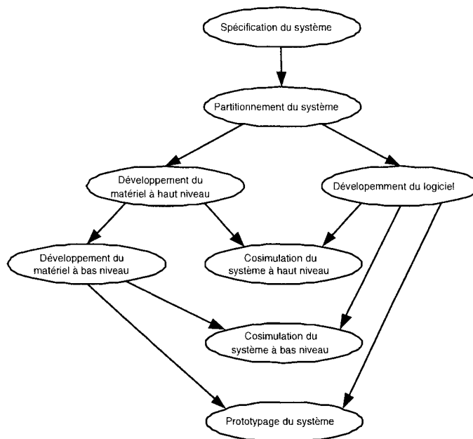
Figure 1.9 Flot de conception pour FPGA plateforme avec cosimulation
