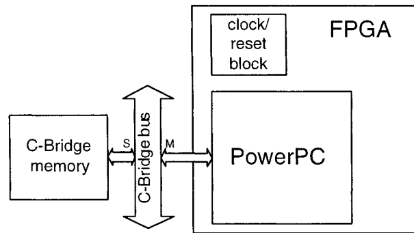
Figure 3.1 Design utilisé pour le test du PSP
