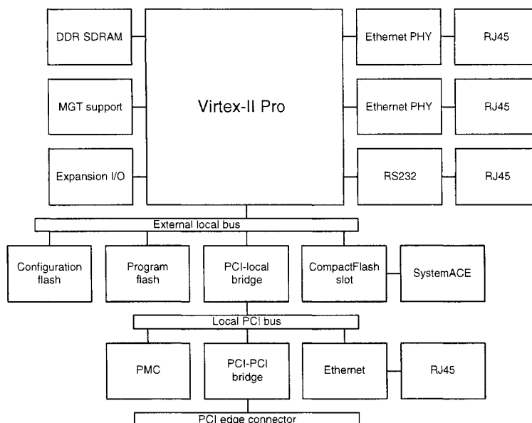
Figure 2.1 Schéma blocs de la carte AP100
