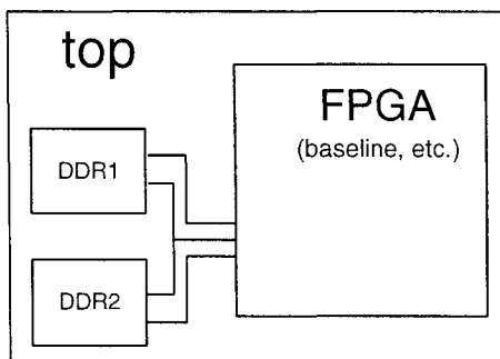
Figure 3.3 Modèle top-level avec mémoire externe
