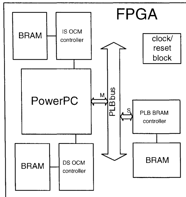
Figure 3.2 Schéma blocs du premier design créé dans XPS
