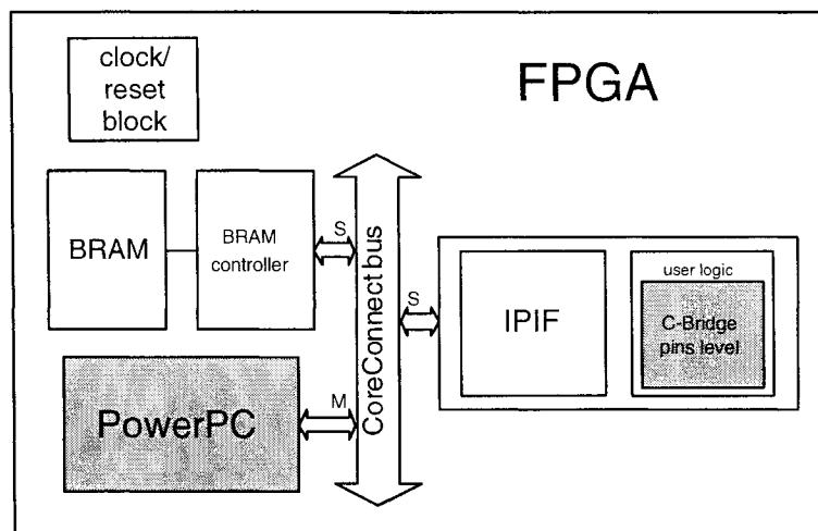
Figure 3.7 Principe de fonctionnement d'un module IPIF+C-Bridge
