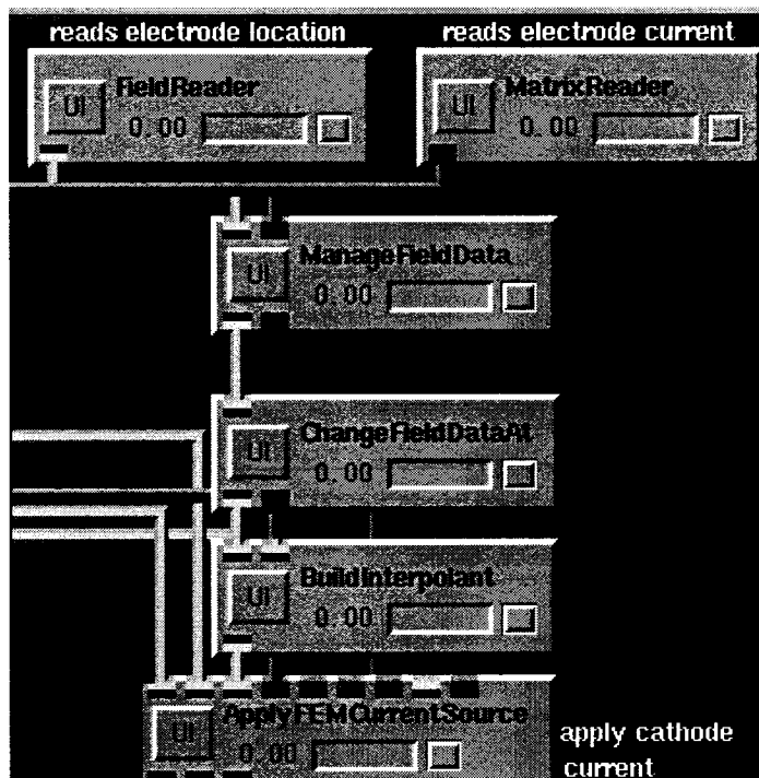
Figure 4-6 : Blocs et connexions nécessaires pour la cathode et l'amplitude du courant
