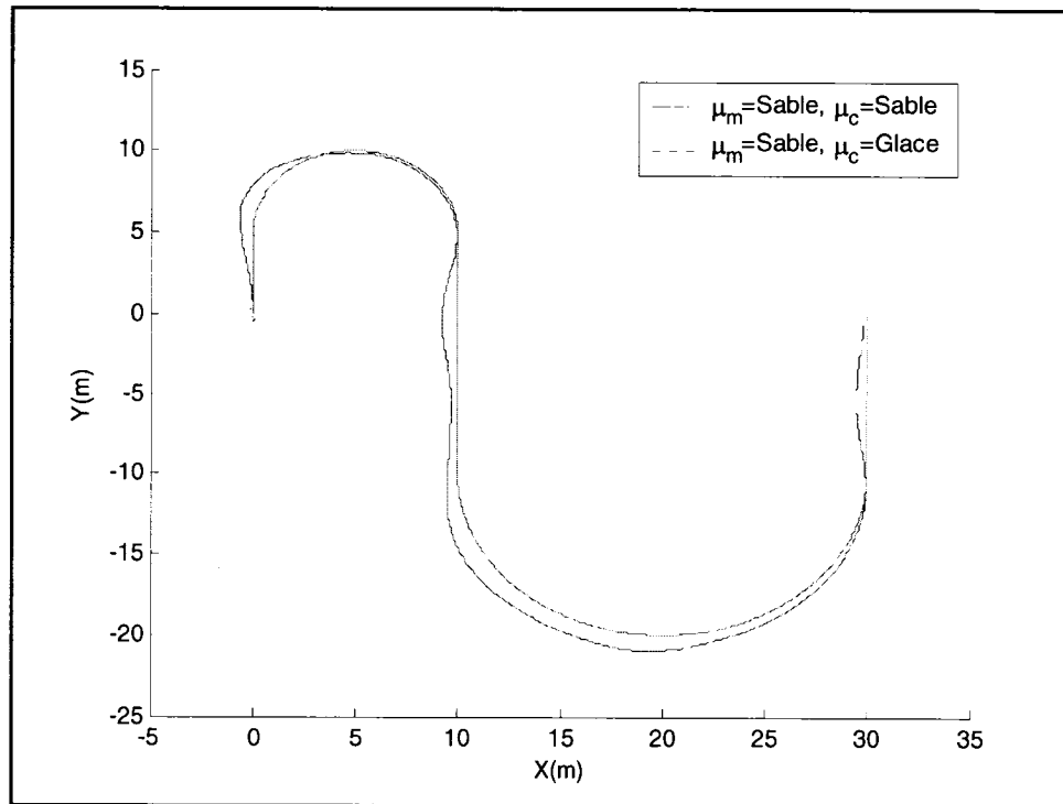
Figure 5.38 : Suivi de chemin avec adhérence du modèle différent de l'adhérence du contrôleur ( \mu_m=\text{Sable} , \mu_c=\text{Glace} )
