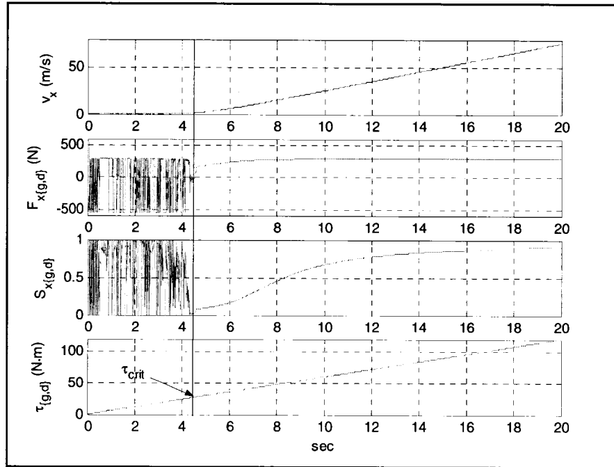
Figure 5.42 : Exemple d'essai pratique en boucle ouverte pour estimer les paramètres du sol
