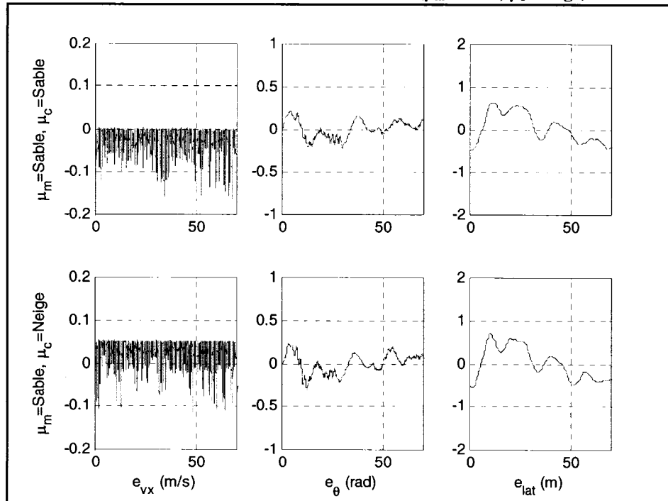
Figure 5.31 : Erreurs de suivi de chemin pour une adhérence du modèle différente de l'adhérence du contrôleur ( \mu_m =Sable, \mu_c =Neige)
