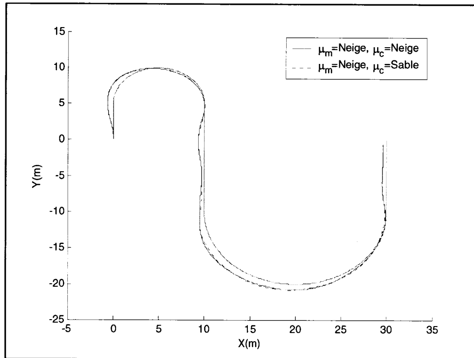
Figure 5.32 : Suivi de chemin avec adhérence du modèle différent de l'adhérence du contrôleur ( \mu_m=\text{Neige} , \mu_c=\text{Sable} )
