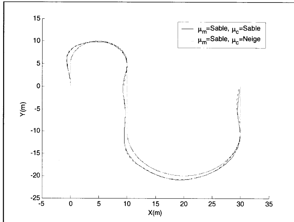
Figure 5.30 : Suivi de chemin avec adhérence du modèle différente de l'adhérence du contrôleur ( \mu_m =Sable, \mu_c =Neige)
