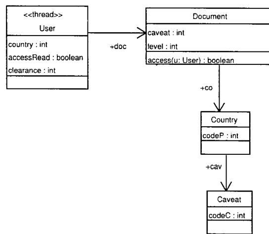
Figure 5.6 Diagramme de classes - Étape 2
