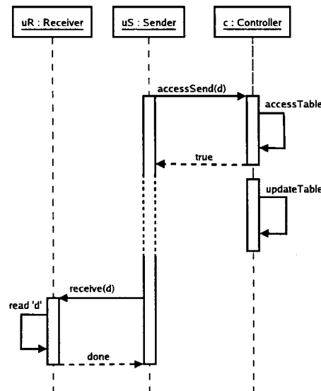
Figure 5.21 Diagramme de séquences - Erreur
