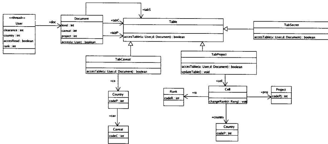
Figure 5.9 Diagramme de classes - Étape 3 et 4
