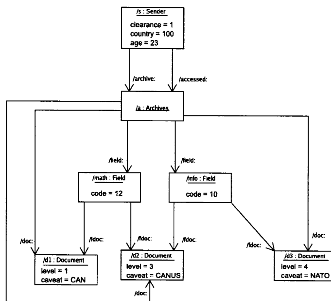
Figure 4.2 Diagramme d'objets - Archives
