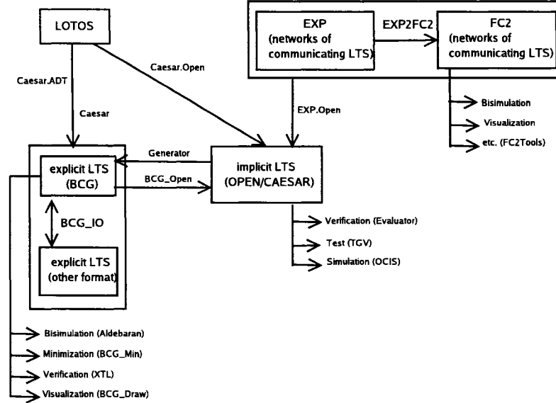
Figure 2.1 Environnement CADP
