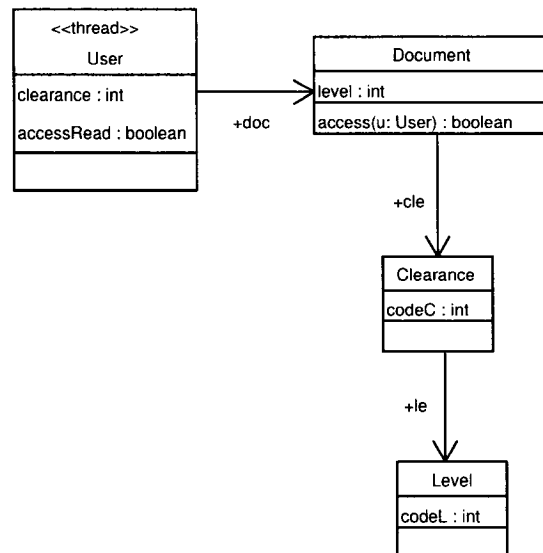
Figure 5.3 Diagramme de classes - Étape 1
