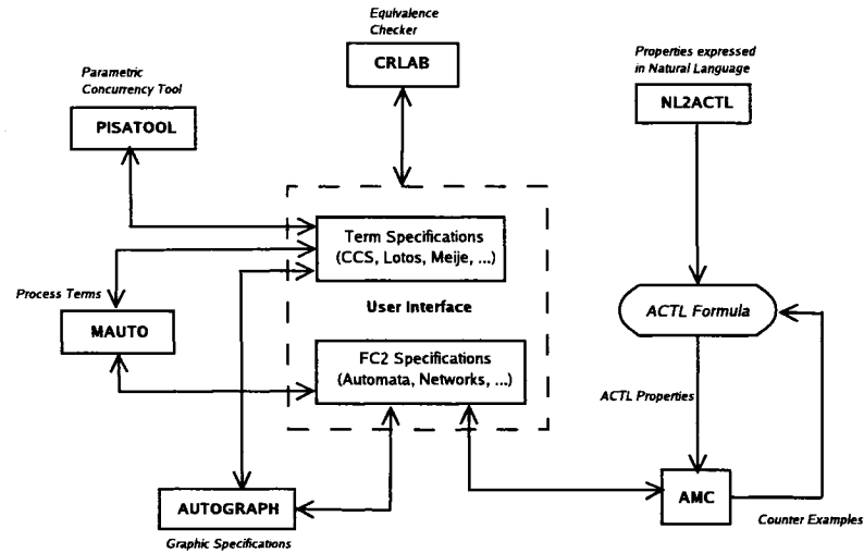
Figure 2.4 Projet JACK
