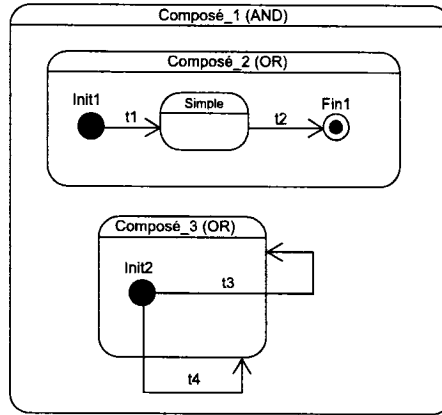
Figure 3.5 Diagramme d'états-transitions (AND)
