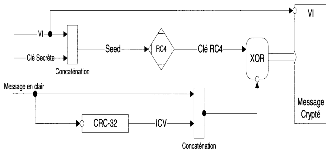
Figure 2.1 Diagramme d'encryption avec WEP
