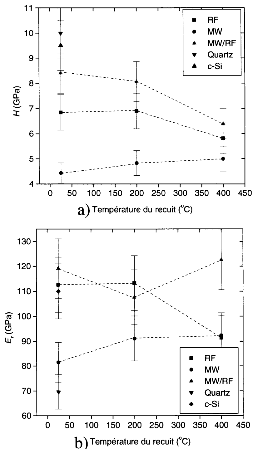
Figure 6.2 : a) Dureté, et b) Module de Young réduit de \text{Nb}_2\text{O}_5 déterminés au nanotriboindenteur ( F_n = 3000 \mu\text{N} , \nu = 200 \mu\text{N/s} )
