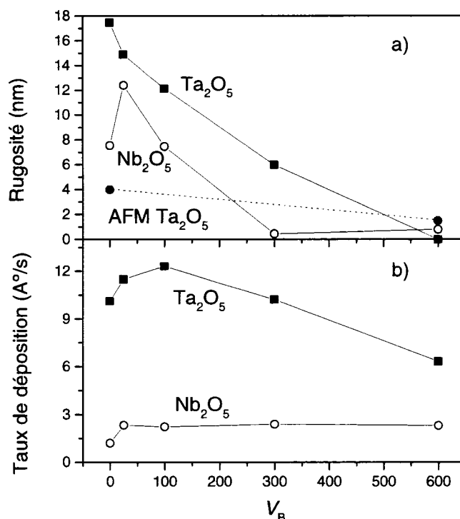
Figure 4.3 : Effet du potentiel d'autopolarisation sur la rugosité (a) et le taux de déposition (b) de couches minces d'oxydes de tantale et de niobium déposées en mode RF et MW/RF. F_{Ar} = 10 sccm, F_{O_2} = 200 sccm, P_{MW} = 500 W.
