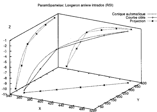
(c) Variation du longeron arriere à l'intrados
