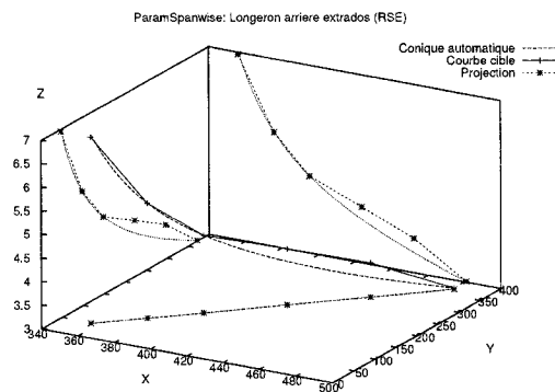
(d) Variation du longeron arriere à l'extrados
