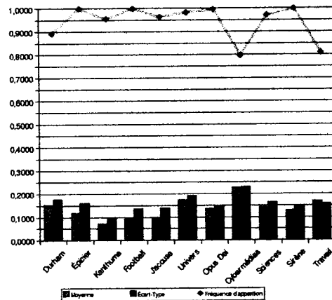
Figure 7.7 Métrique L . Évolution de la cote attribuée à la métrique L, en comparaison à la moyenne et à l'écart-type du poids attribué aux phrases.
