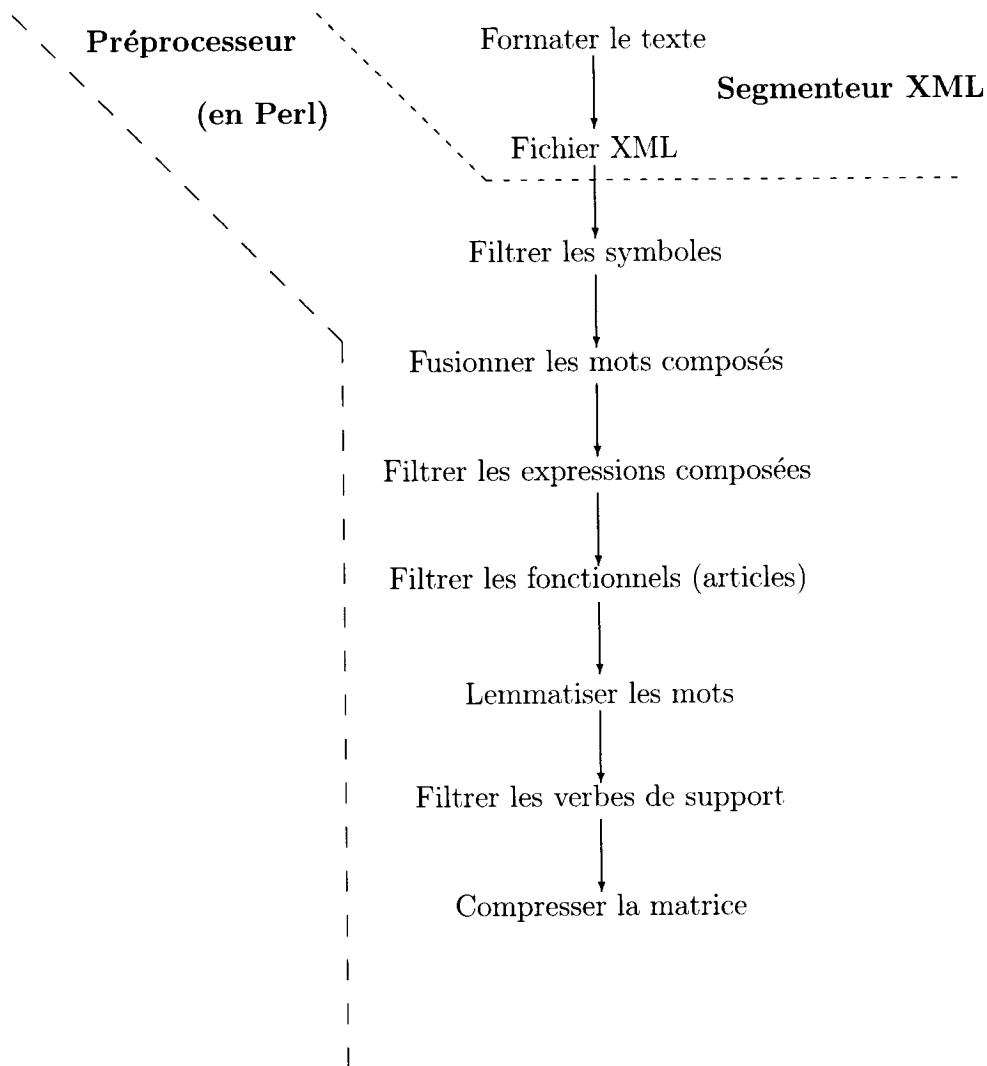
Figure 2.1 Pipeline du pré-traitement de Cortex
