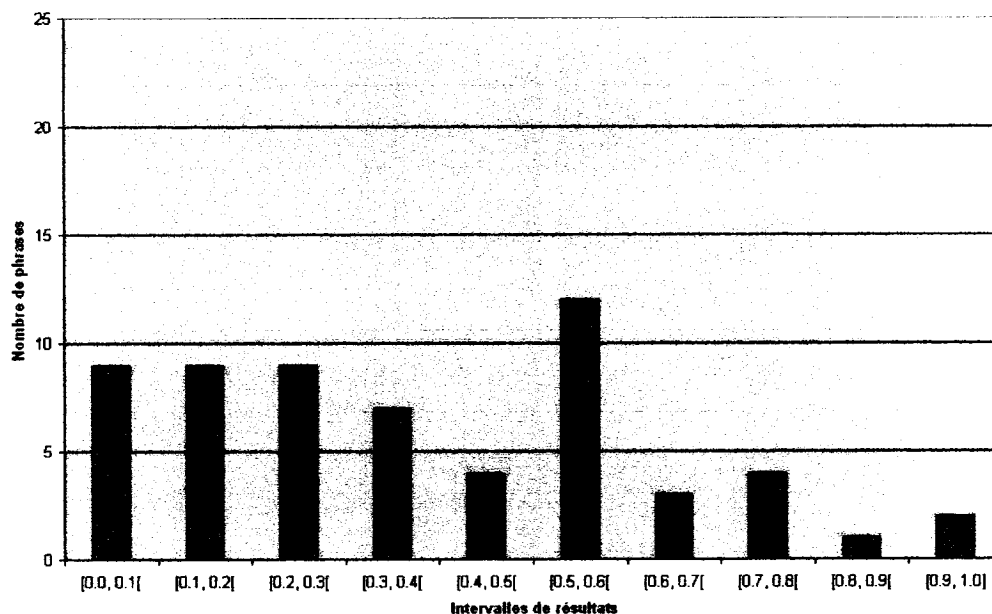
Figure 7.2 Distribution des valeurs normalisées pour la métrique F, pour le texte Cybermédias .
