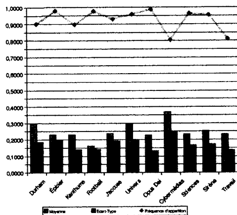
Figure 7.3 Métrique F . Évolution de la cote attribuée à la métrique F, en comparaison à la moyenne et à l'écart-type du poids attribué aux phrases.
