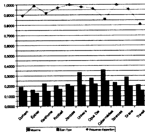
Figure 7.4 Métrique D . Évolution de la cote attribuée à la métrique D, en comparaison à la moyenne et à l'écart-type du poids attribué aux phrases.
