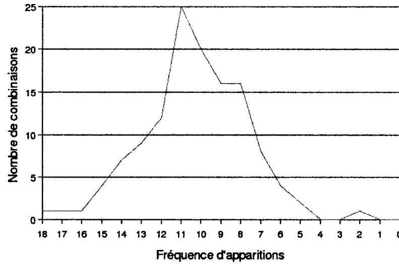
Figure 5.3 Distribution du nombre de combinaisons de métriques selon leur fréquence d'apparition pour n = 20 , T = 309 (synthèse du tableau 5.4).
