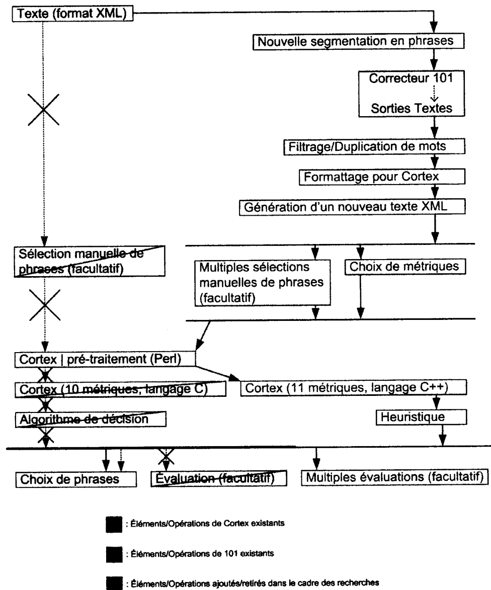
Figure 4.1 Figure illustrant les éléments déjà existants de Cortex (en noir) et du Correcteur 101 (en bleu), ainsi que les éléments/opérations ajoutés aux logiciels afin de réaliser les tests du présent mémoire (en rouge).
