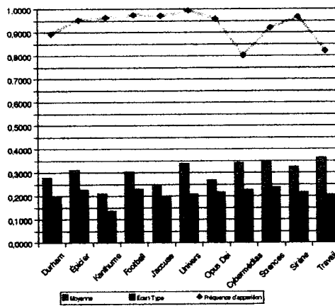
Figure 7.6 Métrique T . Évolution de la cote attribuée à la métrique T, en comparaison à la moyenne et à l'écart-type du poids attribué aux phrases.
