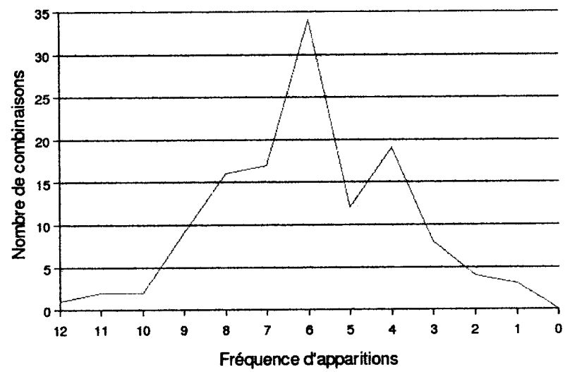
Figure 5.2 Distribution du nombre de combinaisons de métriques selon leur fréquence d'apparition pour n = 10 , T = 757 (synthèse du tableau 5.3).
