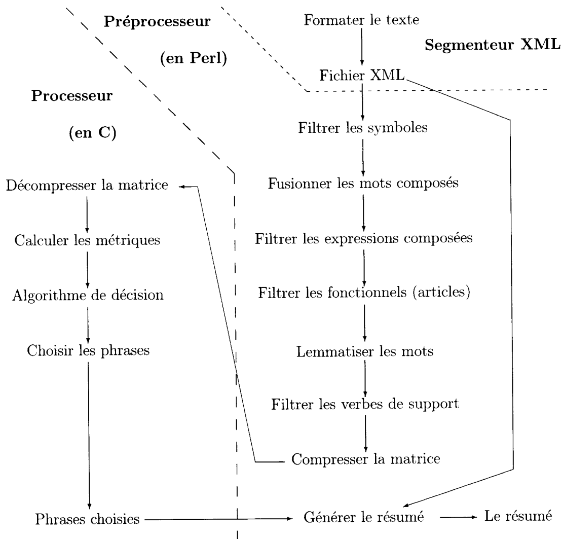
Figure 2.2 Pipeline du traitement complet de Cortex
