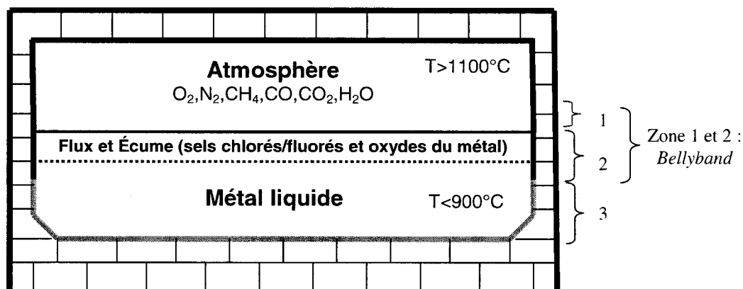
Figure 1-1 : Modélisation d'un four de traitement de l'aluminium
