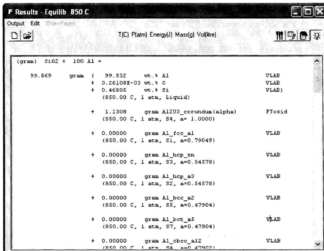
Figure 1-4c : Résultat du calcul suite à la minimisation de l'énergie de Gibbs obtenu dans le logiciel FactSage
