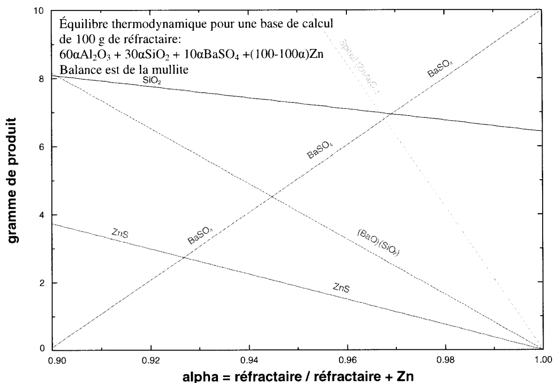
Figure 6-7 : Calcul thermodynamique des produits formés lorsque du Zn réagit avec un excès de réfractaire contenant du BaSO_4 , calculé à 850^\circ C et P_{totale}=1atm
