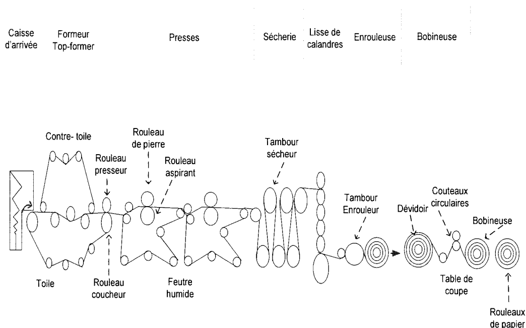
Machine à papier top flyte "B6 et B7"
