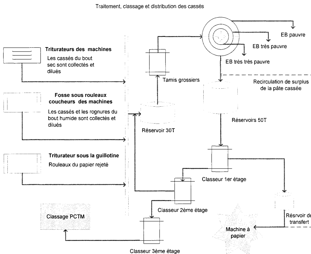
Figure 4-6 Procédé de traitement, de classement et de distribution des cassés « Belgo ».
