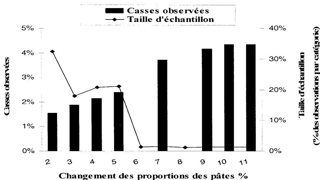
Figure 4-12 Probabilités de casses possiblement dues à la variabilité dans la CA B9. par rapport à l'amplitude des changements des proportions des pâtes.
