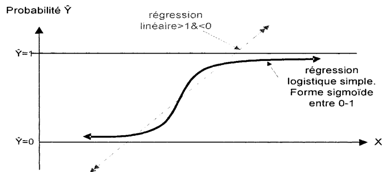
Figure 2-6 Comparaison entre le modèle de régression logistique et le modèle de régression linéaire.
