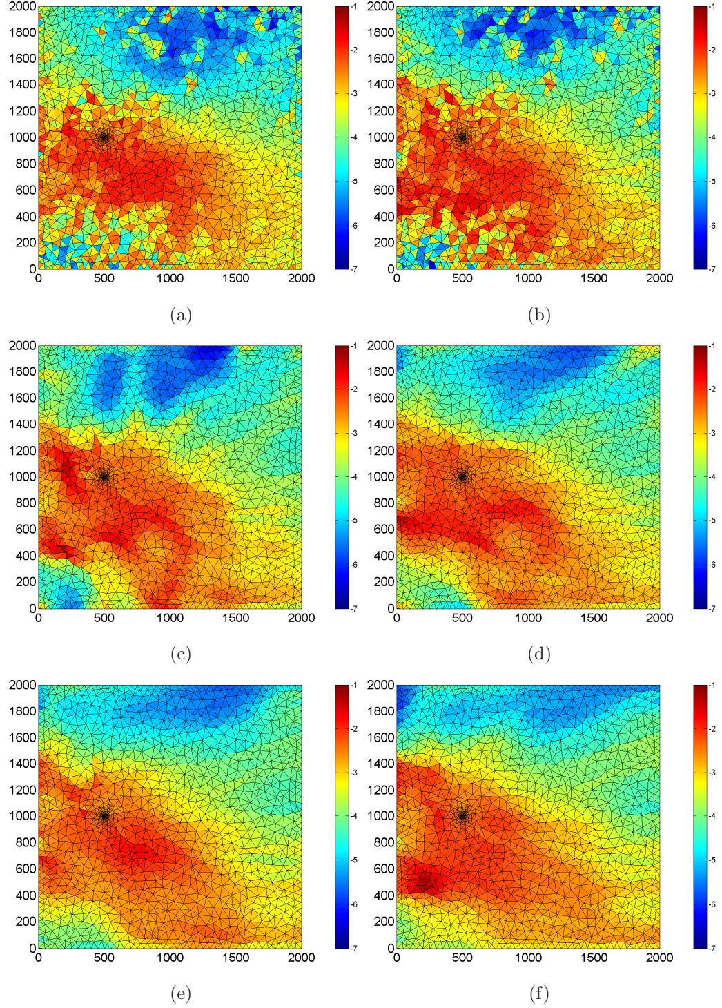
Figure 6.2: Champs de T obtenus pour les scénarios piézométriques 6 à 10 réalisés avec le germe 96 ( \log_{10}(m^2/s) ). (a) Champ de \log_{10}T de référence, (b) à (f) champs de \log_{10}T obtenus pour les scénarios piézométriques 6 à 10.
