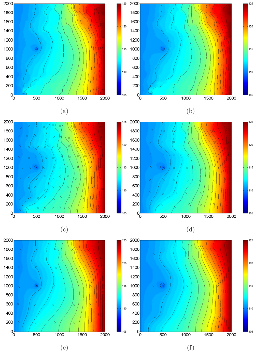
Figure 6.7: Champs de charges obtenus après calibration pour les scénarios piézométriques 6 à 10 avec le germe 96 (m) à t = 0.12d .(a) Champ de référence,(b) à (f) champs obtenus pour les scénarios piézométriques 6 à 1.
