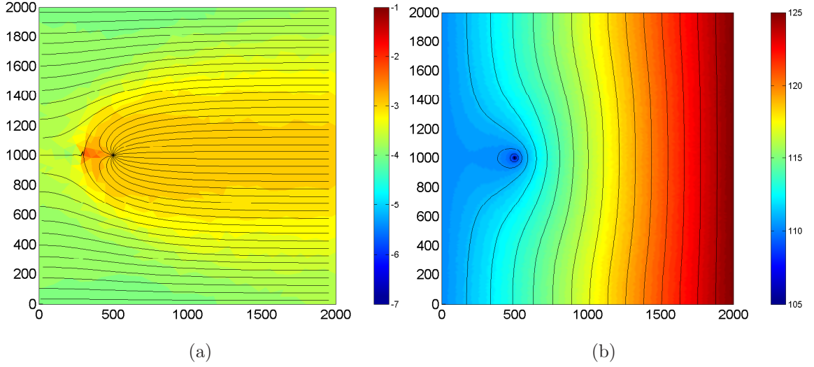
Figure 4.12: Exemple 10 réalisé par la méthode de l'estimation successive des flux en régime transitoire avec un germe de T uniforme de 10^{-4} m^2/s . (a) champ de \log_{10} T calibré et (b) charges ajustées ( m ).
