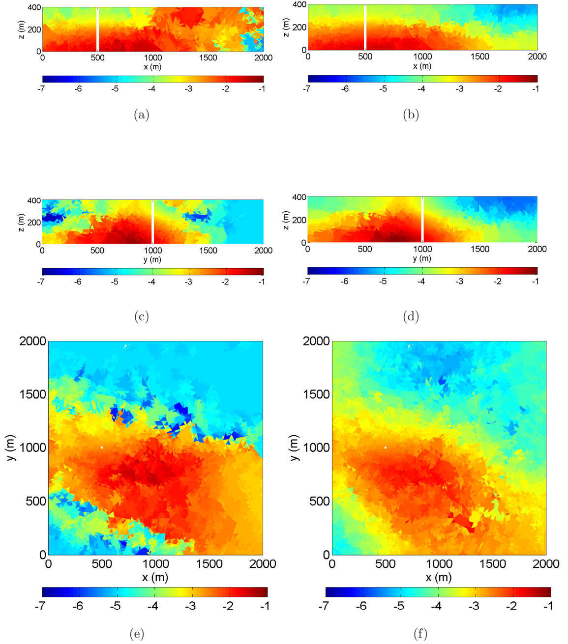
Figure 4.15: Inversion tridimensionnelle en régime transitoire. Coupes du champ de conductivités hydrauliques ( \log_{10}(m/s) ) pour (a) champ calibré ( y=1000\text{m} ), (b) champ de référence ( y=1000\text{m} ), (c) champ calibré ( x=500\text{m} ), (d) champ de référence ( x=500\text{m} ), (e) champ calibré ( z=200\text{m} ), (f) champ de référence ( z=200\text{m} ).
