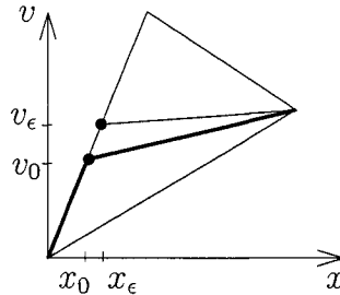
Figure 5.7 Proposition 5.3, cas 5 : l'erreur en x_0 et x_\epsilon .
