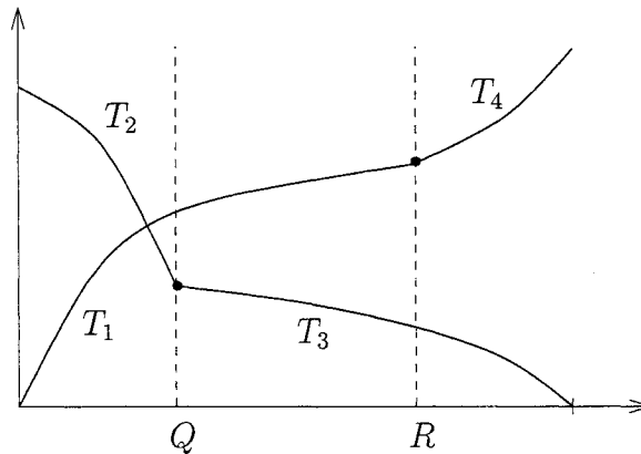
Figure 4.13 La fonction \theta(x) .
