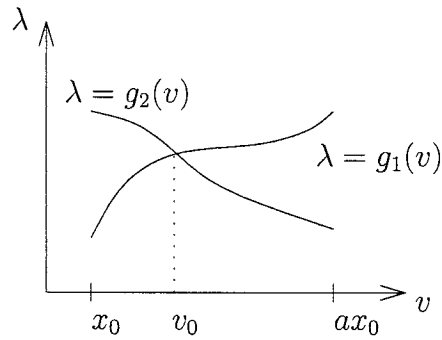
Figure 5.3 Solution aux équations (5.8)
